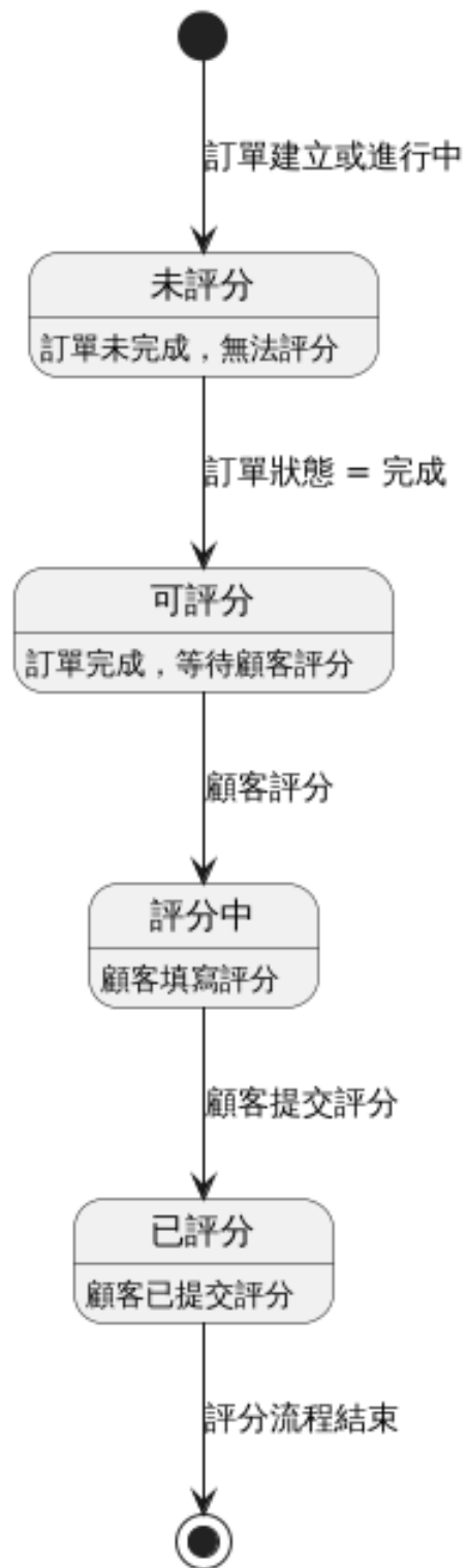
圖 7-4-4 訂單評分狀態機
