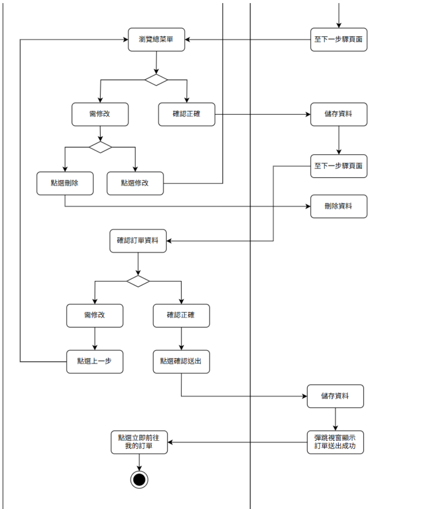
圖 5-3-7 活動圖之顧客發送訂單
