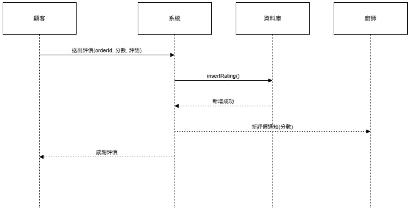
圖 6-1-11 循序圖之顧客給廚師評價
