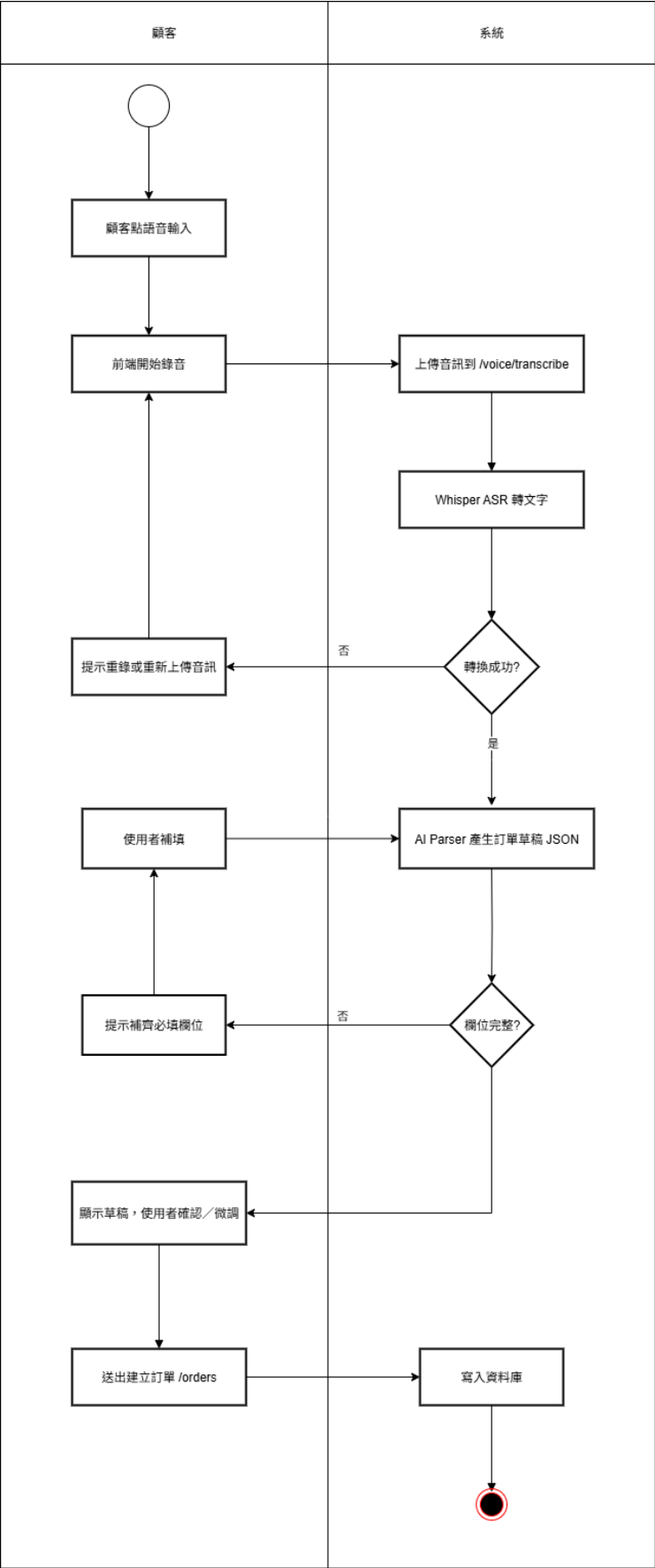
圖 5-3-17 活動圖之 AI 語音輸入
