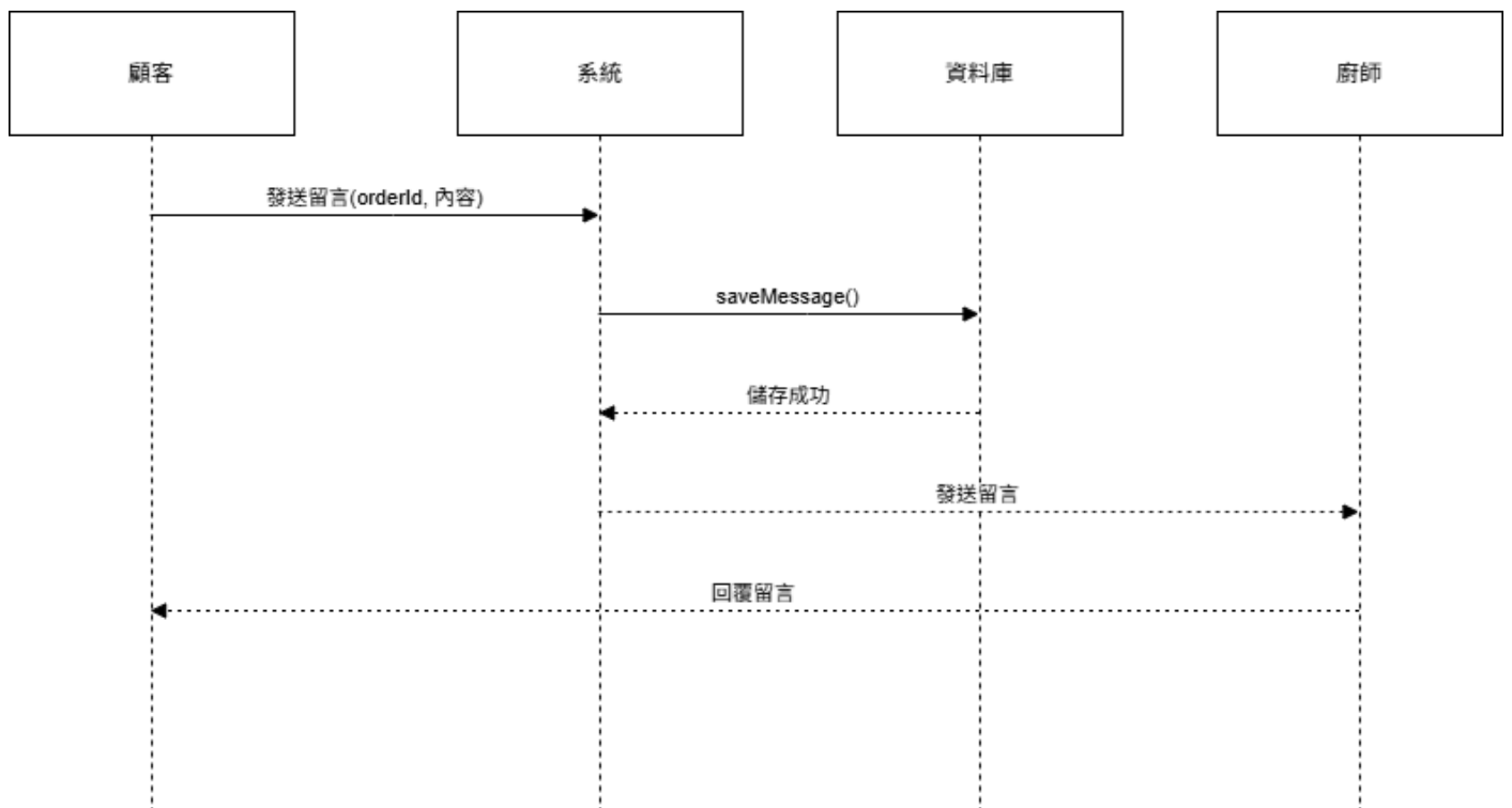
圖 6-1-10 循序圖之顧客端訂單留言板
