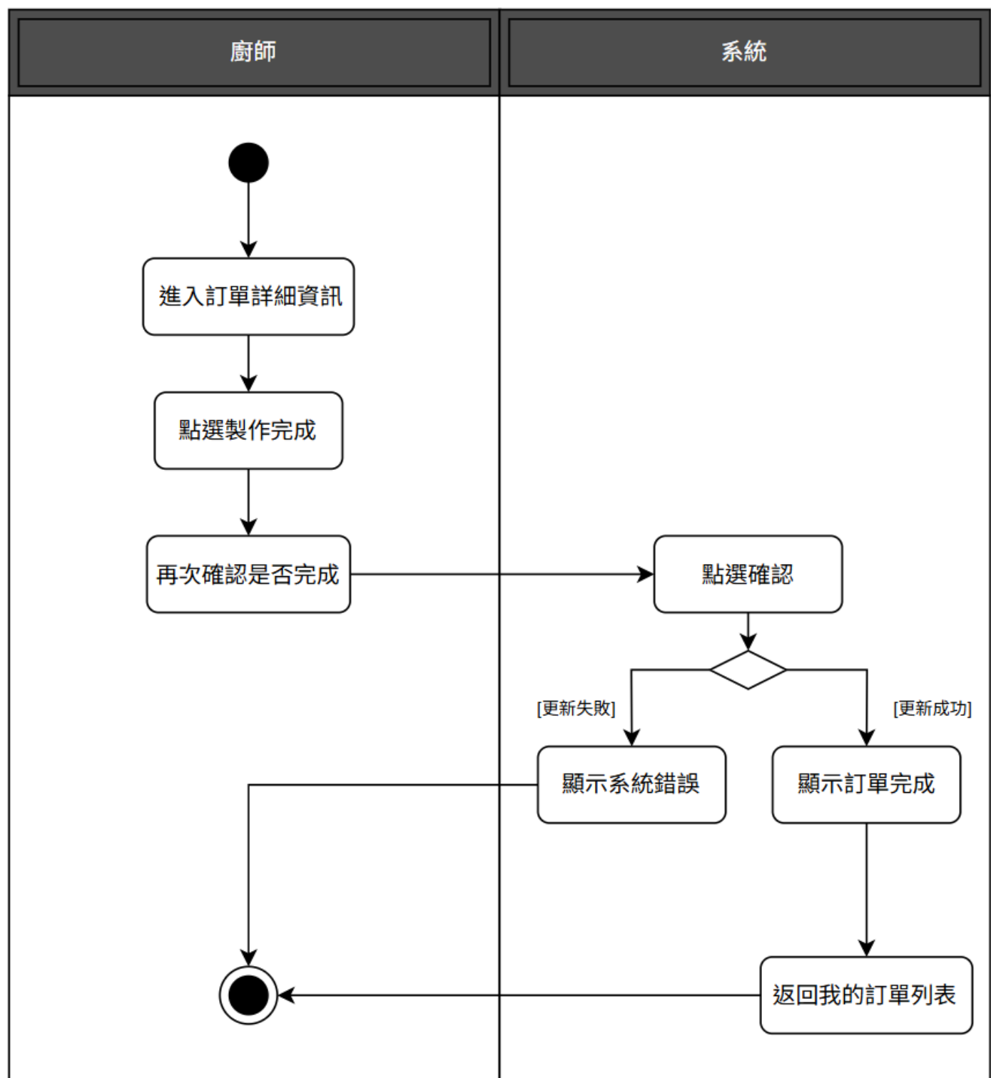
圖 5-3-15 活動圖之廚師更新訂單狀態
