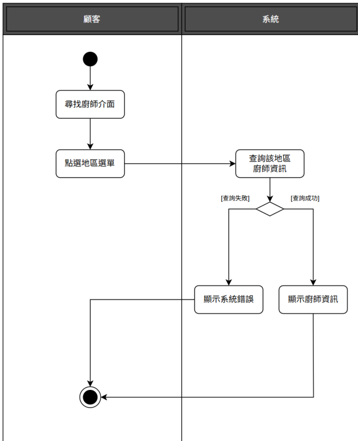
圖 5-3-5 活動圖之顧客查詢廚師
