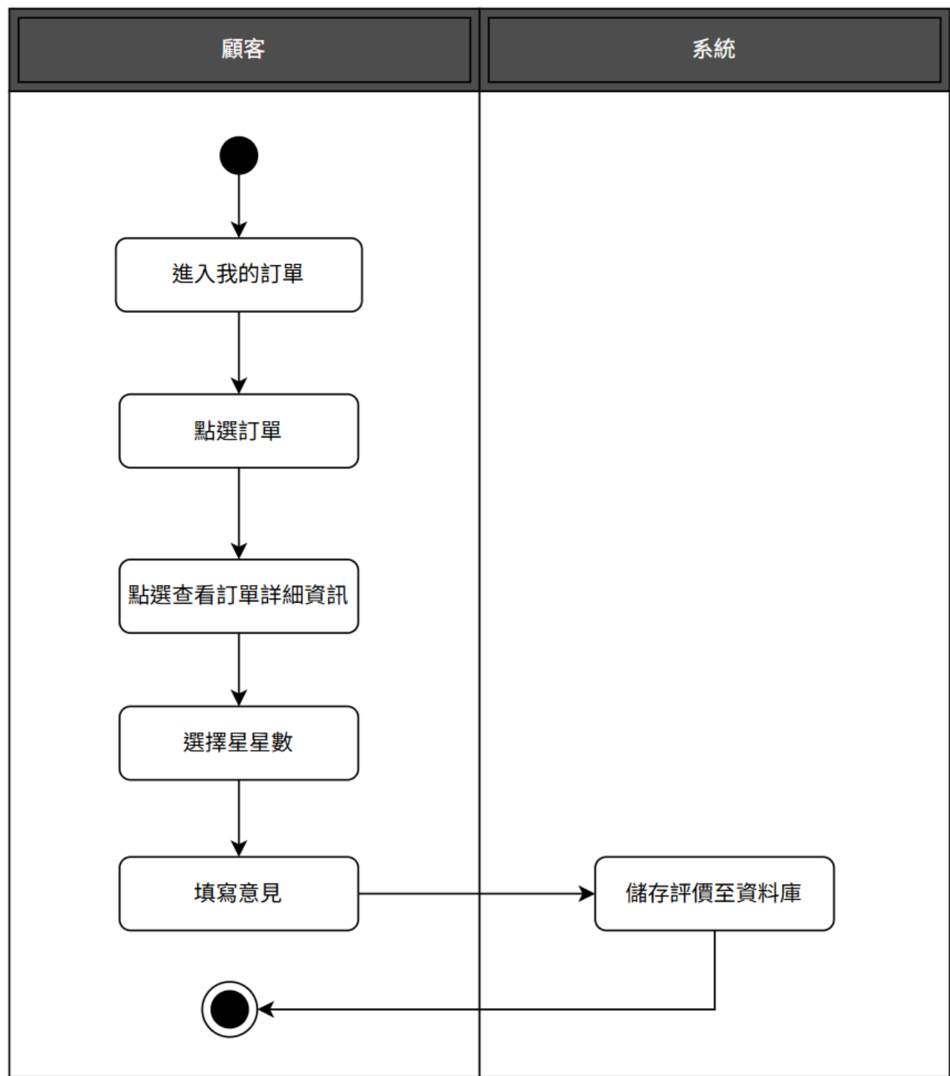
圖 5-3-11 活動圖之顧客給予廚師評價
