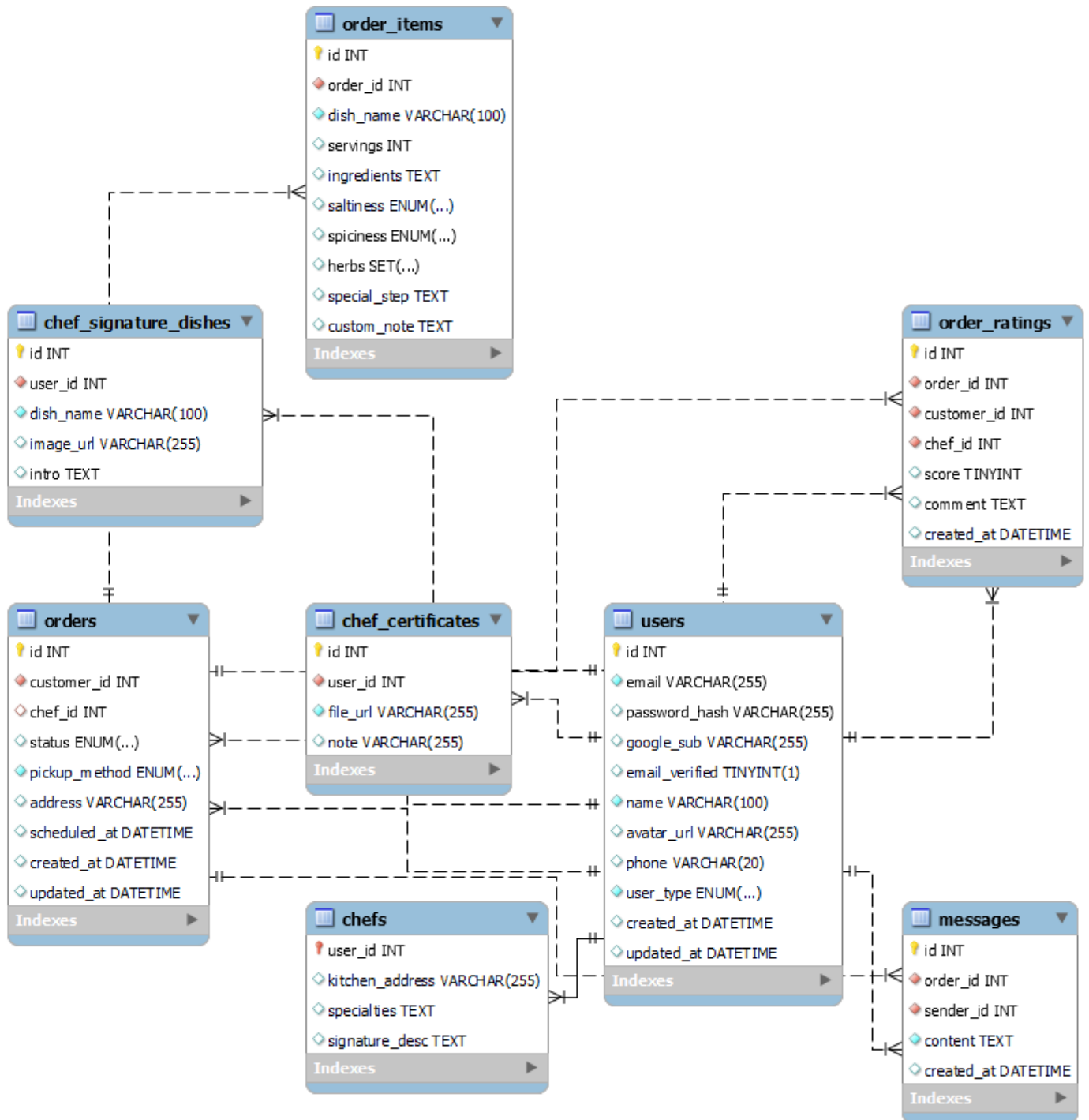
圖 8-1-1 資料庫關聯表
