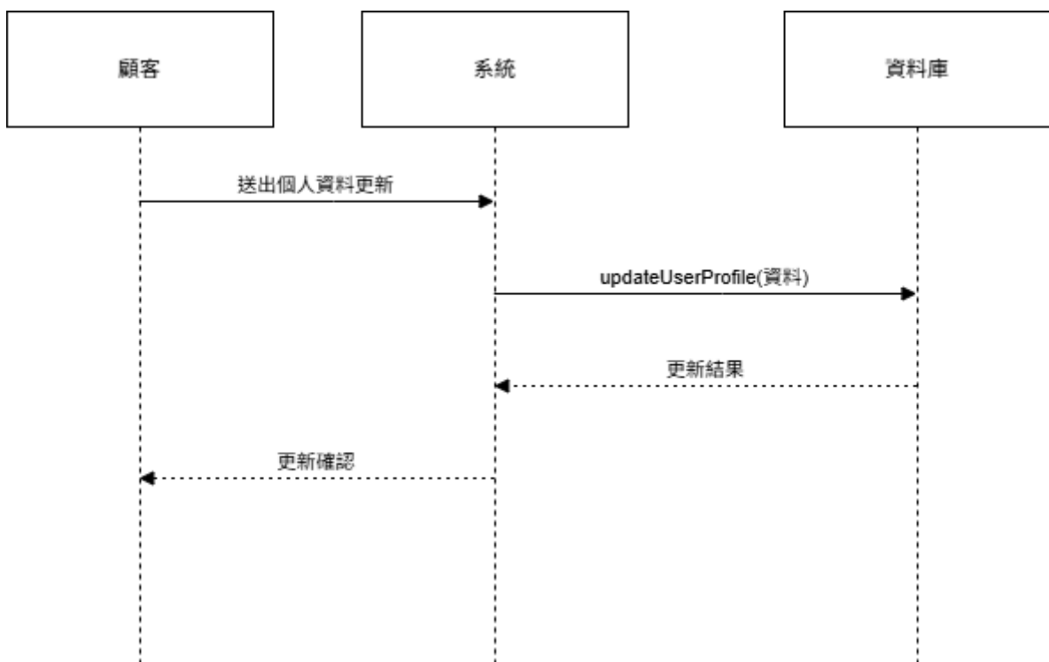
圖 6-1-3 循序圖之顧客編輯個人資料
