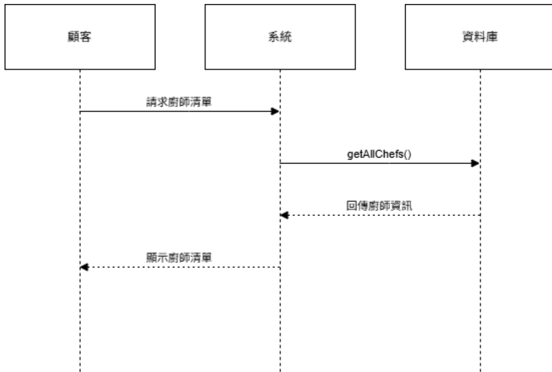
圖 6-1-4 循序圖之顧客瀏覽所有廚師
