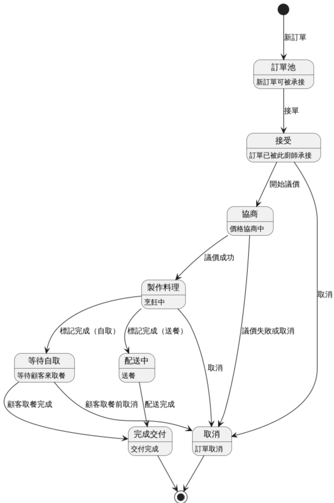
圖 7-4-3 廚師接單狀態機
