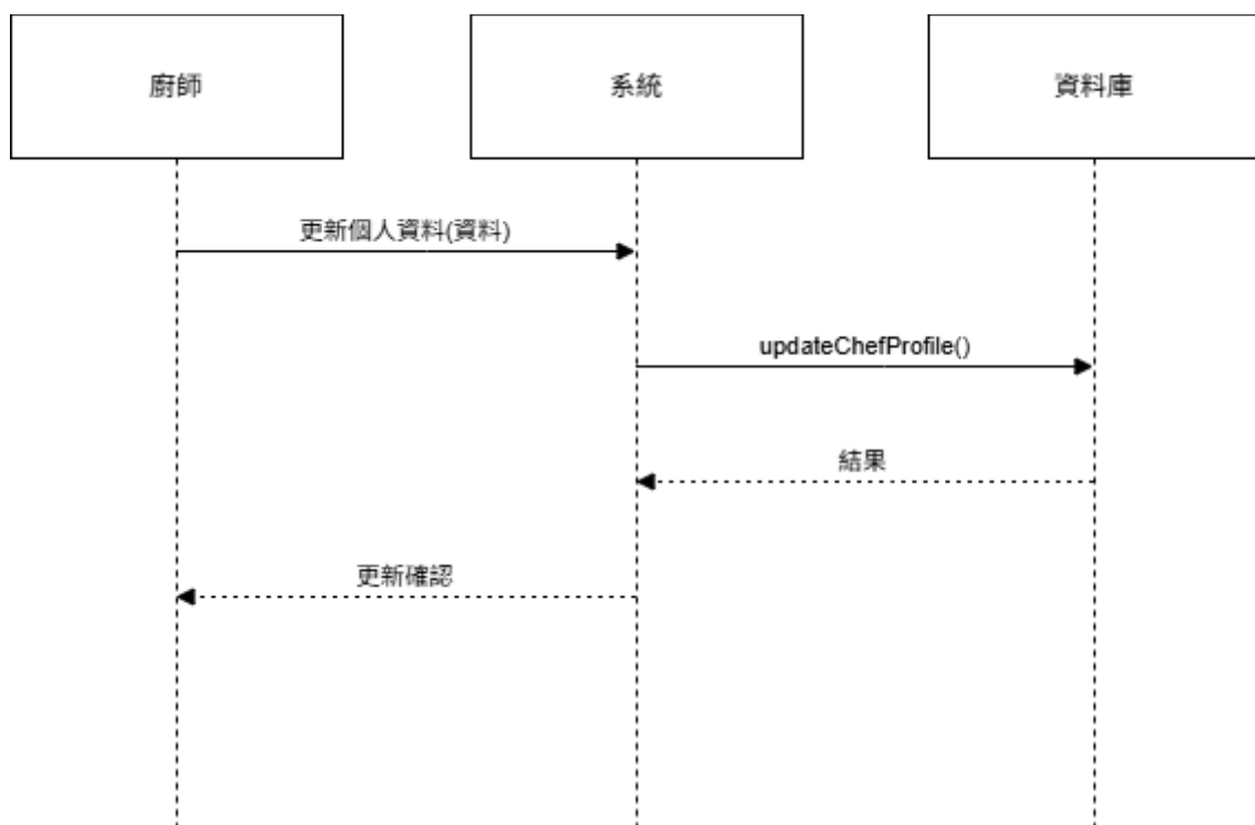
圖 6-1-12 循序圖之廚師編輯個人資料
