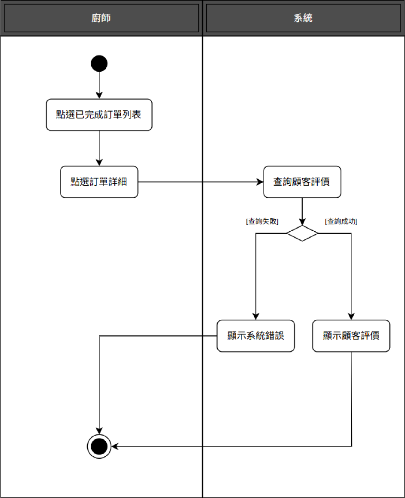
圖 5-3-16 活動圖之廚師查看評價
