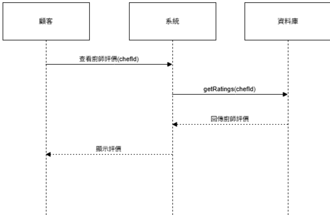
圖 6-1-6 循序圖之顧客瀏覽廚師評價
