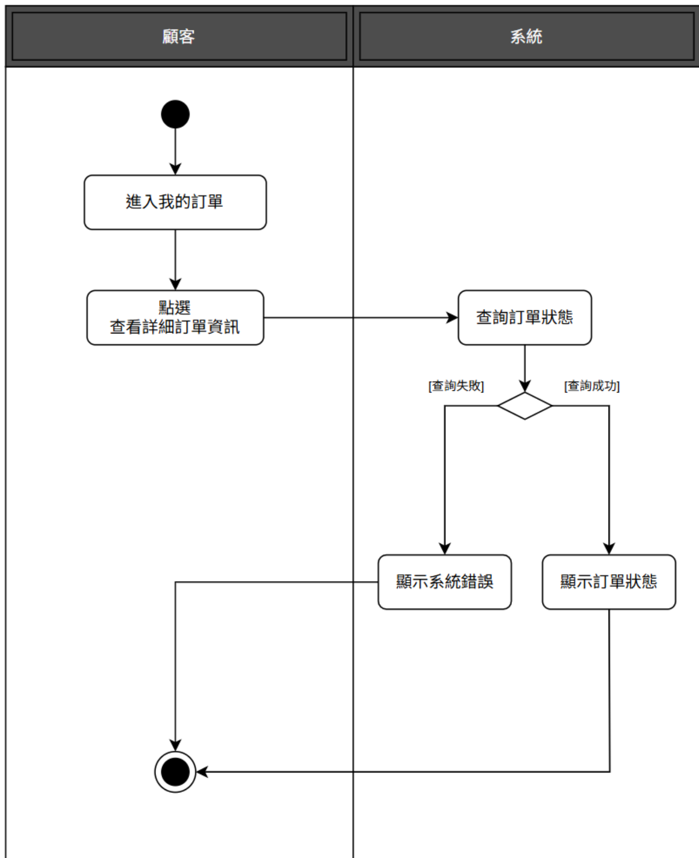
圖 5-3-9 活動圖之查看訂單狀態-顧客端
