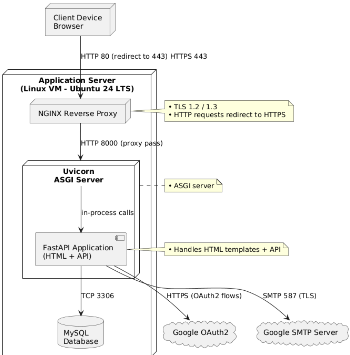
圖 7-1 部署圖
