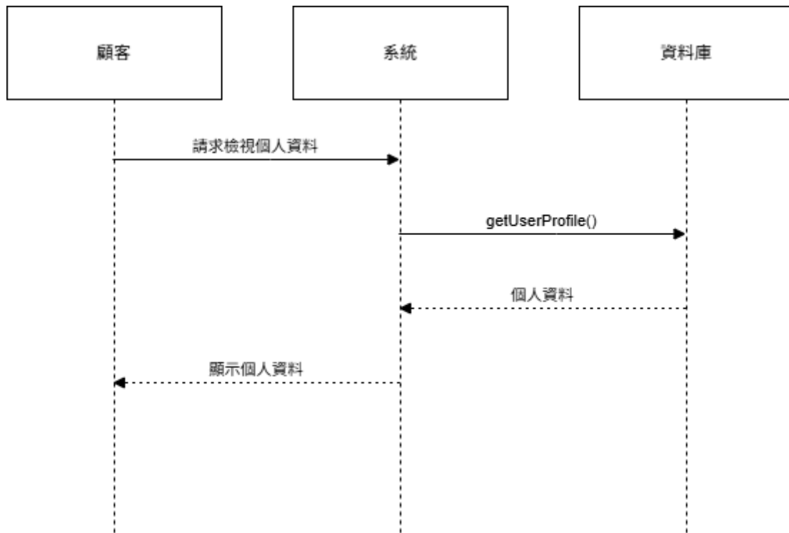
圖 6-1-2 循序圖之顧客檢視個人資料
