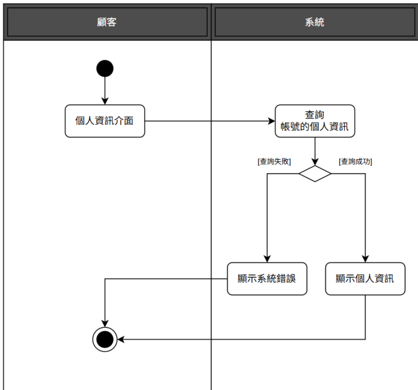
圖 5-3-2 活動圖之檢視個人資料-顧客
