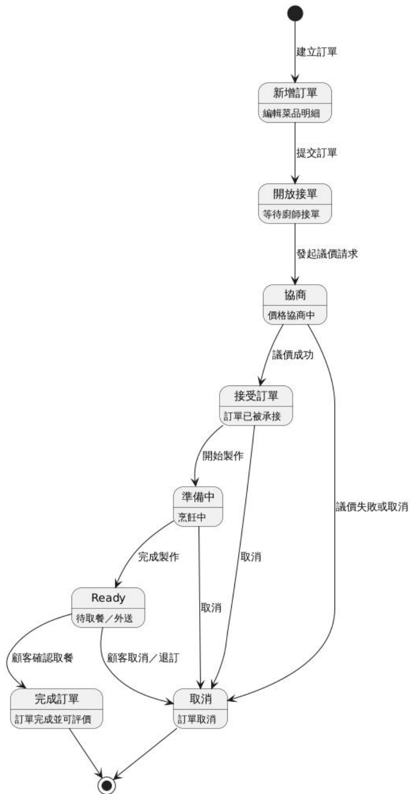
圖 7-4-2 顧客訂單狀態機
