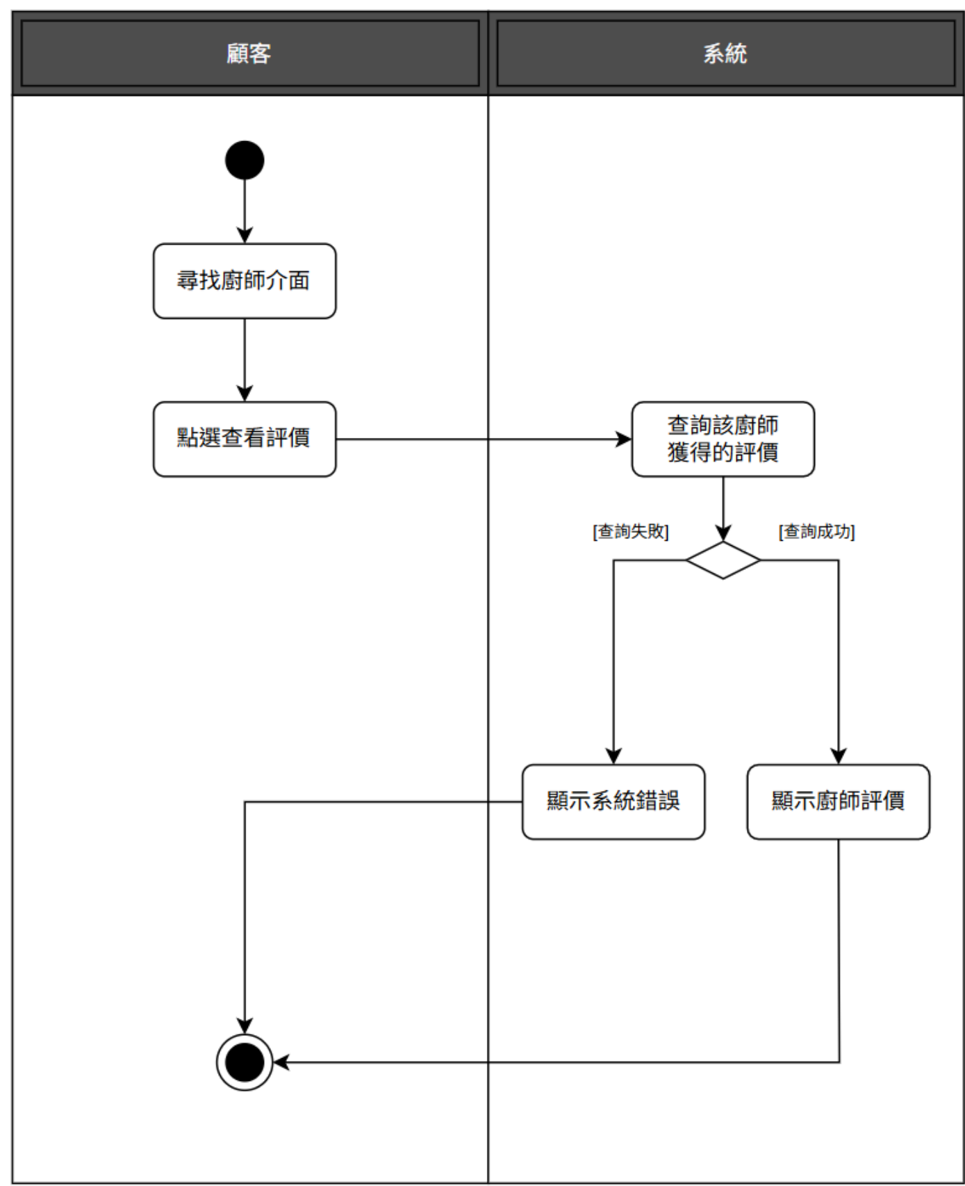
圖 5-3-6 活動圖之顧客瀏覽廚師評價
