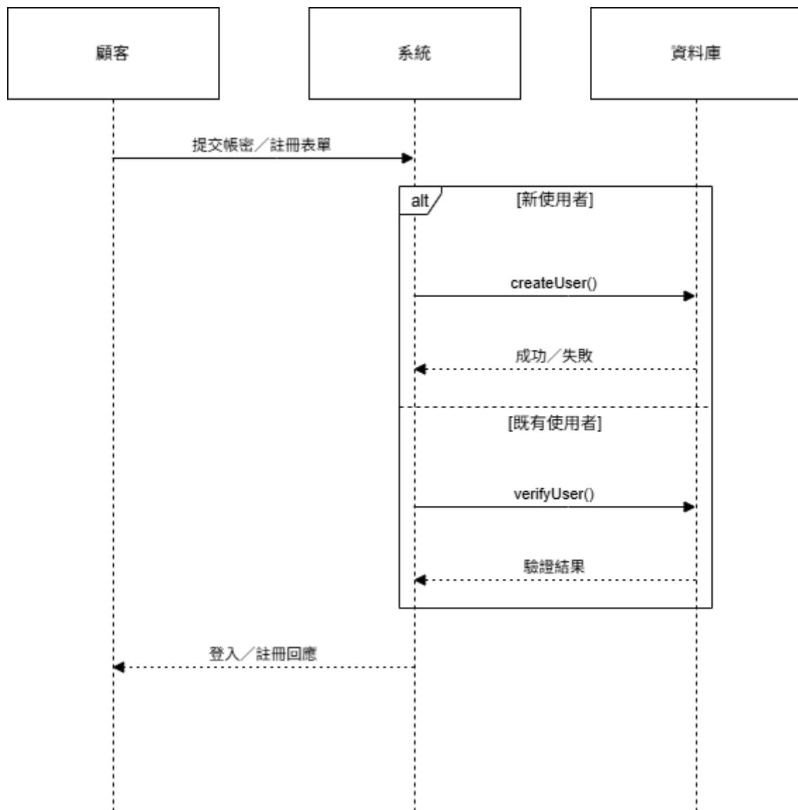
圖 6-1-1 循序圖之顧客註冊登入
