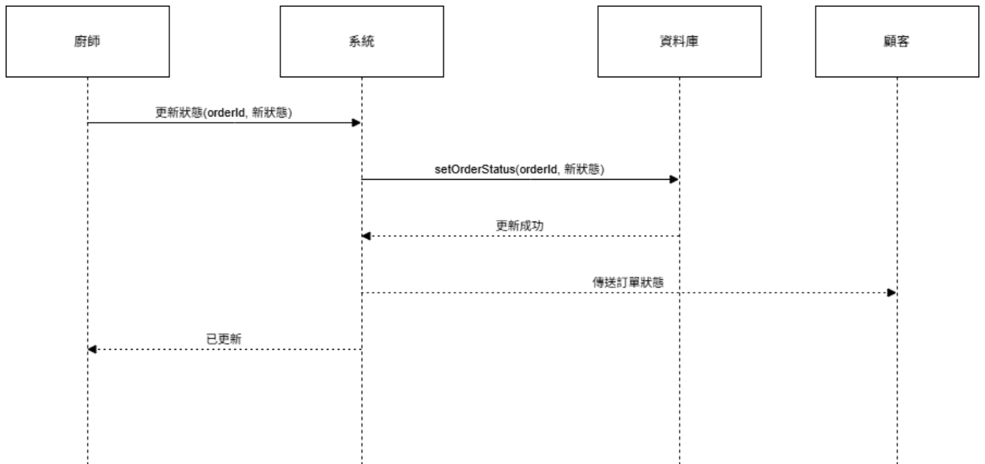
圖 6-1-15 循序圖之廚師更新訂單狀態
