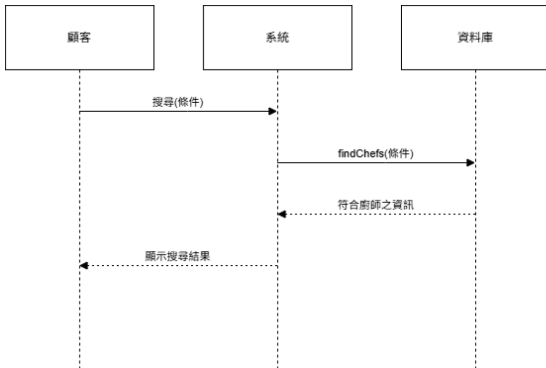
圖 6-1-5 循序圖之顧客查詢廚師
