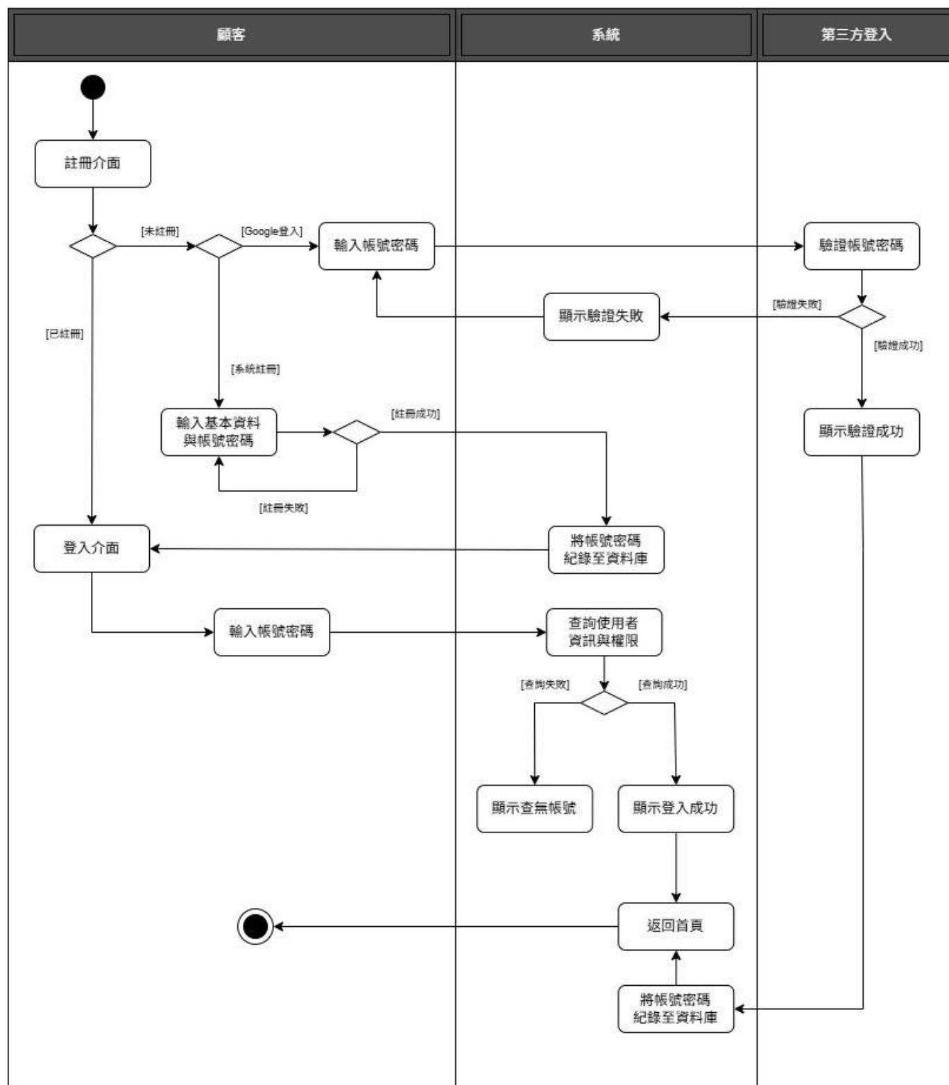
圖 5-3-1 活動圖之註冊登入-顧客
