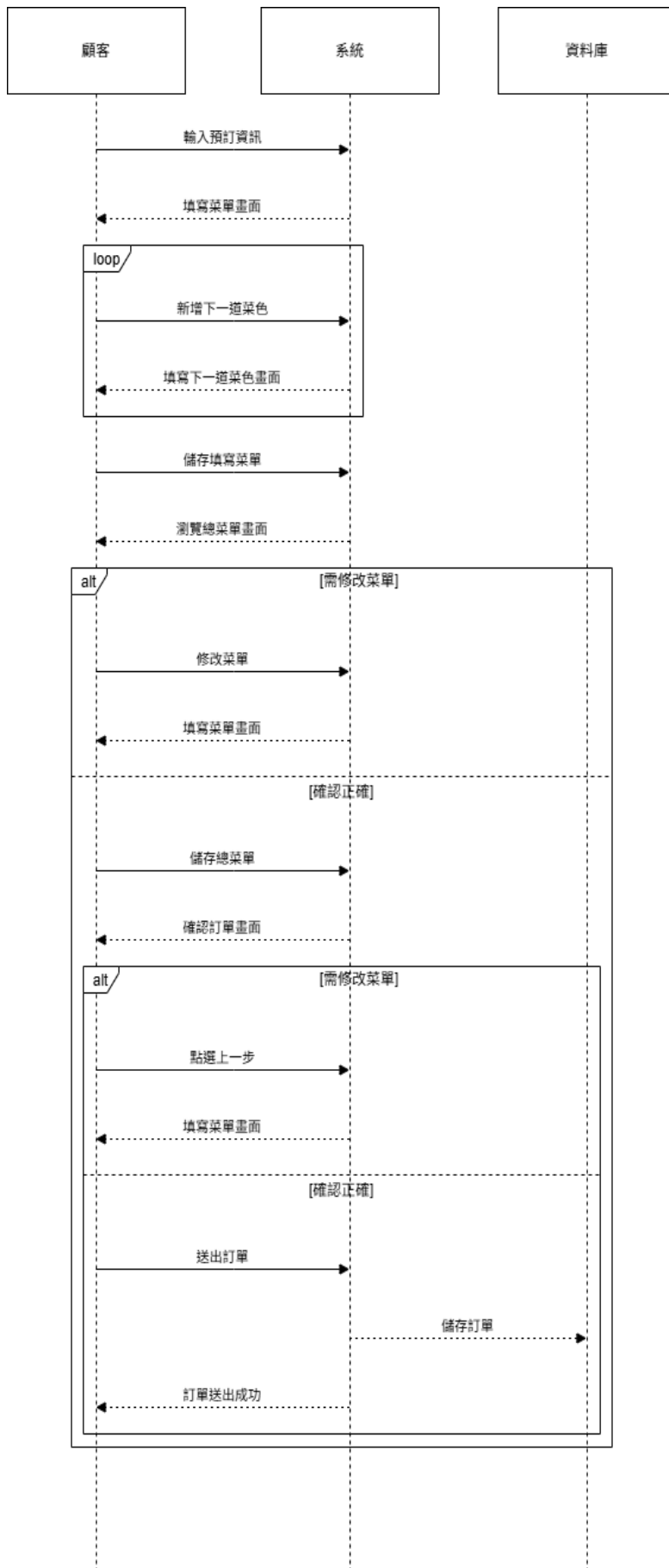
圖 6-1-7 循序圖之顧客發送訂單
