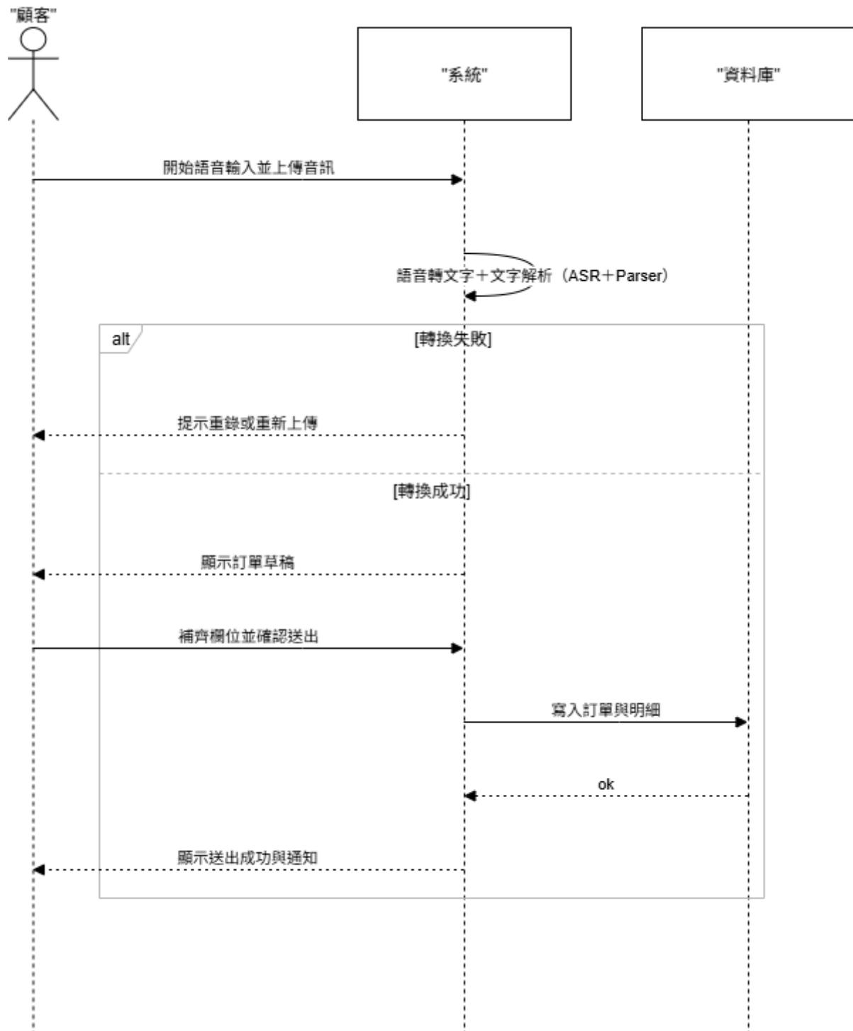
圖 6-1-17 循序圖之 AI 語音輸入
