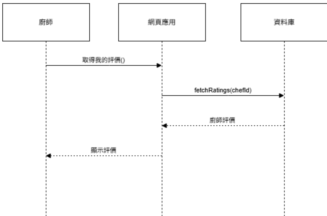
圖 6-1-16 循序圖之廚師查看評價
