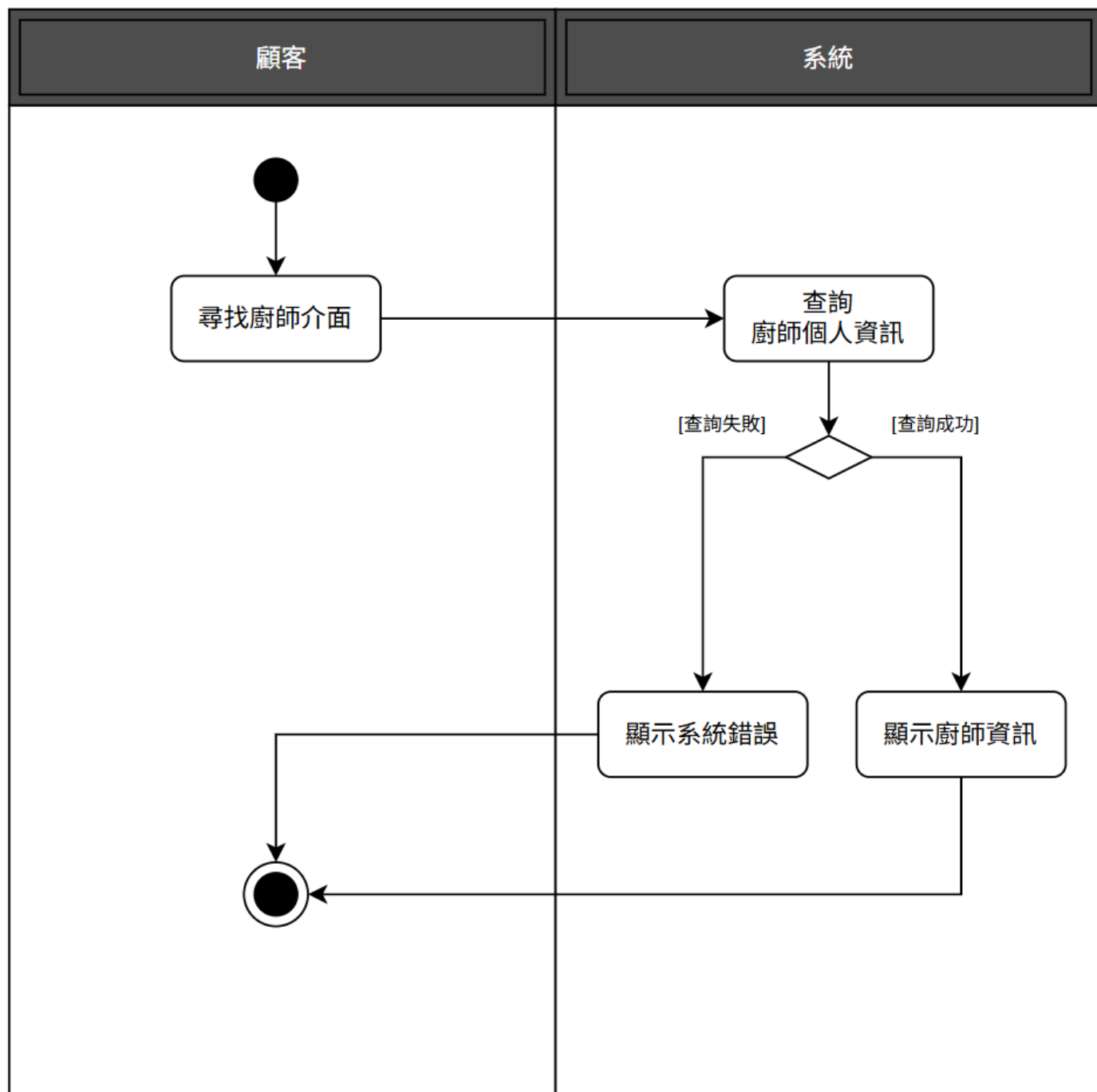
圖 5-3-4 活動圖之顧客瀏覽所有廚師
