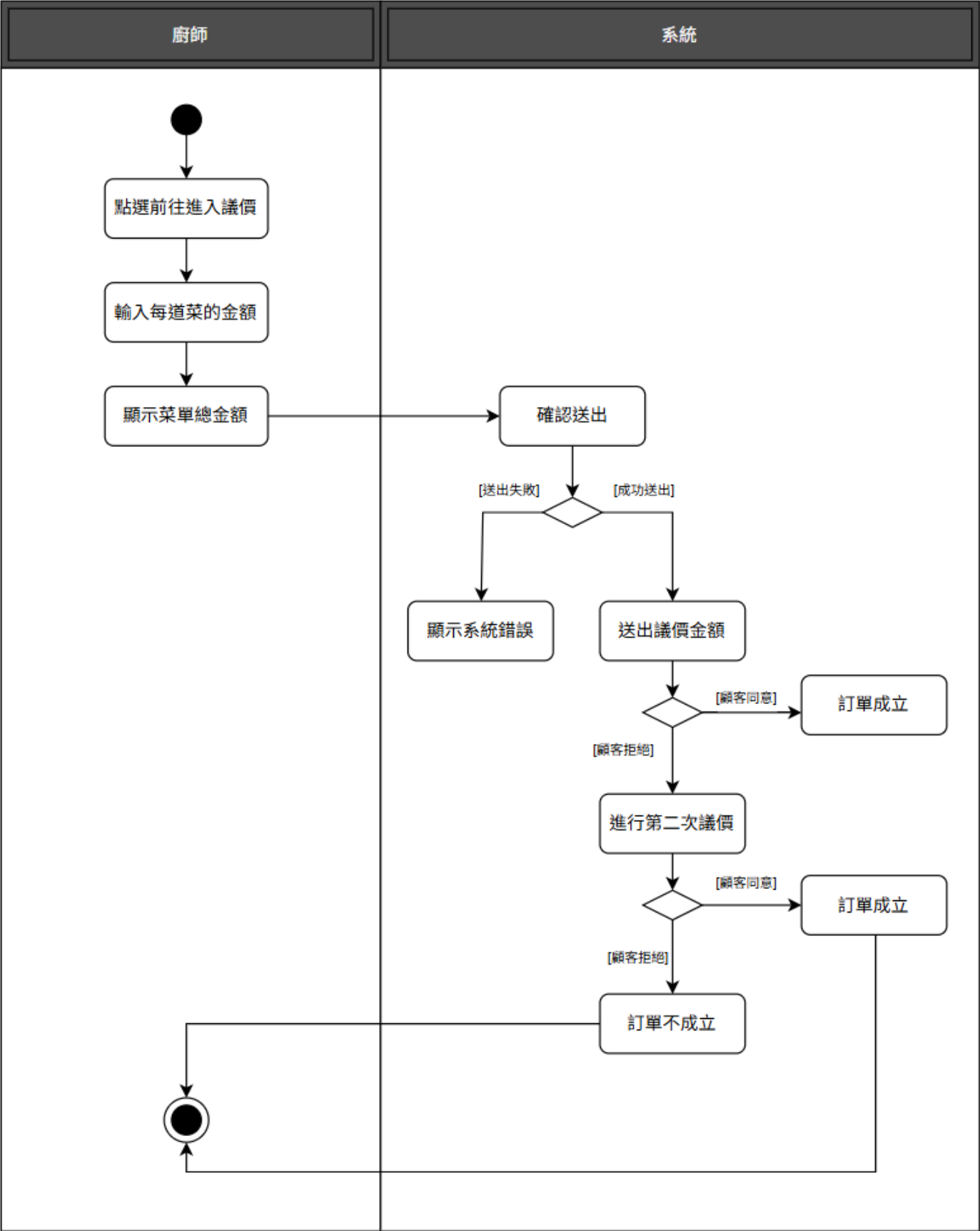
圖 5-3-14 活動圖之議價-廚師端
