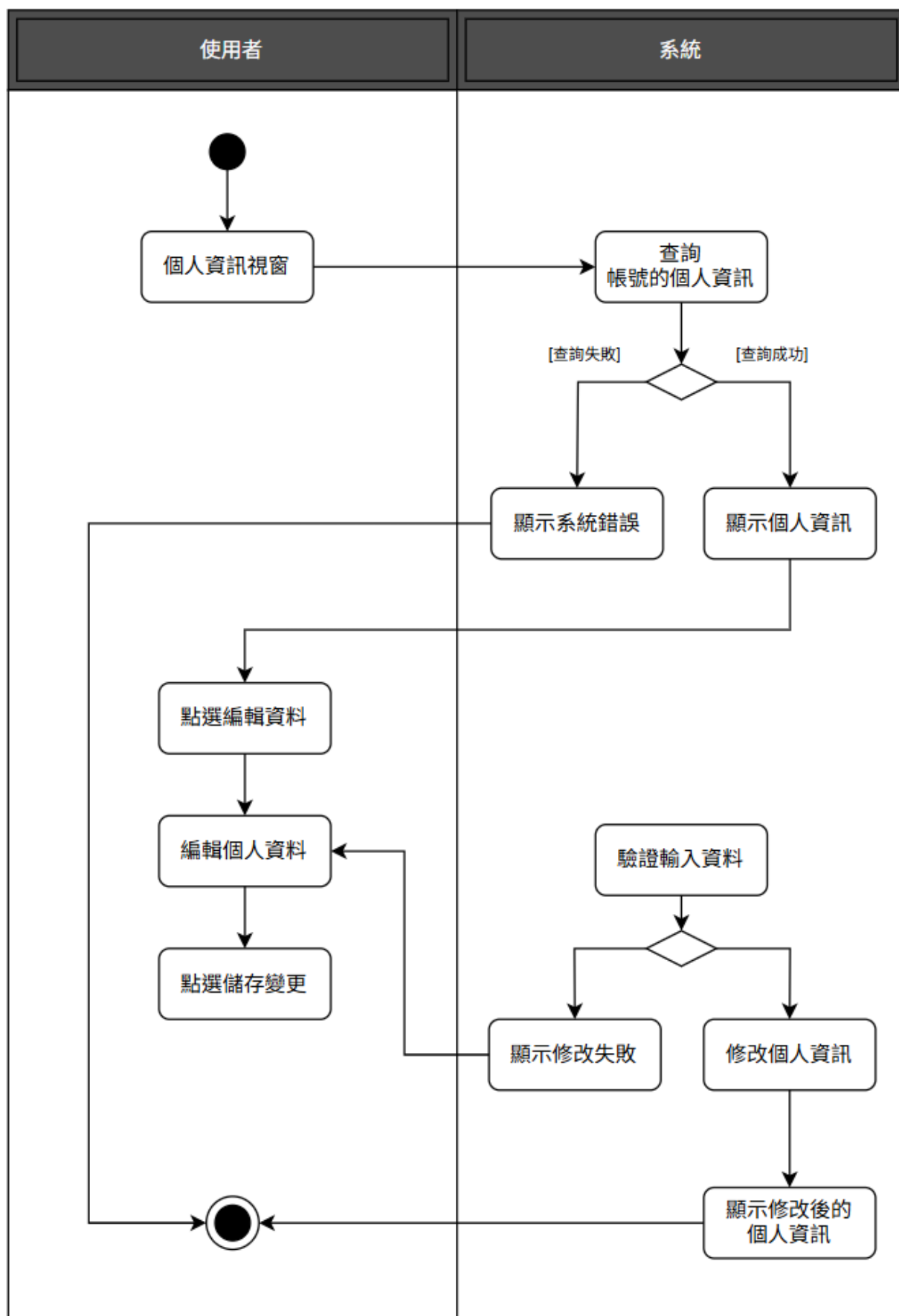
圖 5-3-3 活動圖之編輯個人資料-顧客
