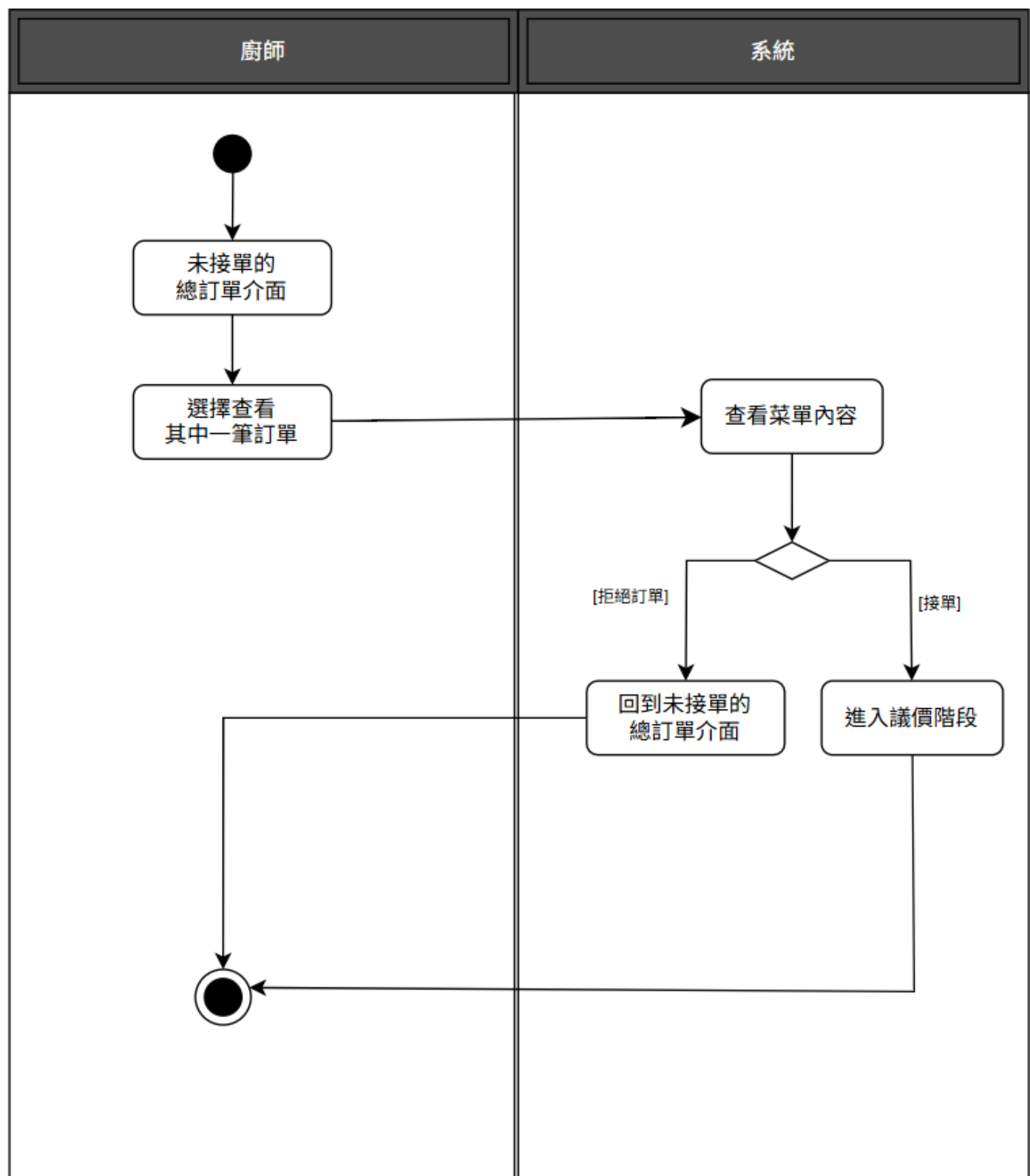
圖 5-3-13 活動圖之廚師接單
