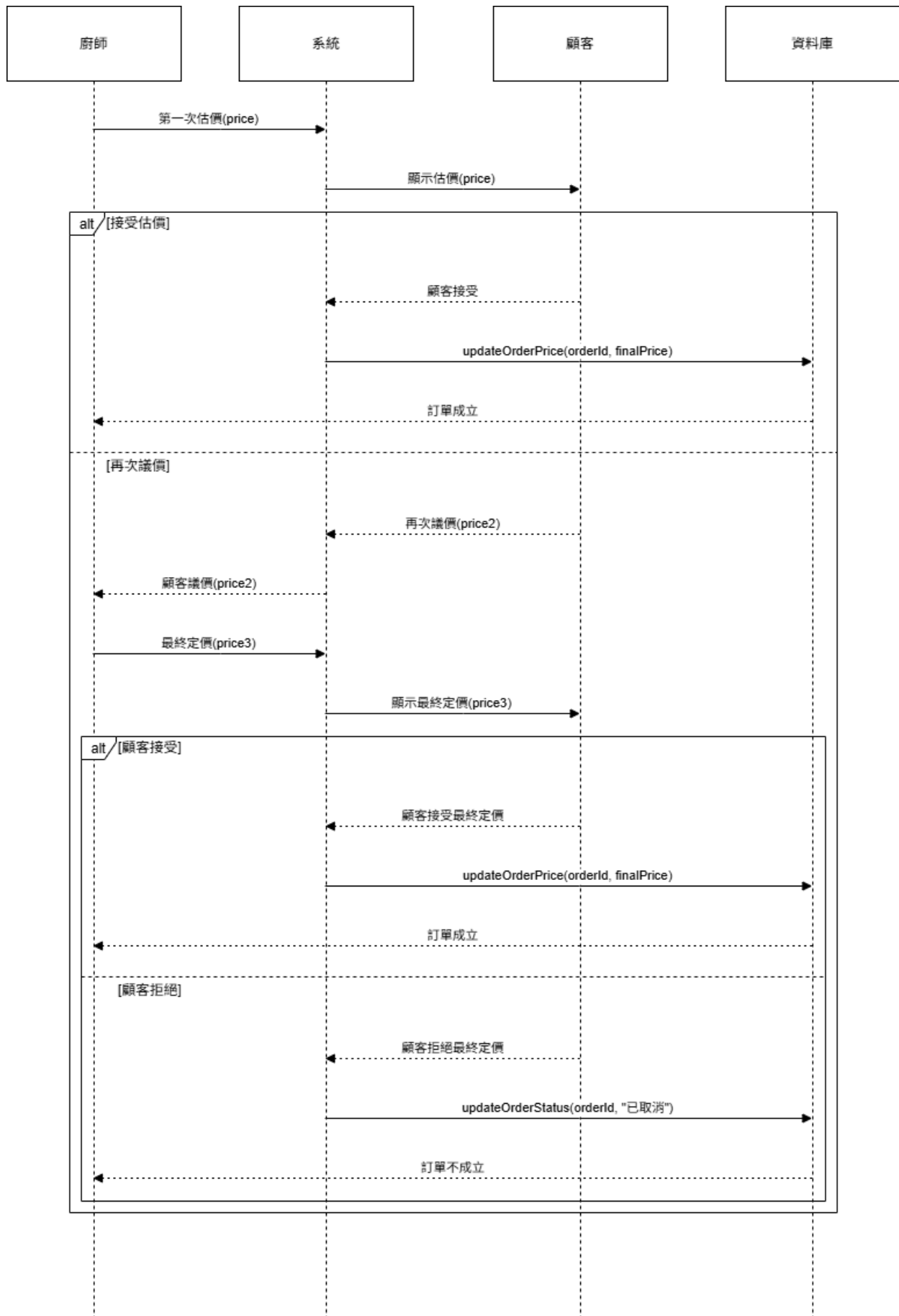
圖 6-1-14 循序圖之廚師端議價
