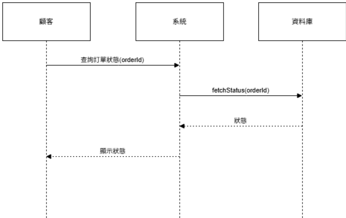
圖 6-1-9 循序圖之顧客查看訂單狀態
