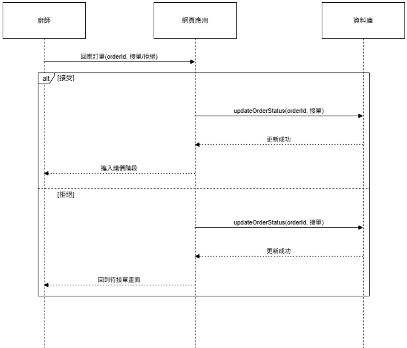
圖 6-1-13 循序圖之廚師接受/拒絕訂單
