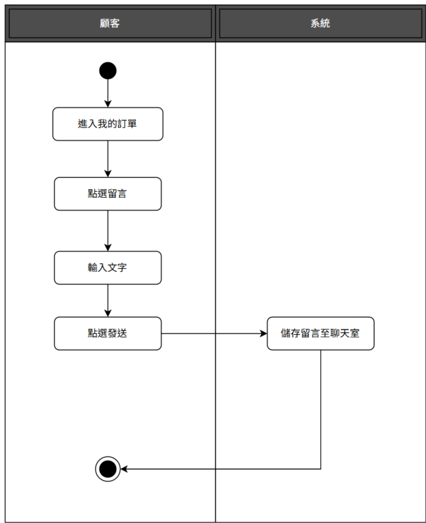
圖 5-3-10 活動圖之訂單留言板-顧客端
