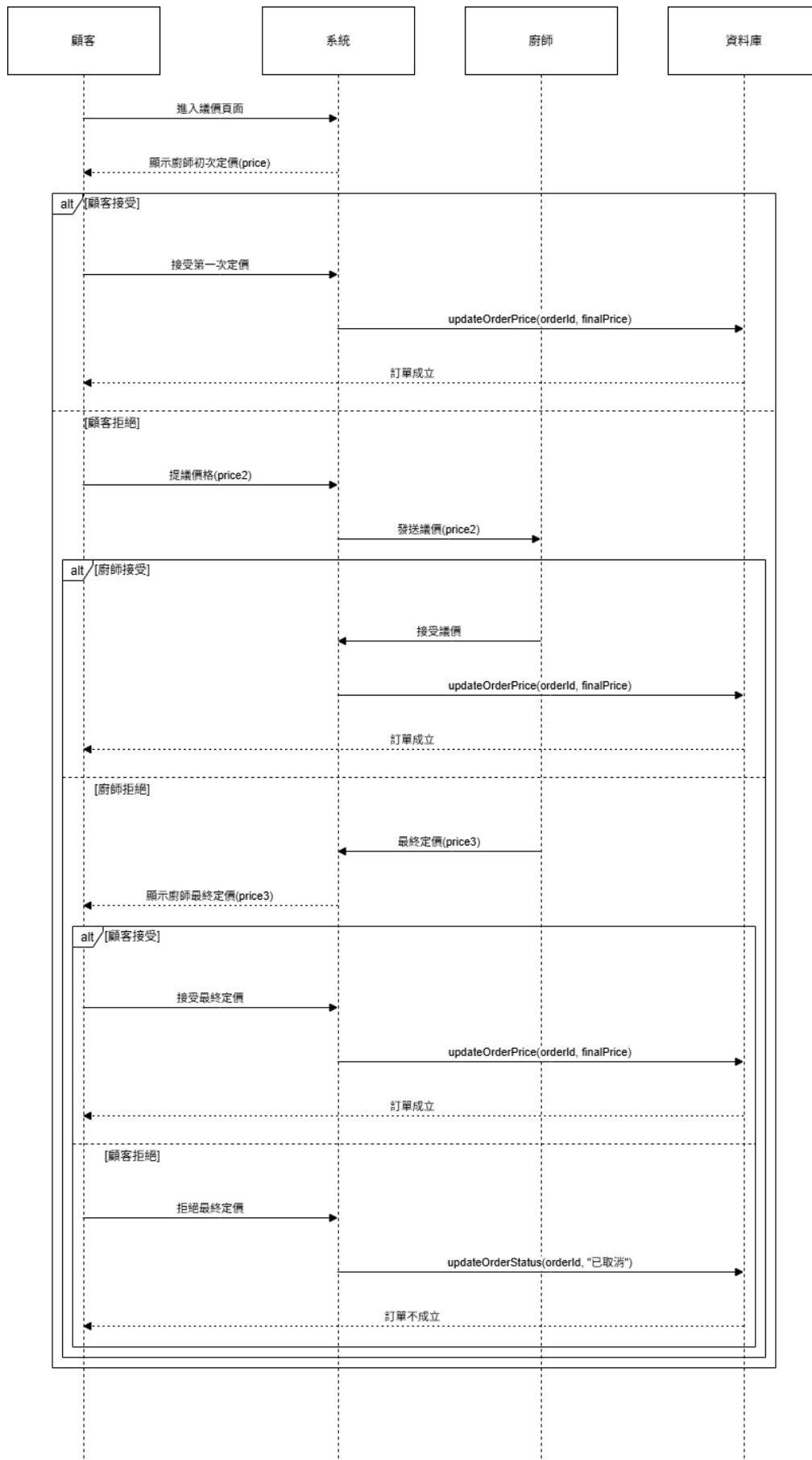
圖 6-1-8 循序圖之顧客端議價
