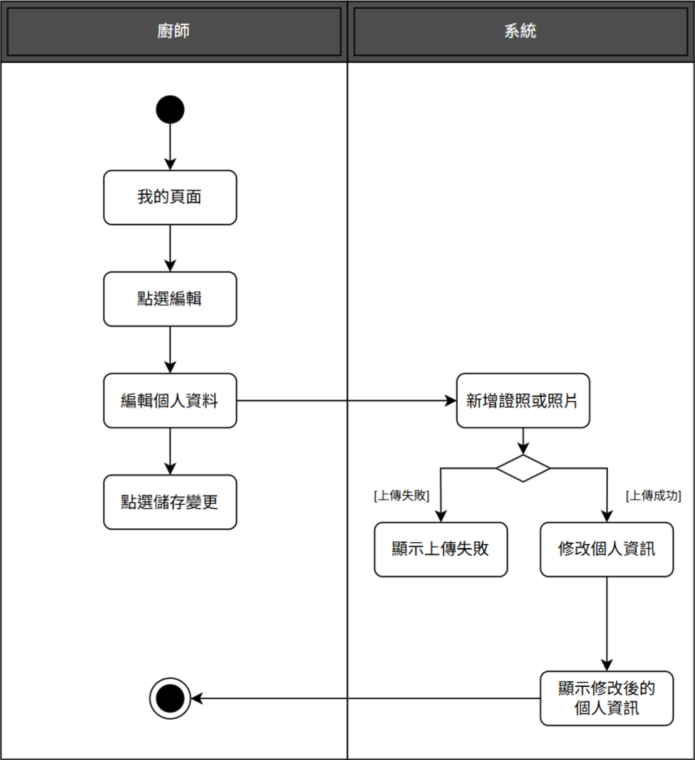
圖 5-3-12 活動圖之編輯個人資料-廚師端
