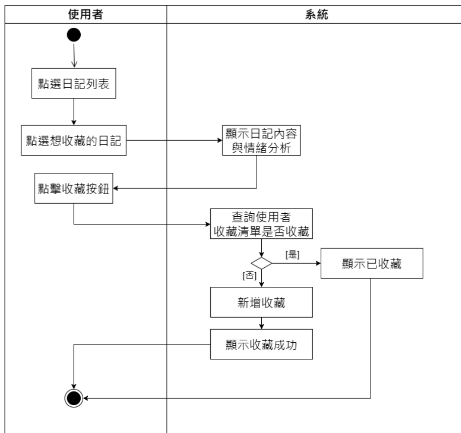
▲圖 5-3-5 收藏活動圖
