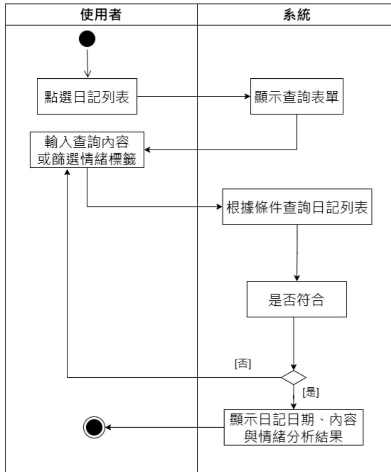
▲圖 5-3-4 查詢歷史日記活動圖
