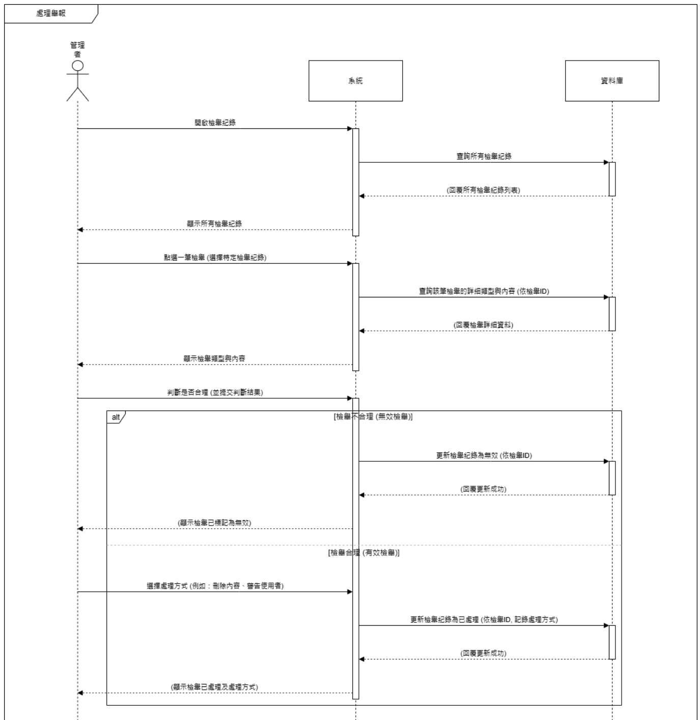
▲圖 6-1- 11 處理舉報循序圖
