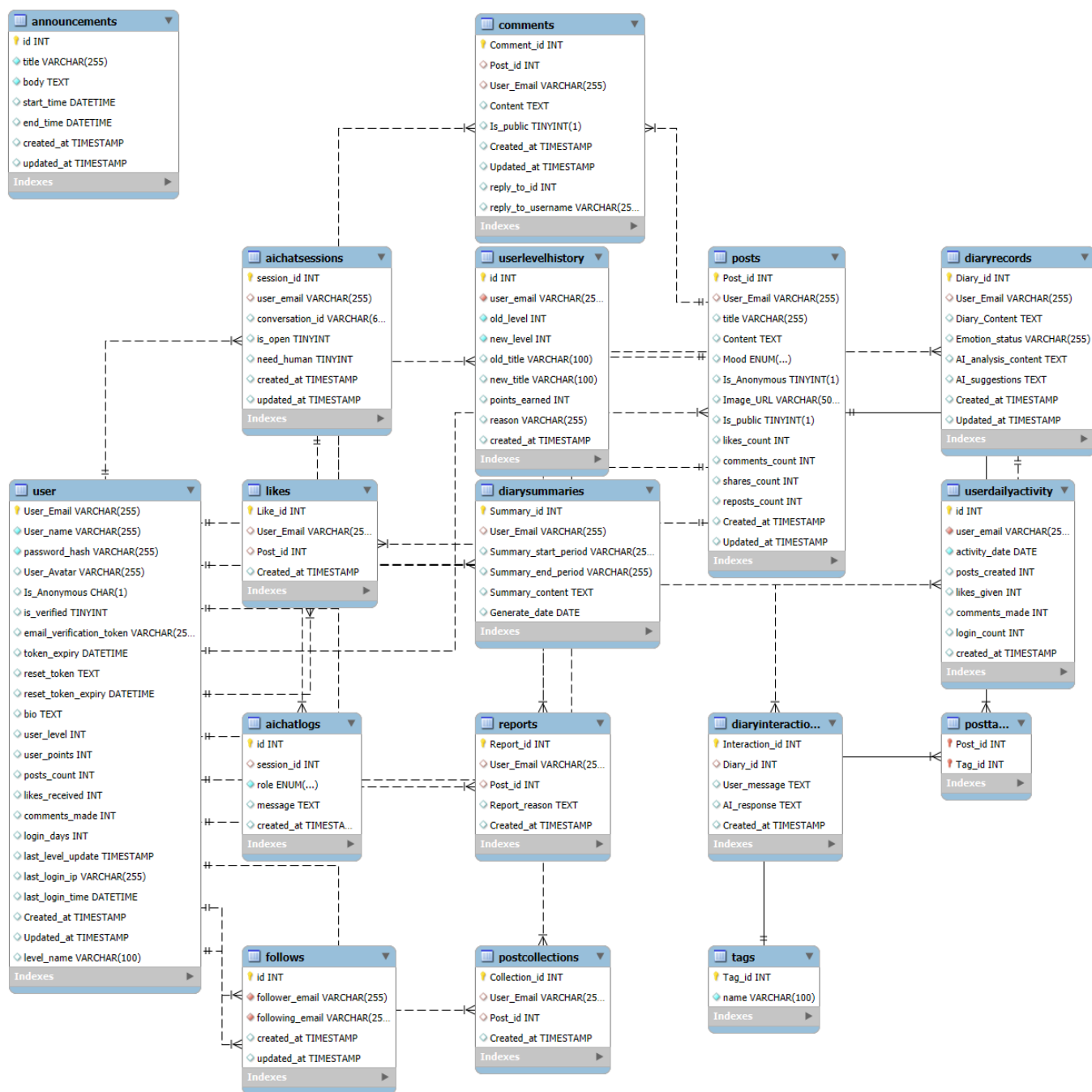
▲圖 8-1-1 資料庫關聯圖
