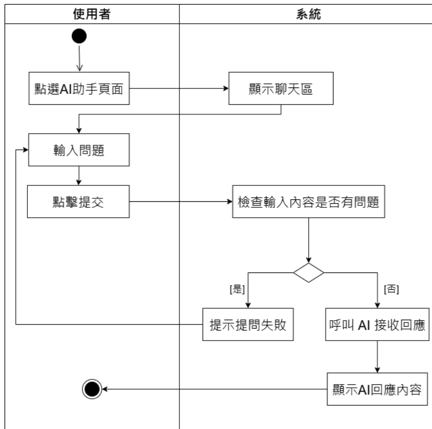
▲圖 5-3- 6 AI 互動活動圖
