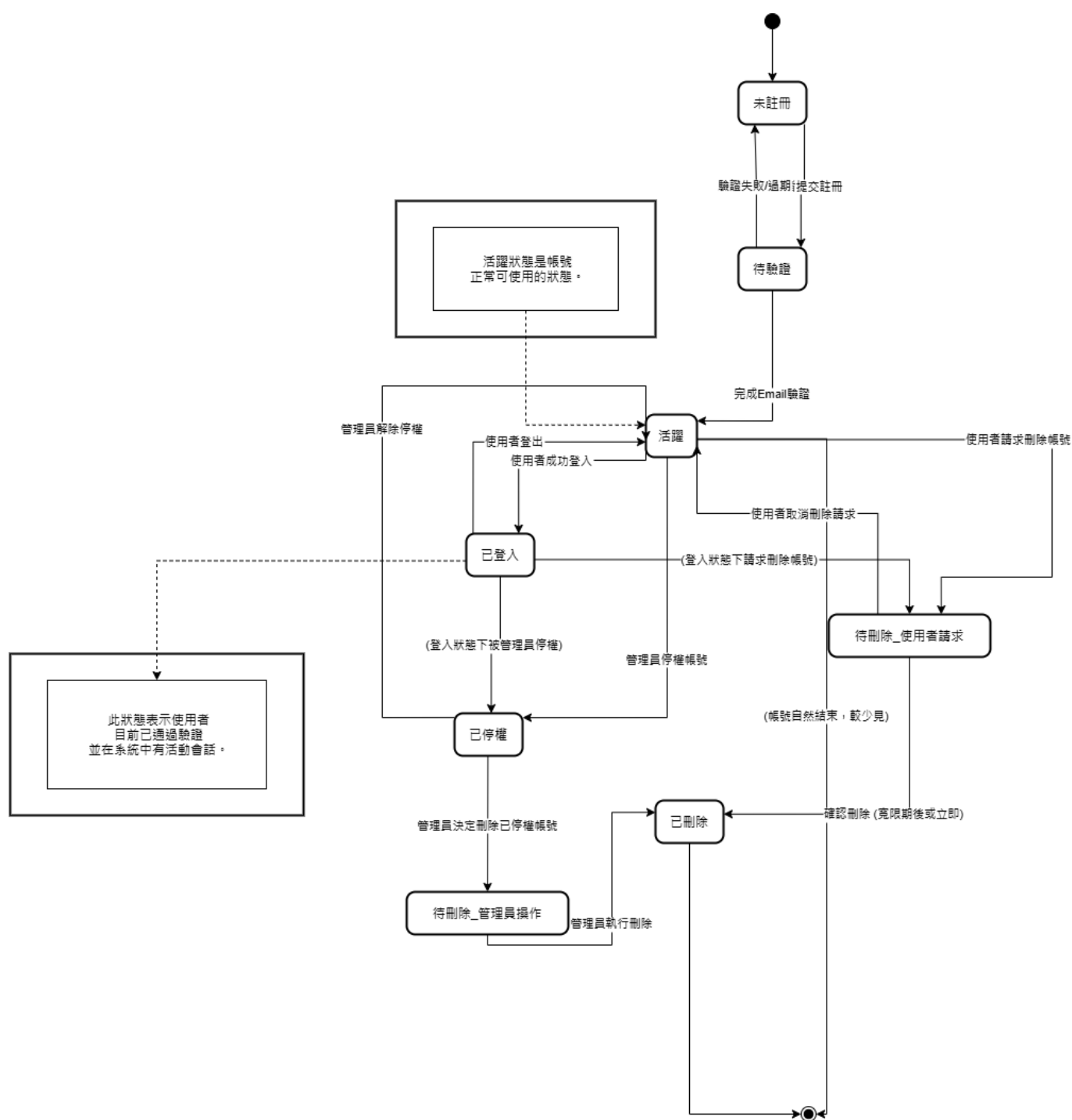
▲圖 7-4- 1 使用者帳號之狀態機
