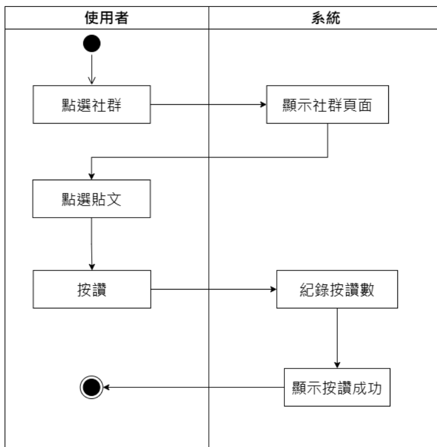
▲圖 5-3- 9 按讚活動圖
