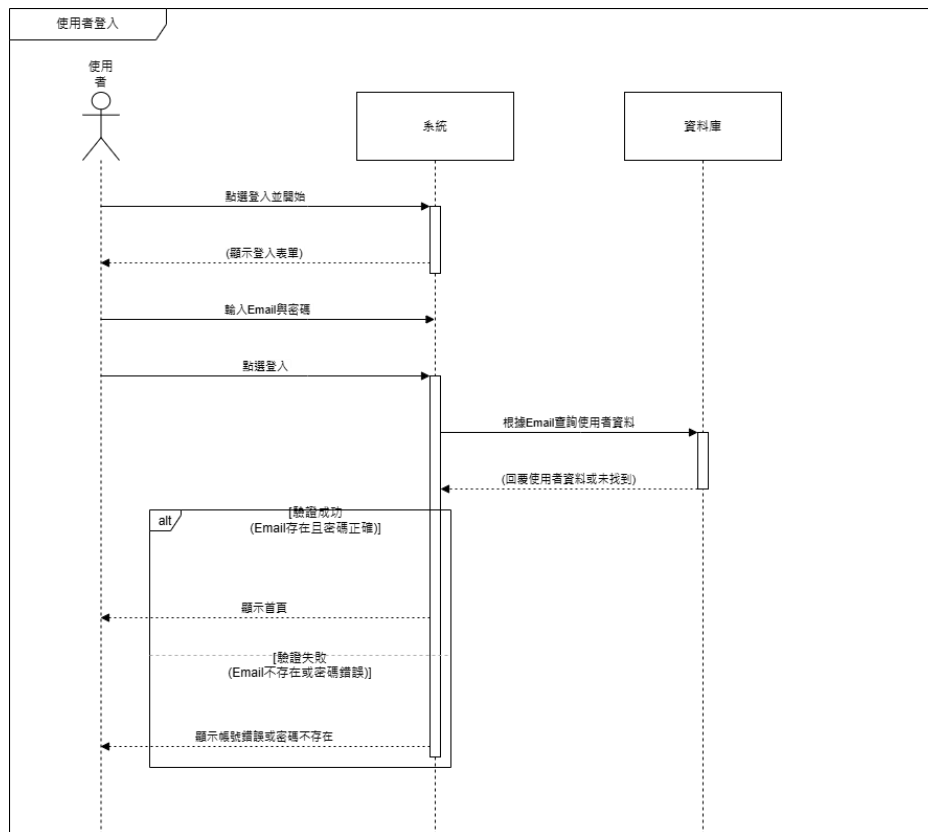
▲圖 6-1-2 登入循序圖
