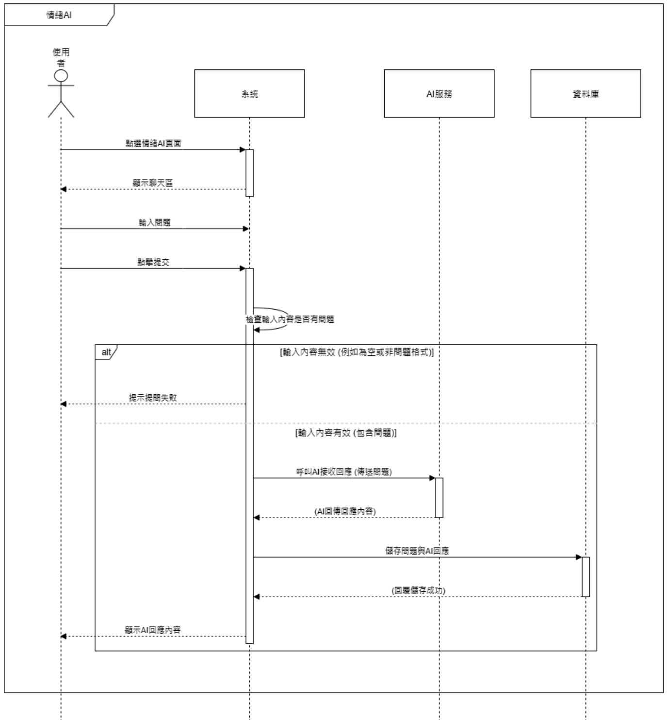
▲圖 6-1-12 情緒 AI 循序圖
