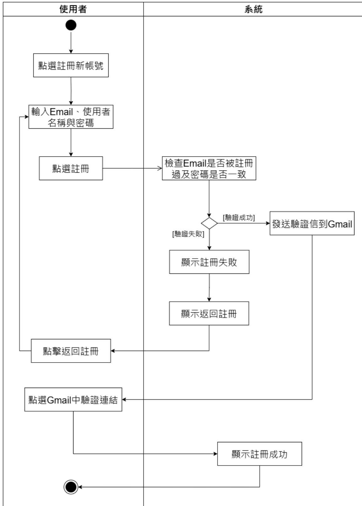
▲圖 5-3- 1 註冊活動圖
