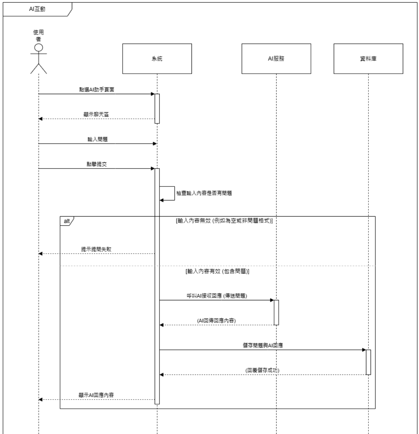
▲圖 6-1- 6 AI 互動循序圖
