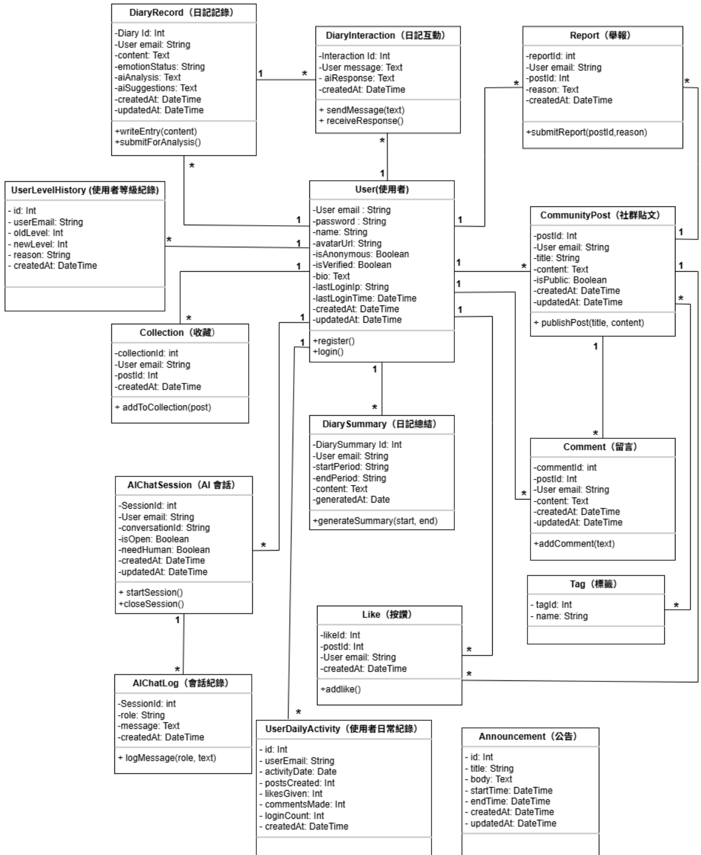
▲圖 6-2- 1 設計類別圖
