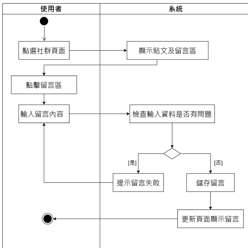
▲圖 5-3- 8 留言活動圖
