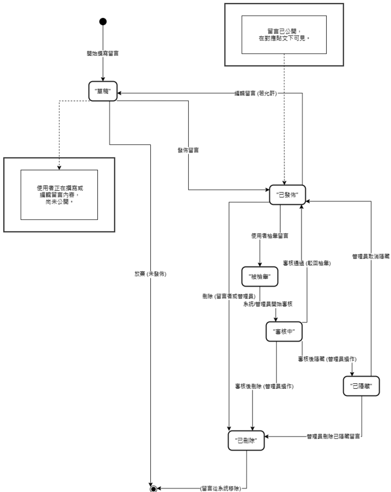
▲圖 7-4-3 社群留言之狀態機
