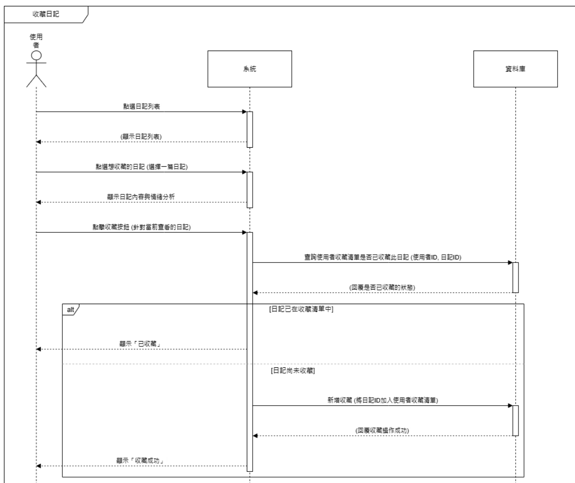
▲圖 6-1-5 收藏循序圖
