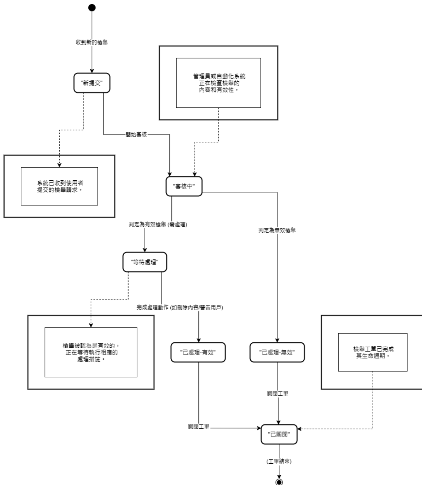
▲圖 7-4-5 舉報之狀態機
