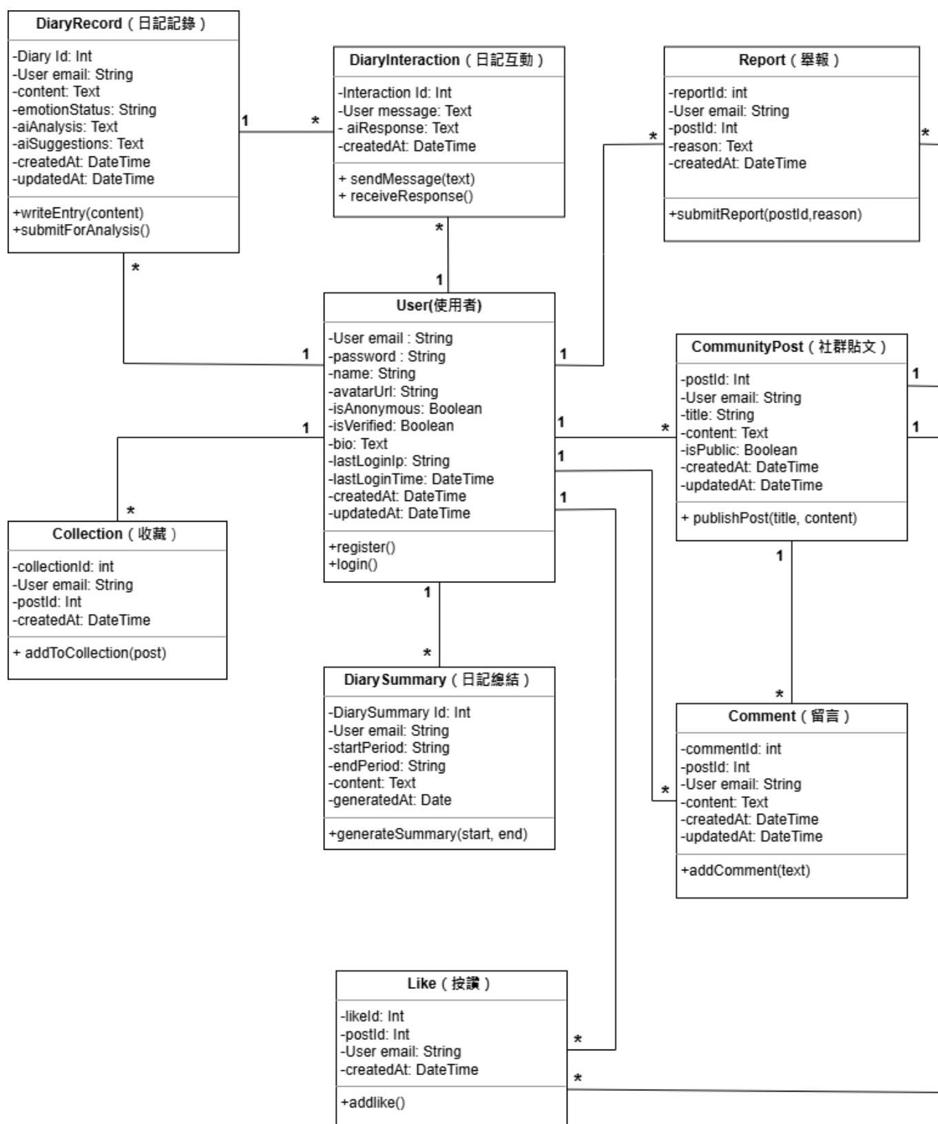
▲圖 5-4- 1 分析類別圖
