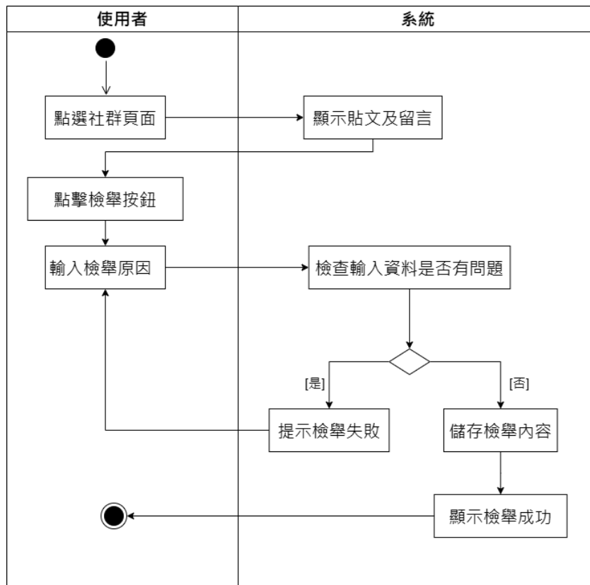
▲圖 5-3- 10 舉報活動圖
