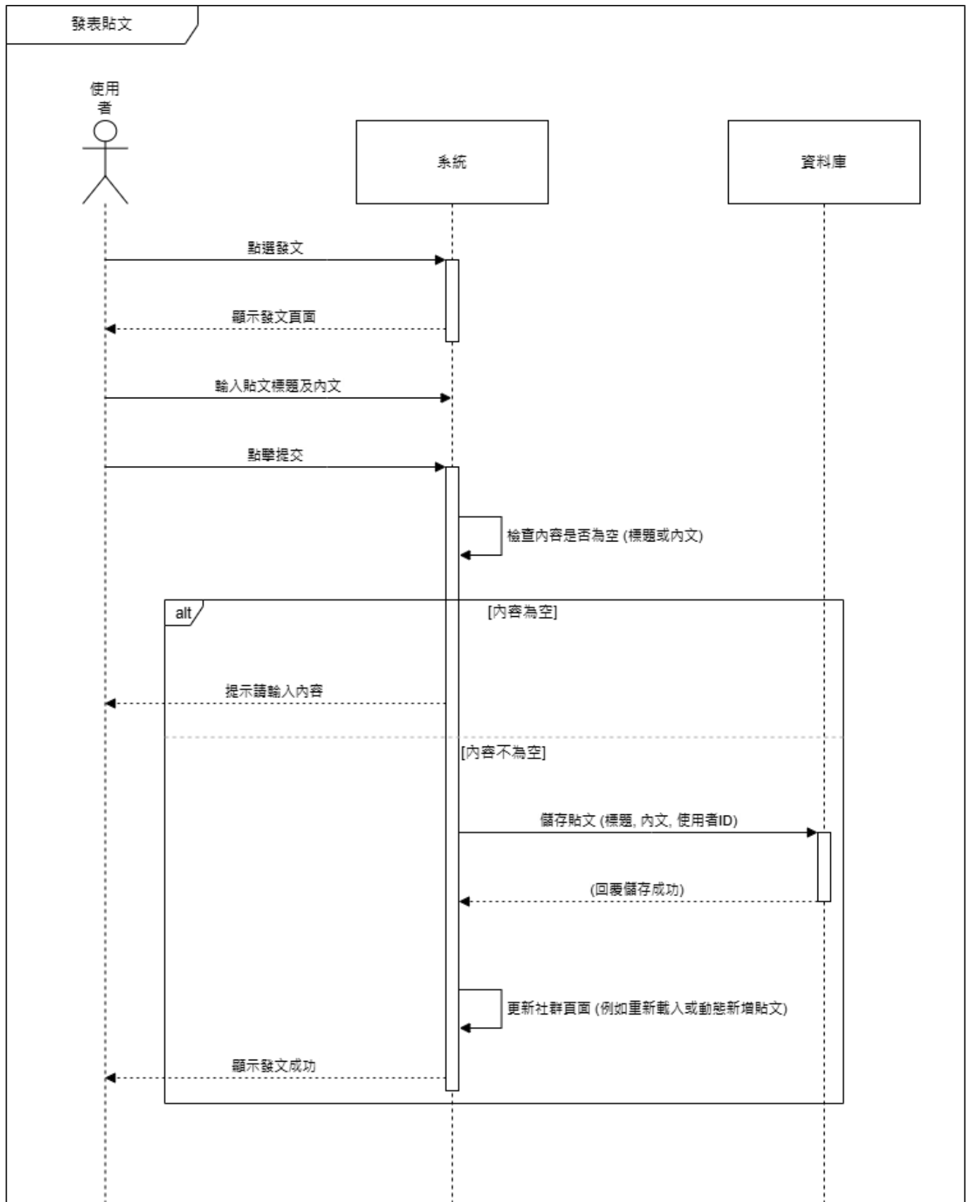
▲圖 6-1-7 發表貼文循序圖
