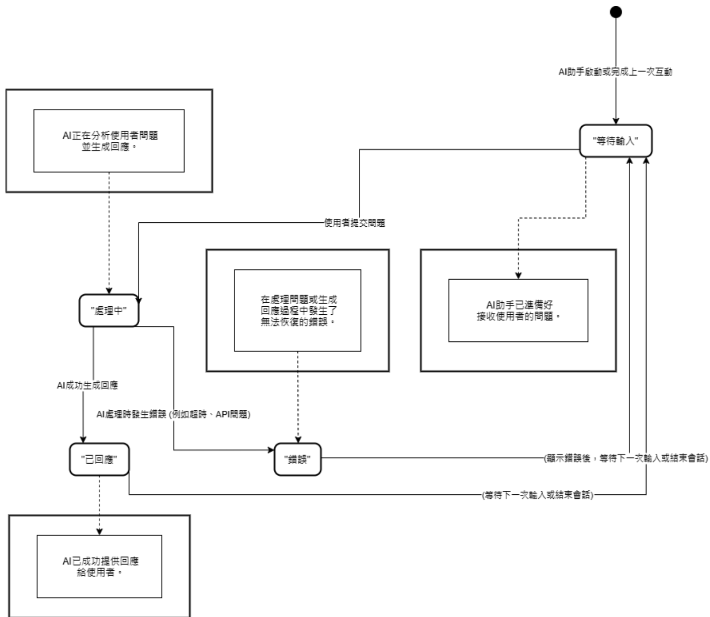
▲圖 7-4- 6 AI 互動會話之狀態機
