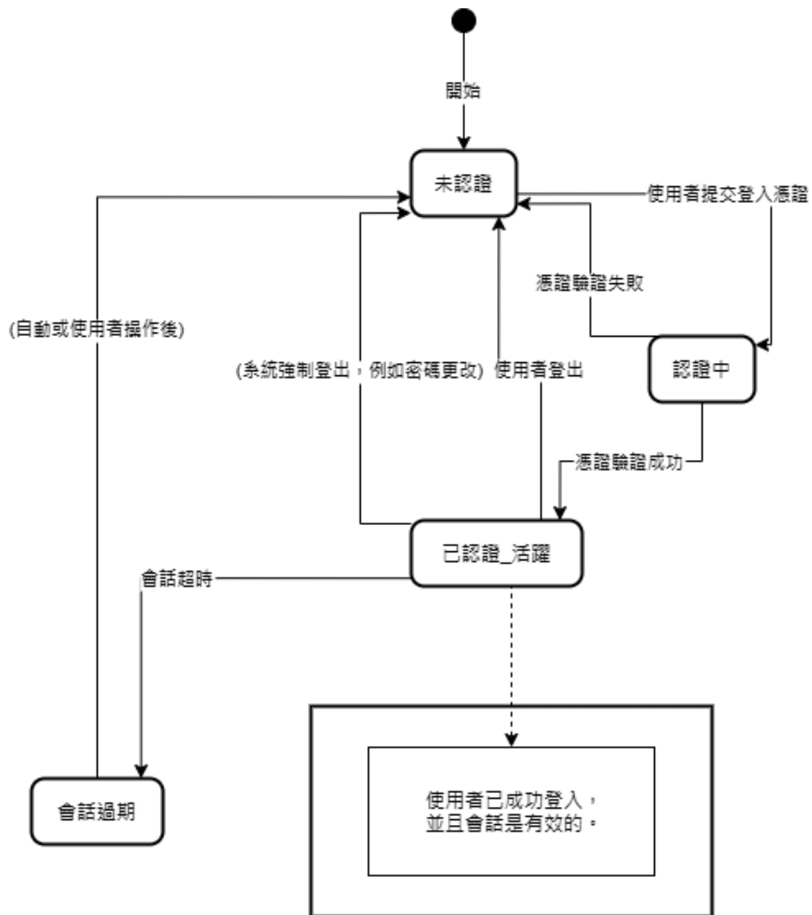
▲圖 7-4-2 使用者會話之狀態機
