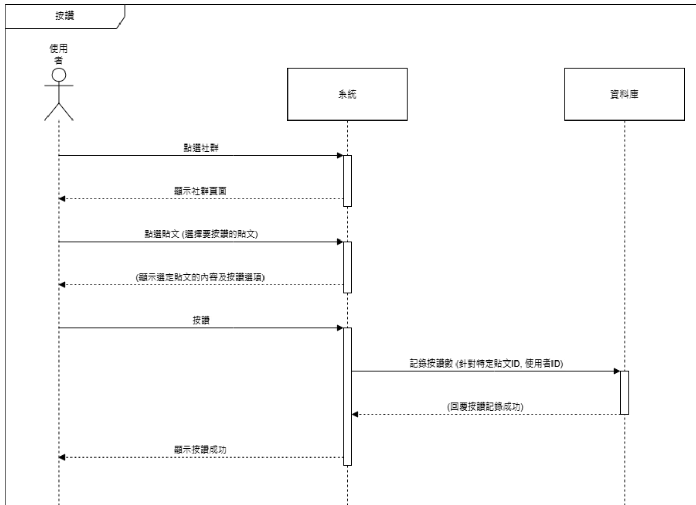
▲圖 6-1-9 按讚循序圖
