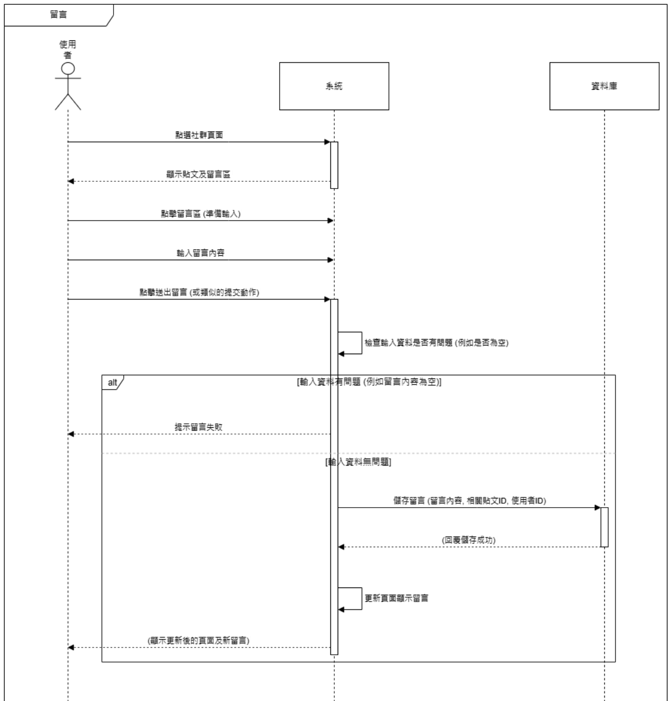
▲圖 6-1-8 留言循序圖
