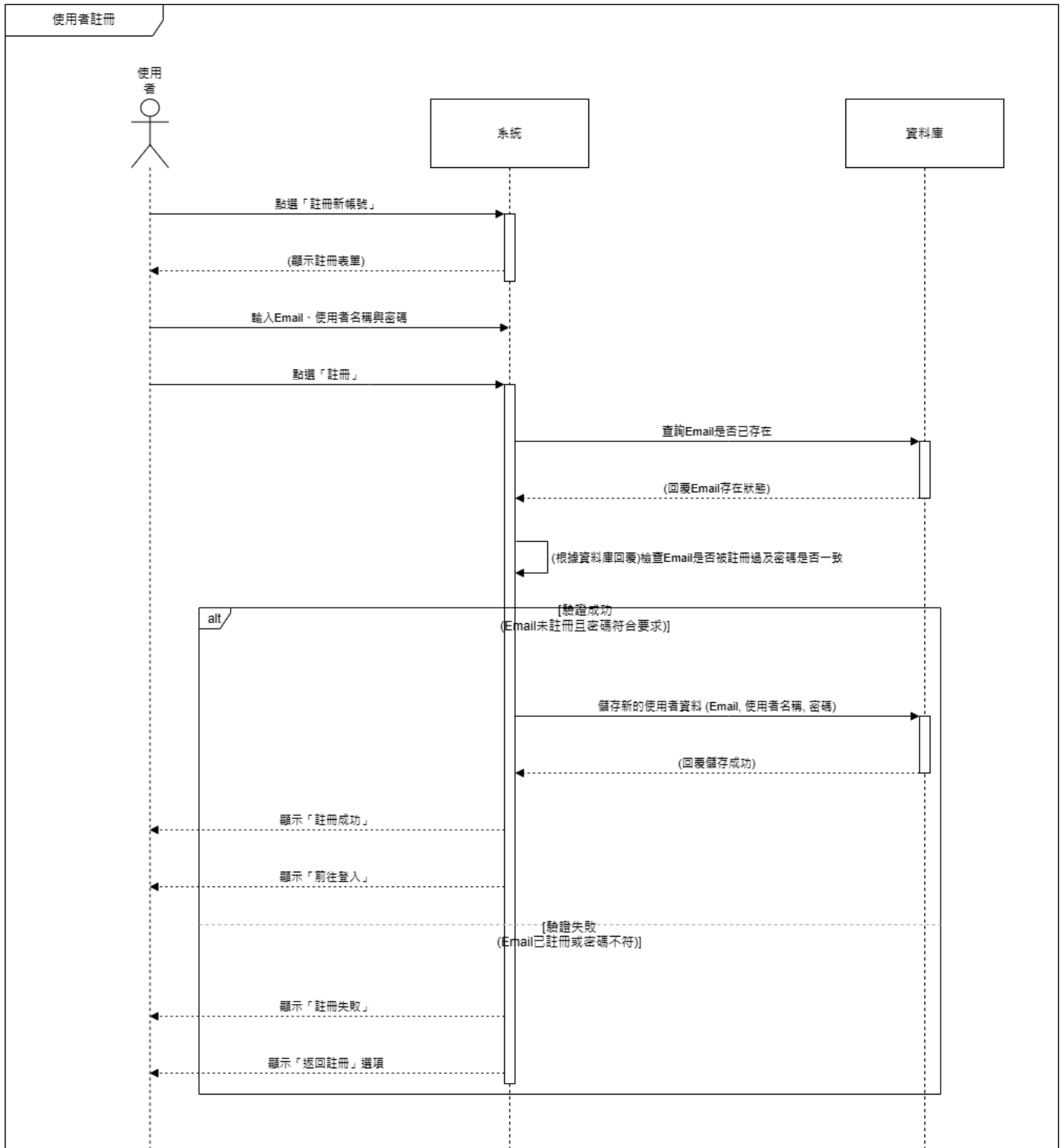
▲圖 6-1- 1 註冊循序圖
