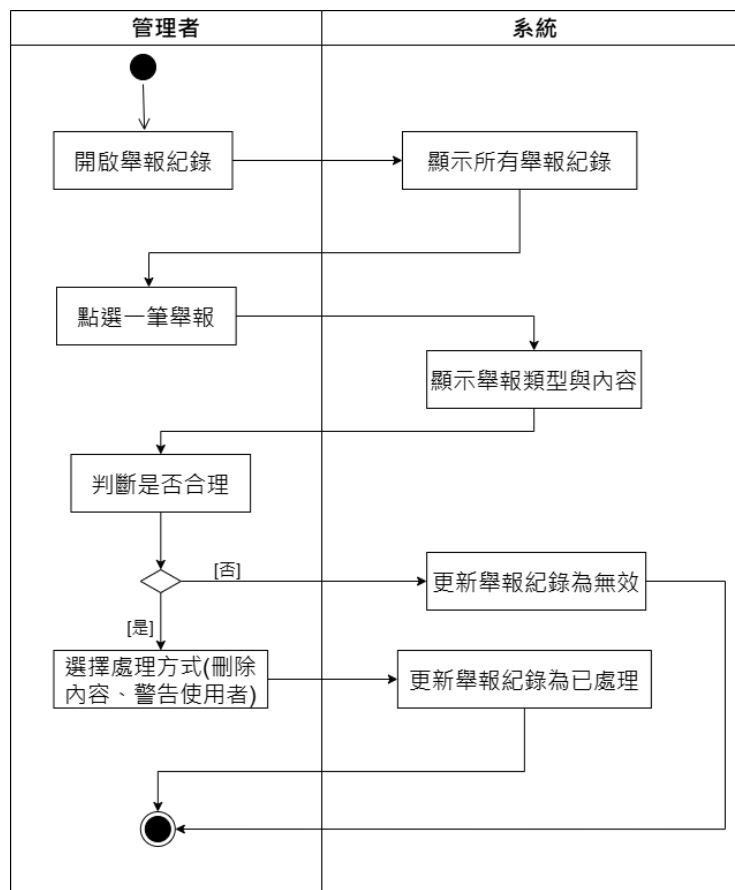
▲圖 5-3- 11 處理舉報活動圖
