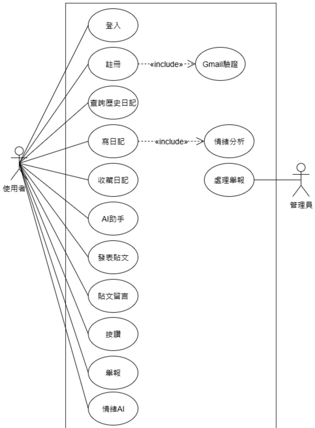
▲圖 5-2- 1 使用個案圖
