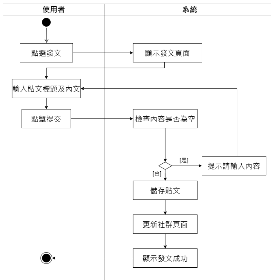
▲圖 5-3- 7 發表貼文活動圖
