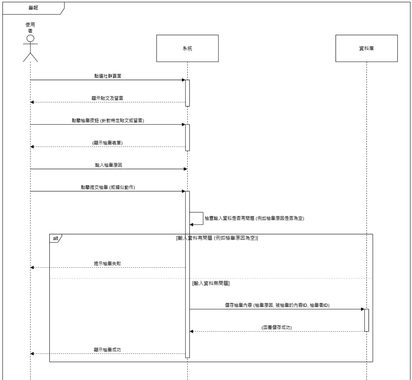
▲圖 6-1-10 舉報循序圖
