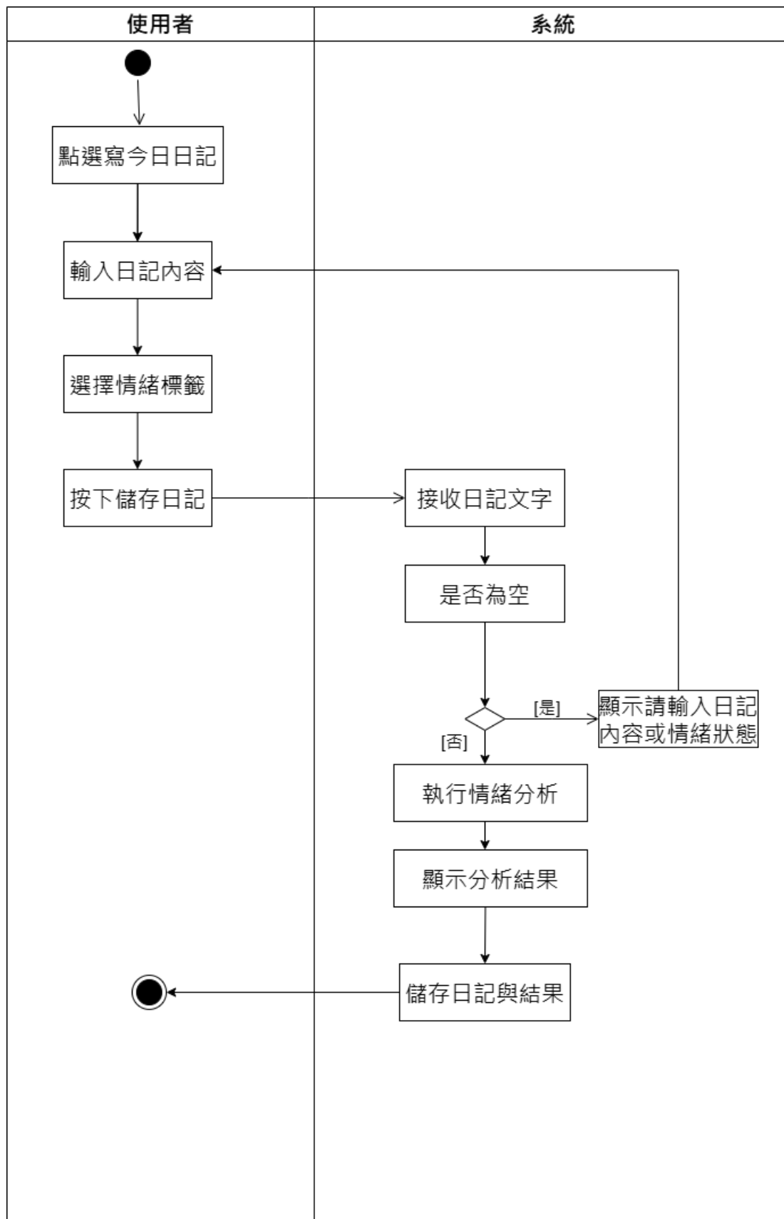
▲圖 5-3-3 寫日記活動圖
