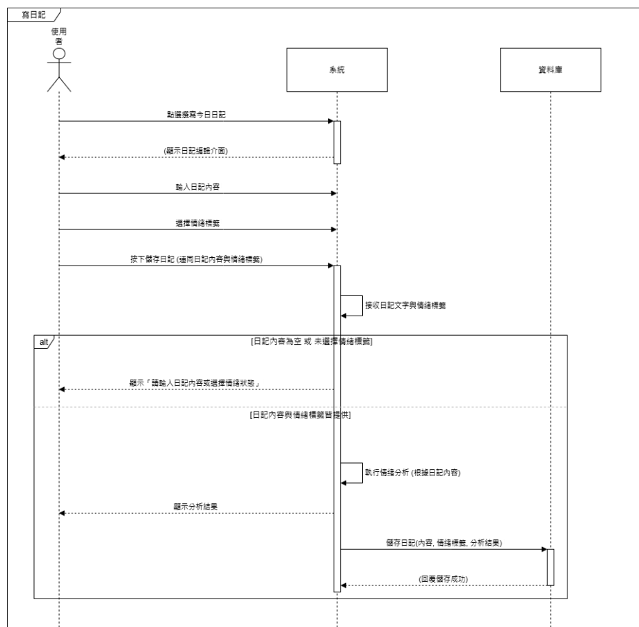
▲圖 6-1-3 寫日記循序圖
