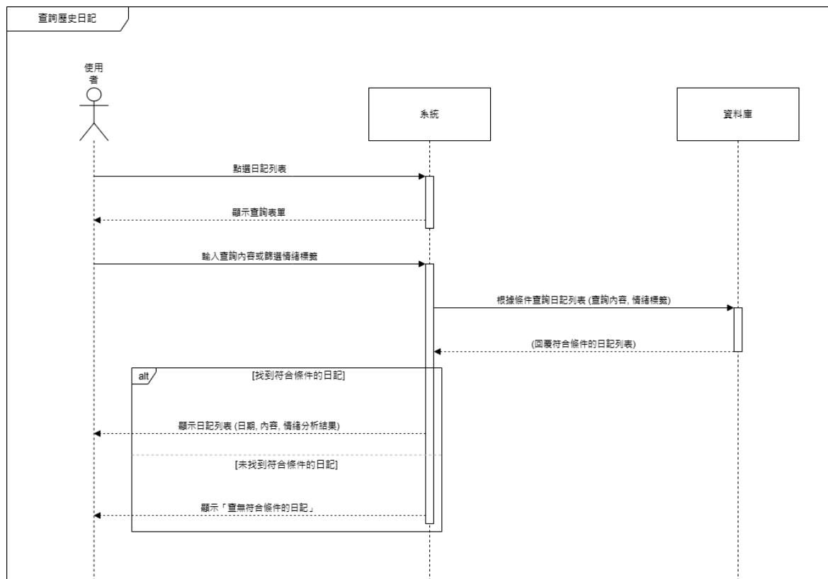
▲圖 6-1-4 查詢歷史日記循序圖
