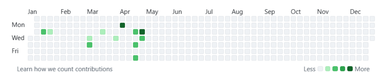
圖 4-3-3 GitHub 記錄
