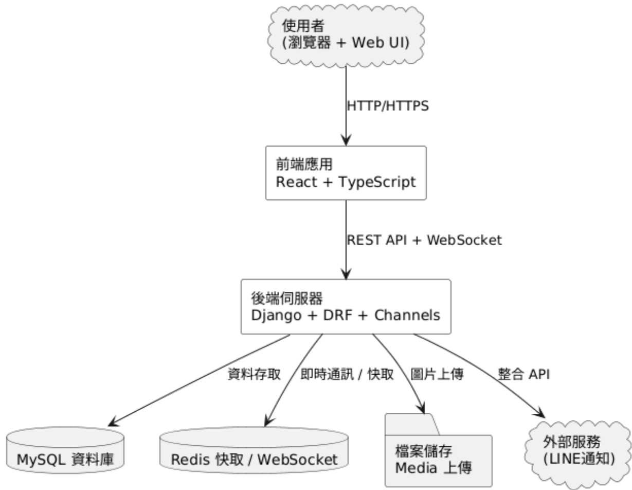
圖 3-1-1 系統架構圖
