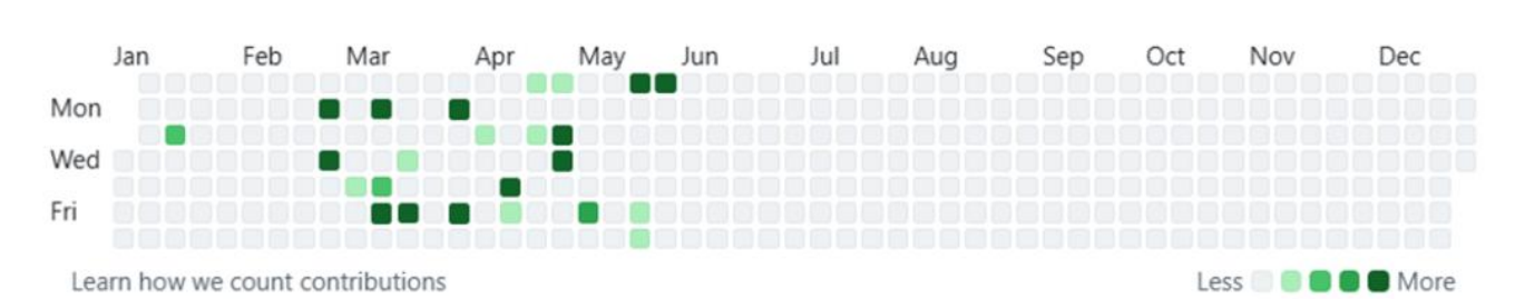
圖 4-3-4 GitHub 記錄
