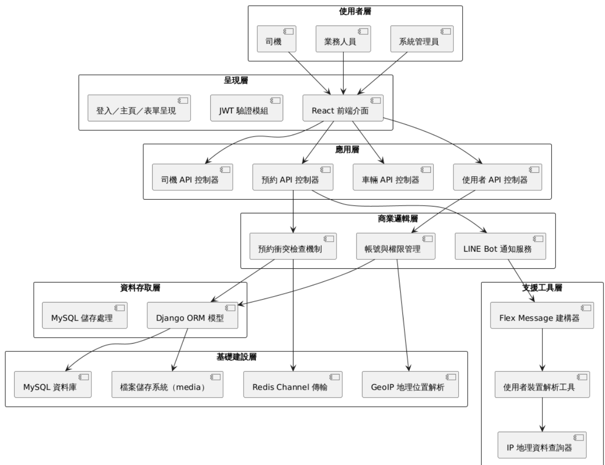
圖 7-2-1 套件圖
