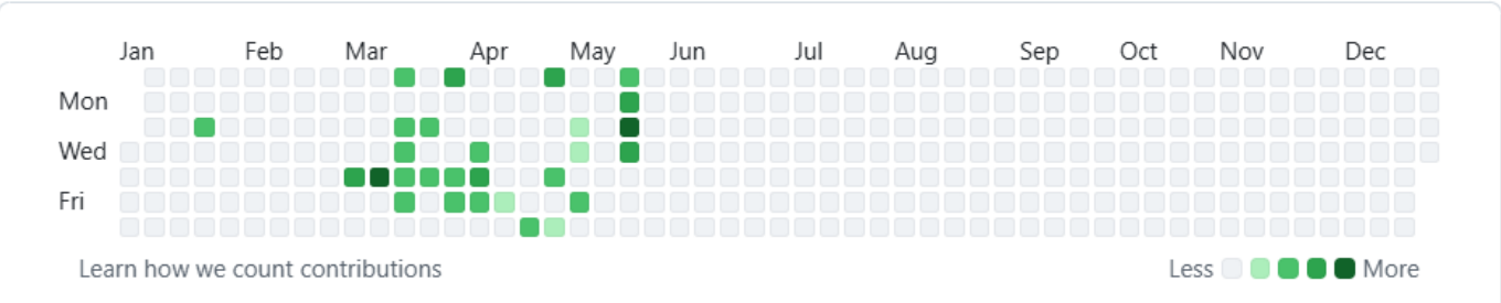
圖 4-3-1 GitHub 記錄
