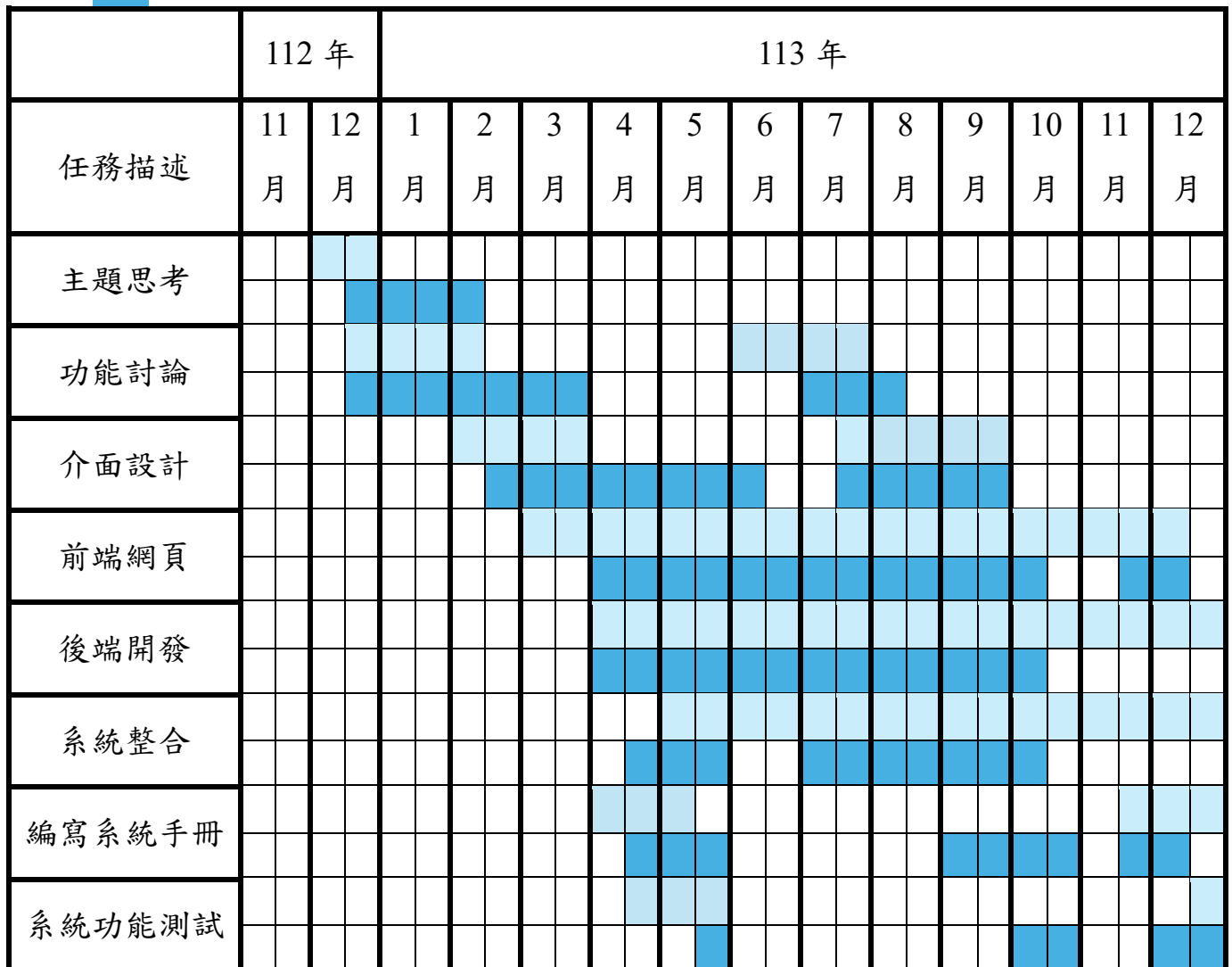
圖 4-1-1 甘特圖
