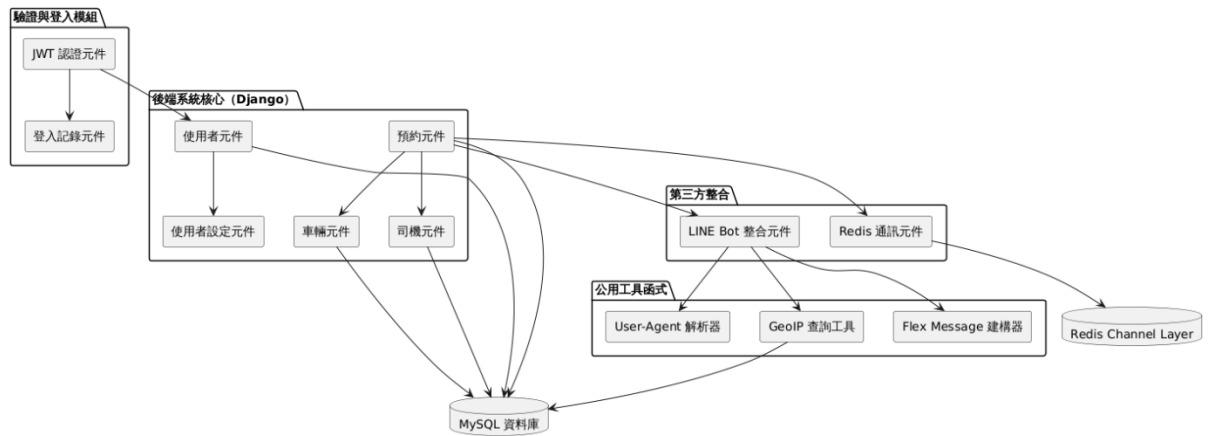
圖 7-3-1 元件圖
