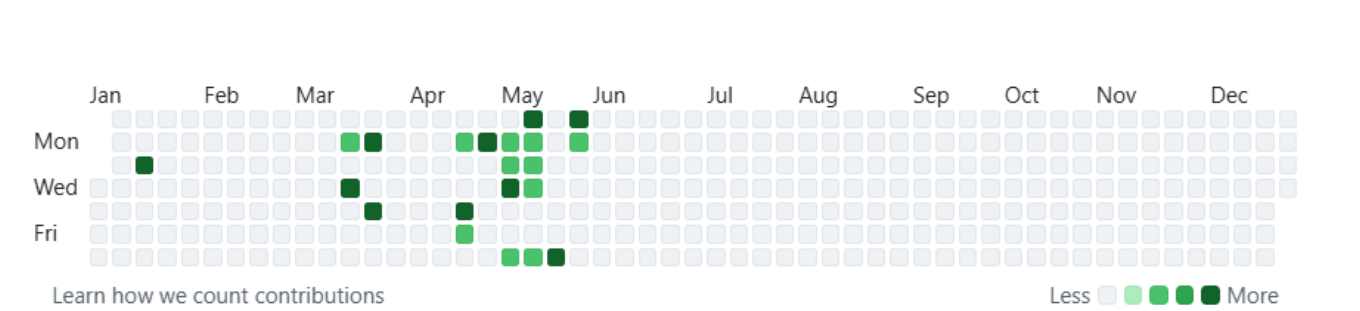
圖 4-3-2 GitHub 記錄
