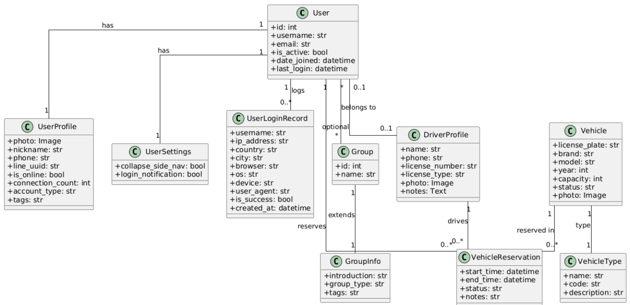
圖 6-2-1 設計類別圖
