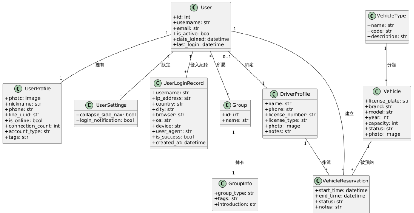
圖 5-4-1 分析類別圖
