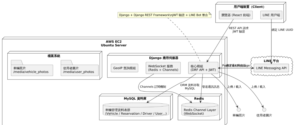
圖 7-1-1 佈署圖
