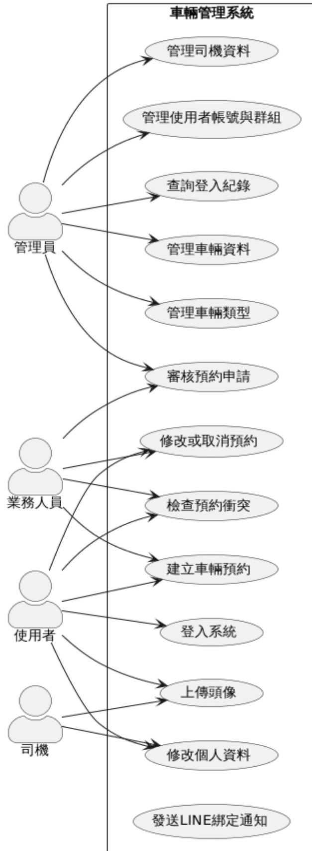
圖 5-2-1 使用個案圖
