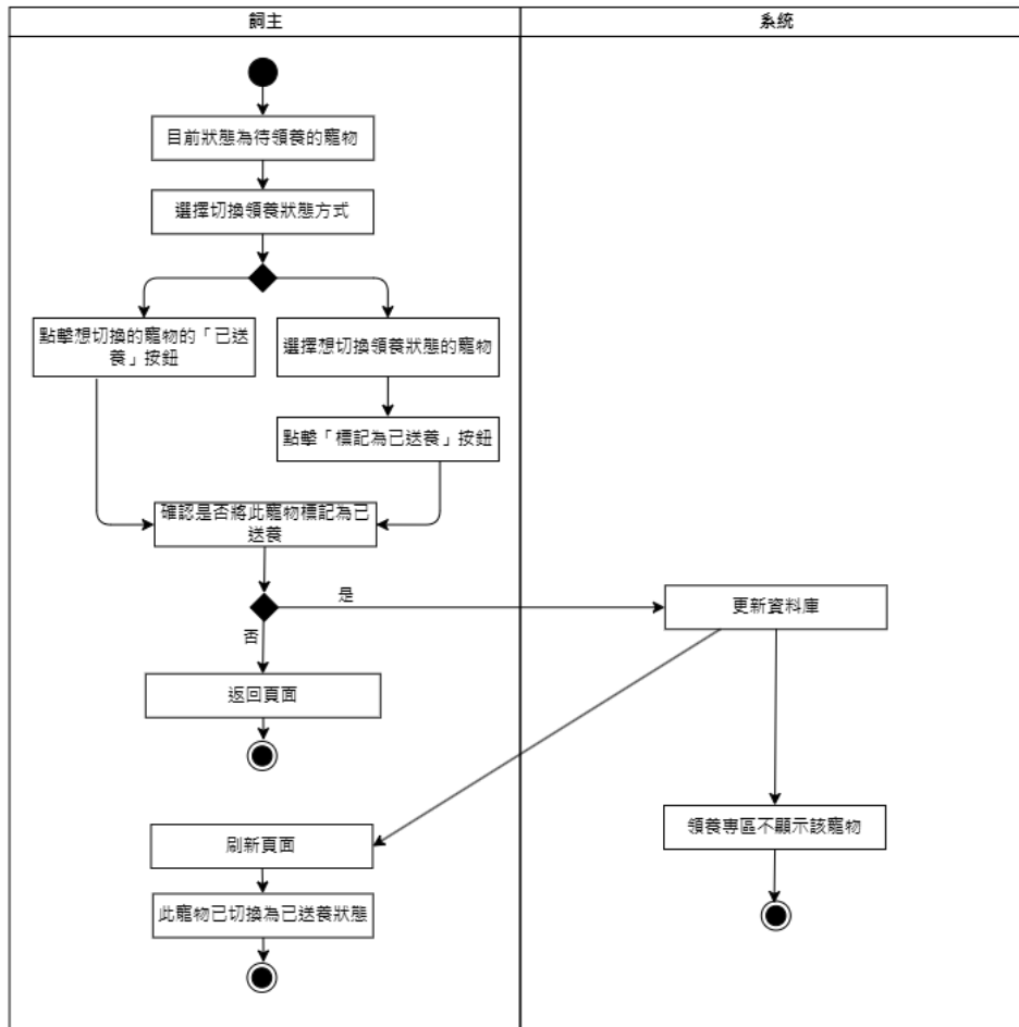
圖 5-3-20 切換為已送養狀態活動圖
