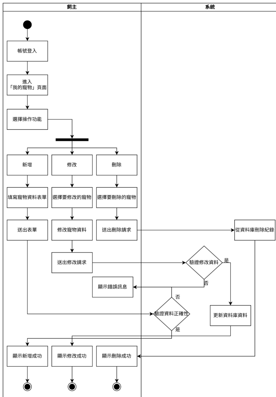
圖 5-3-4 寵物管理活動圖
