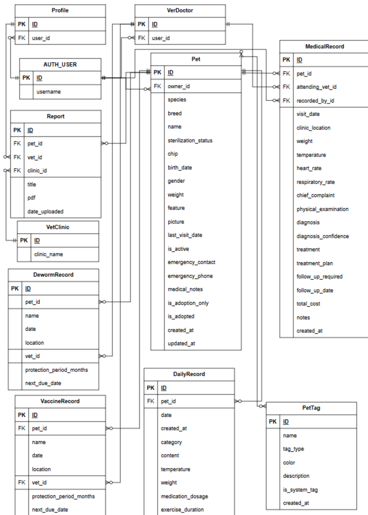
圖 8-1-3 資料庫關聯圖：寵物、標籤與日誌
