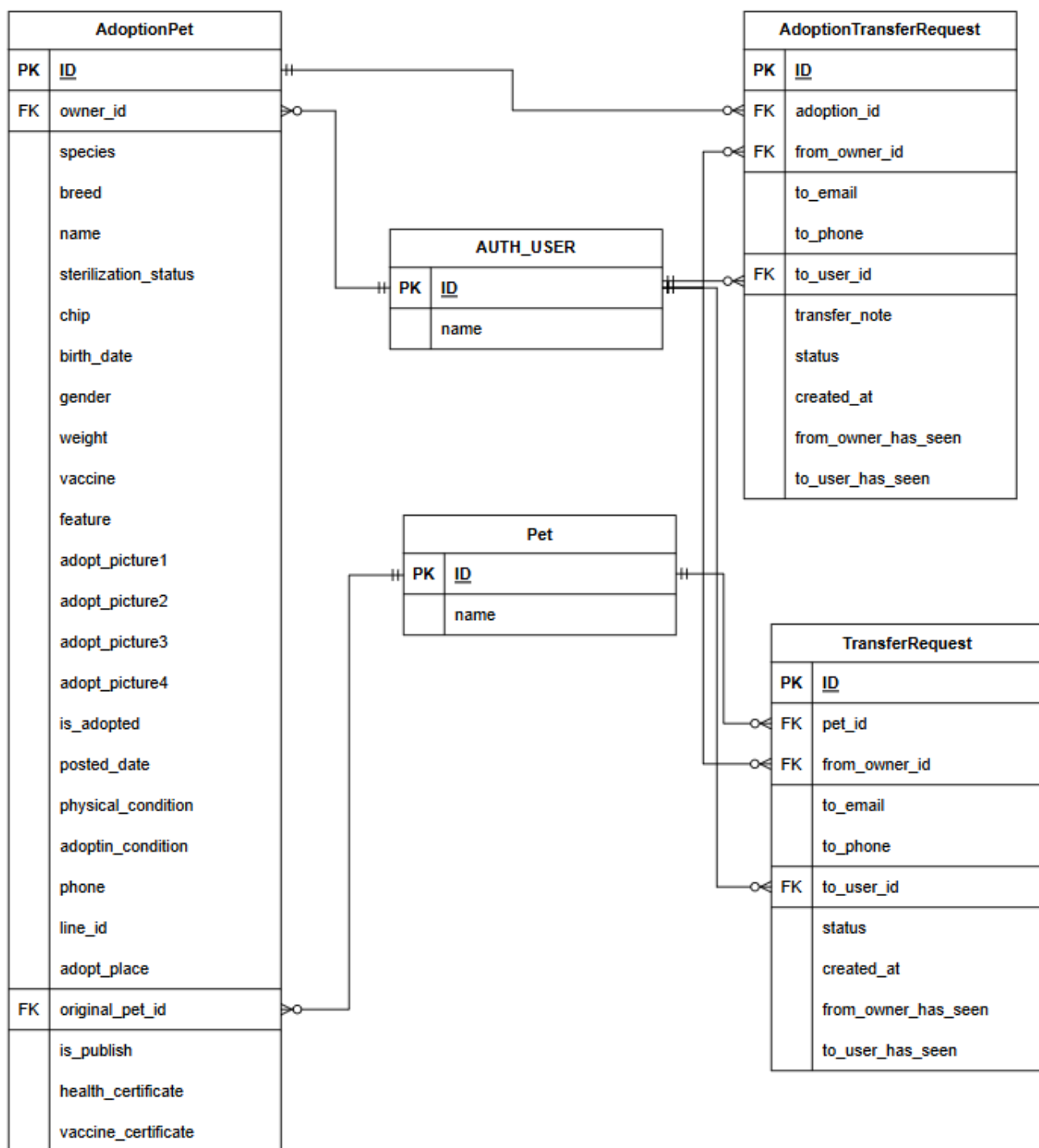
圖 8-1-5 資料庫關聯圖：領養
