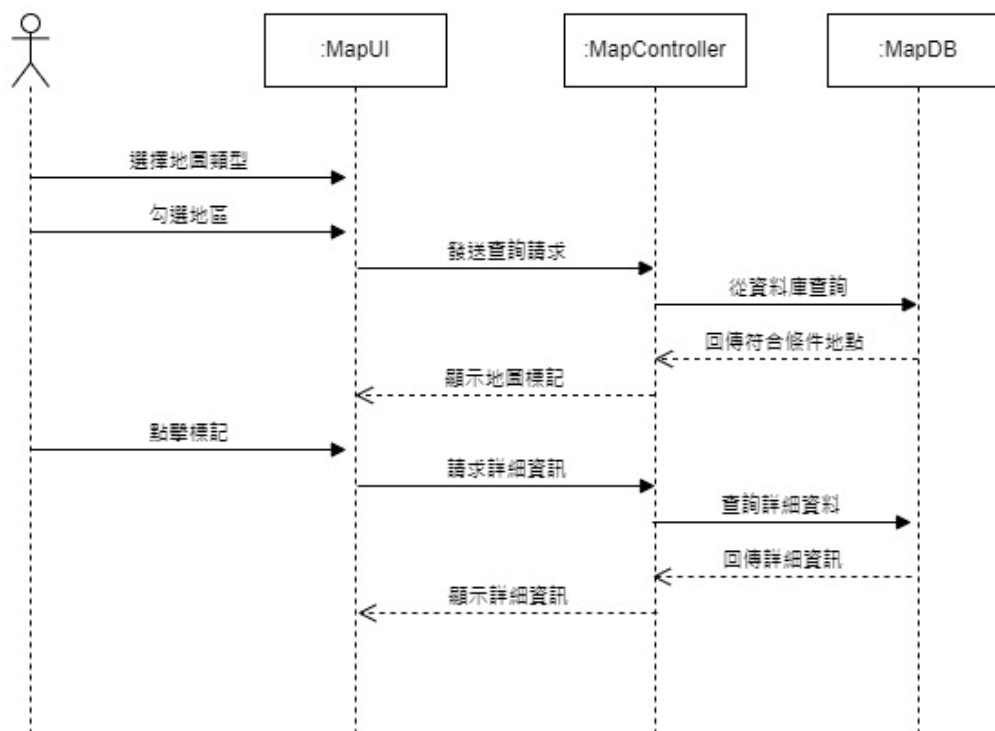
圖 6-1-5 查詢地圖循序圖
