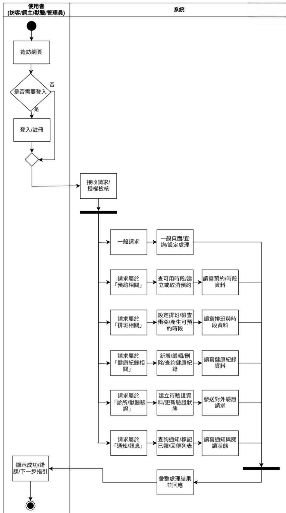
圖 5-3-1 整體系統使用活動圖
