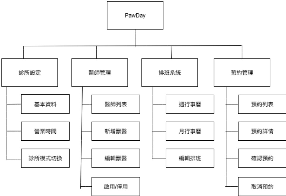
圖 3-1-4 診所管理員網頁架構圖
