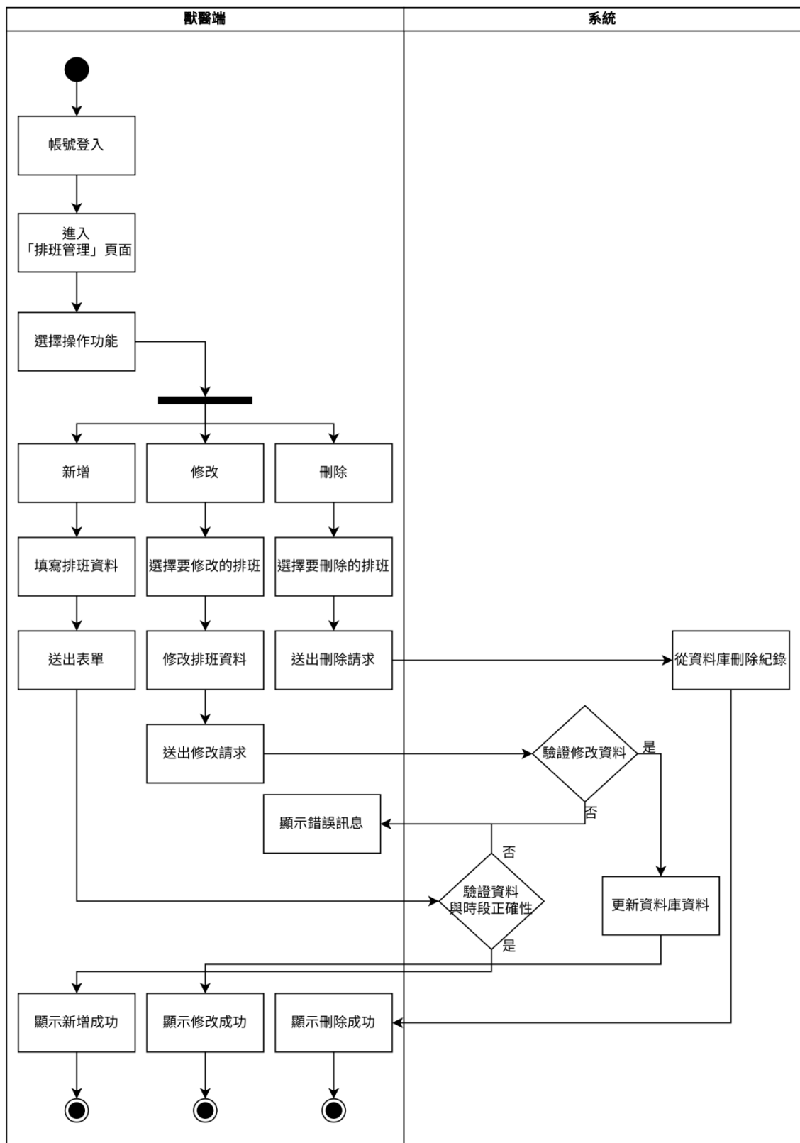
圖 5-3-9 獸醫排班管理活動圖
