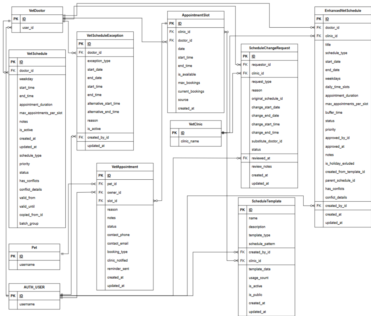
圖 8-1-2 資料庫關聯圖：排班與預約
