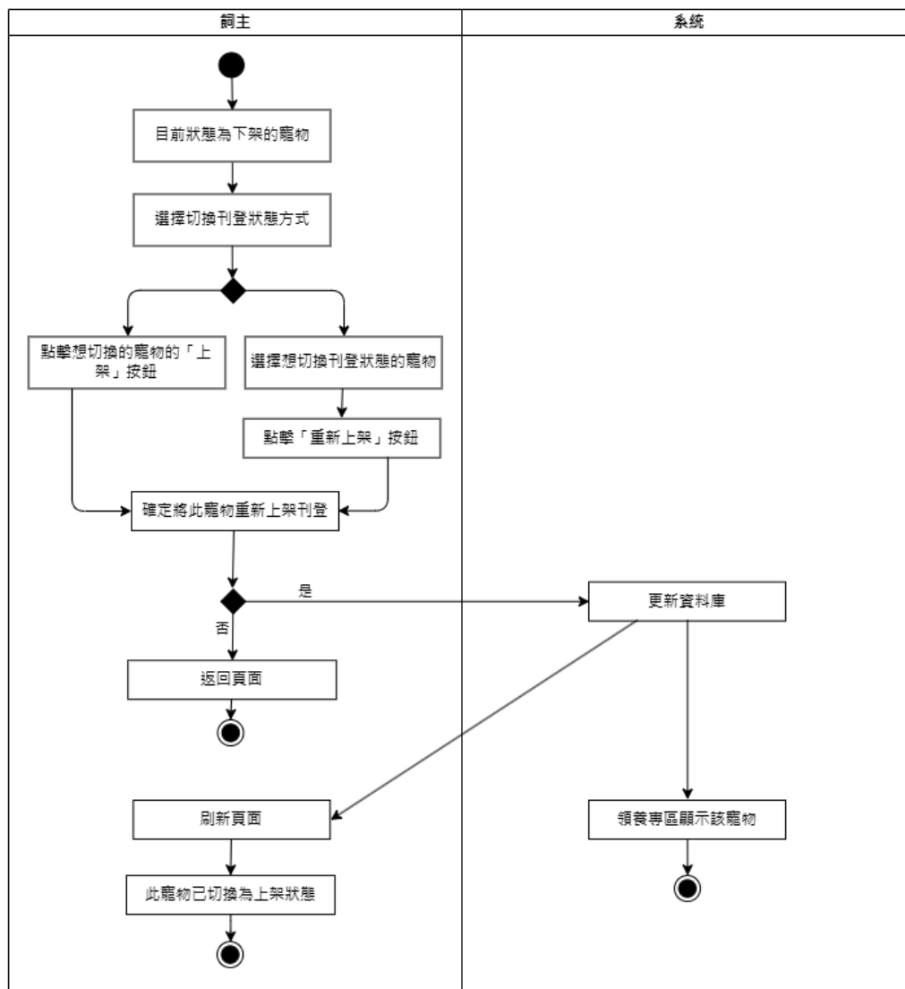
圖 5-3-18 切換為上架狀態活動圖
