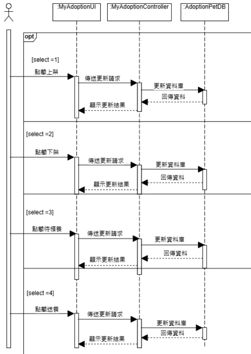
圖 6-1-14 切換狀態循序圖
