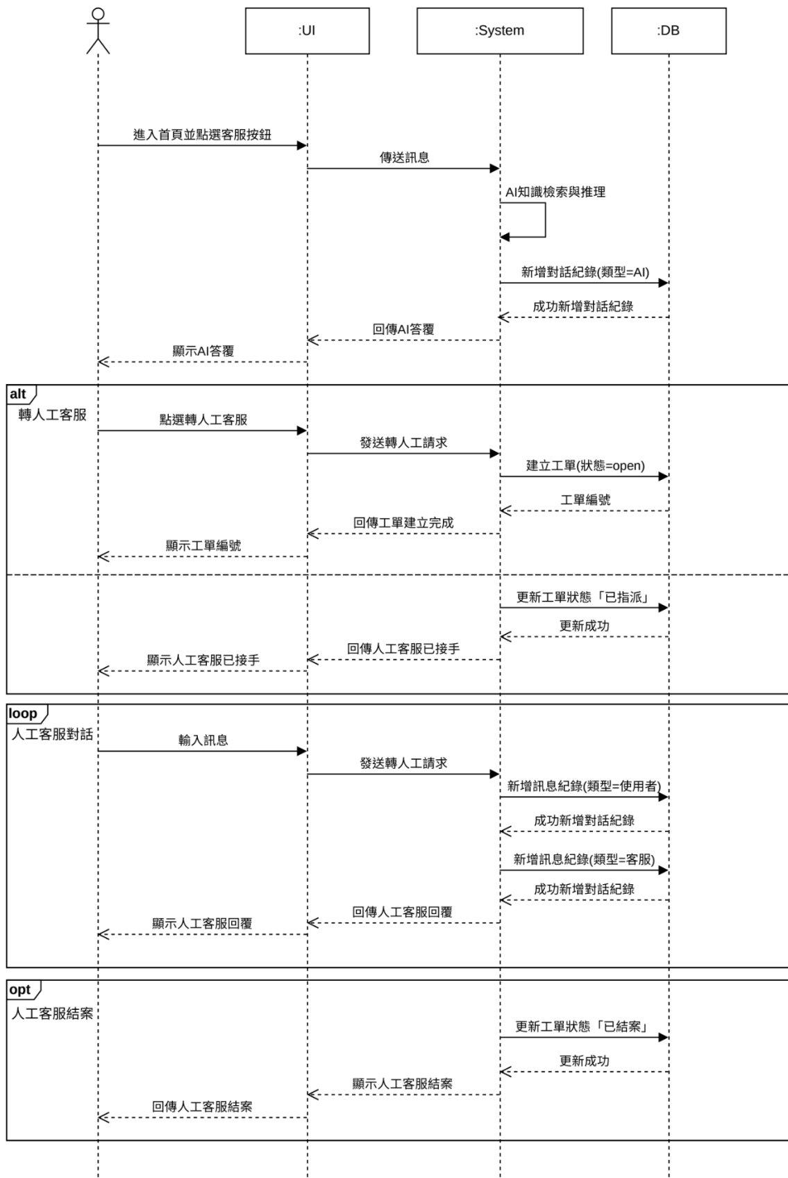
圖 6-1-10 AI/人工客服循序圖
