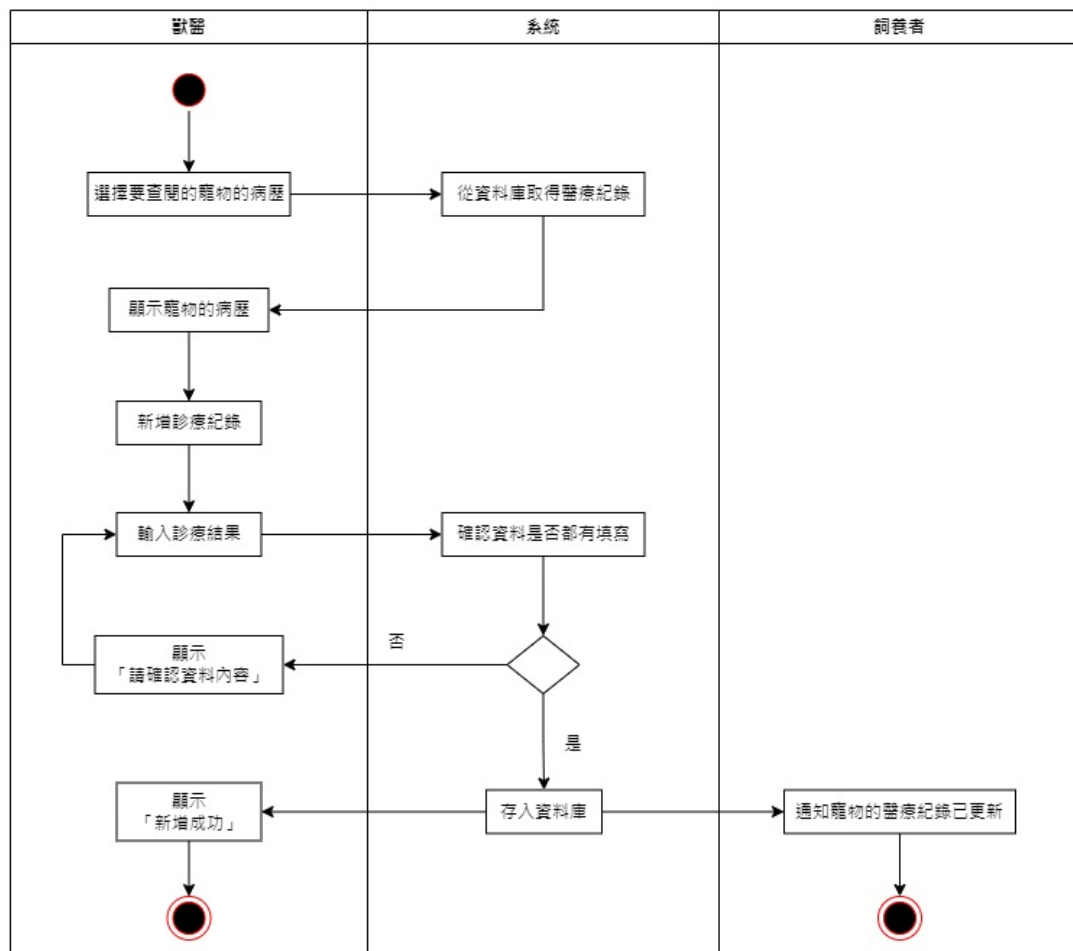
圖 5-3-8 獸醫看診活動圖
