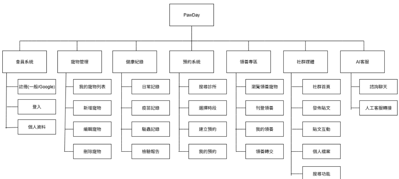
圖 3-1-2 飼主端網頁架構圖
