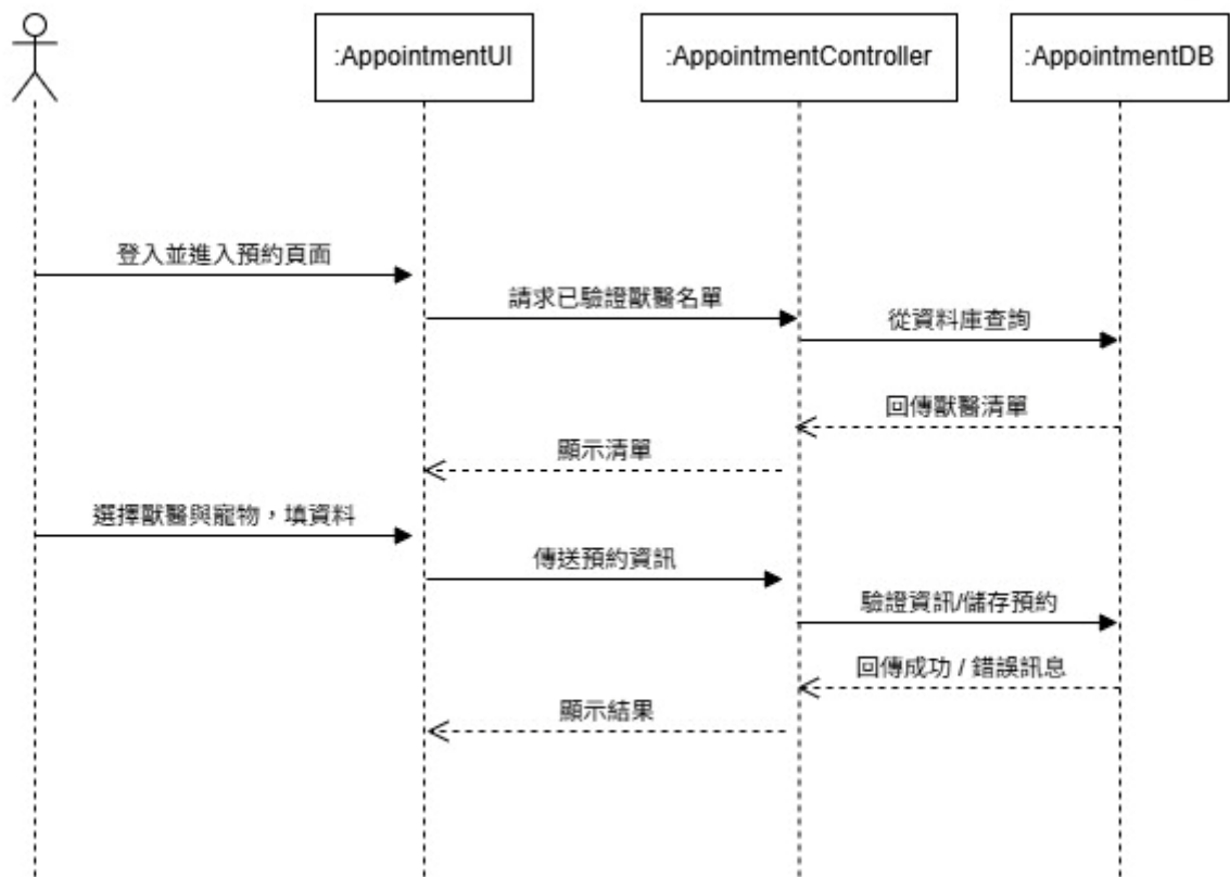
圖 6-1-6 飼主預約獸醫循序圖
