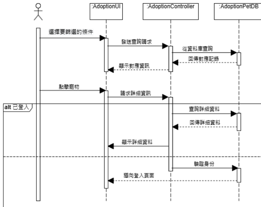
圖 6-1-13 搜尋寵物循序圖
