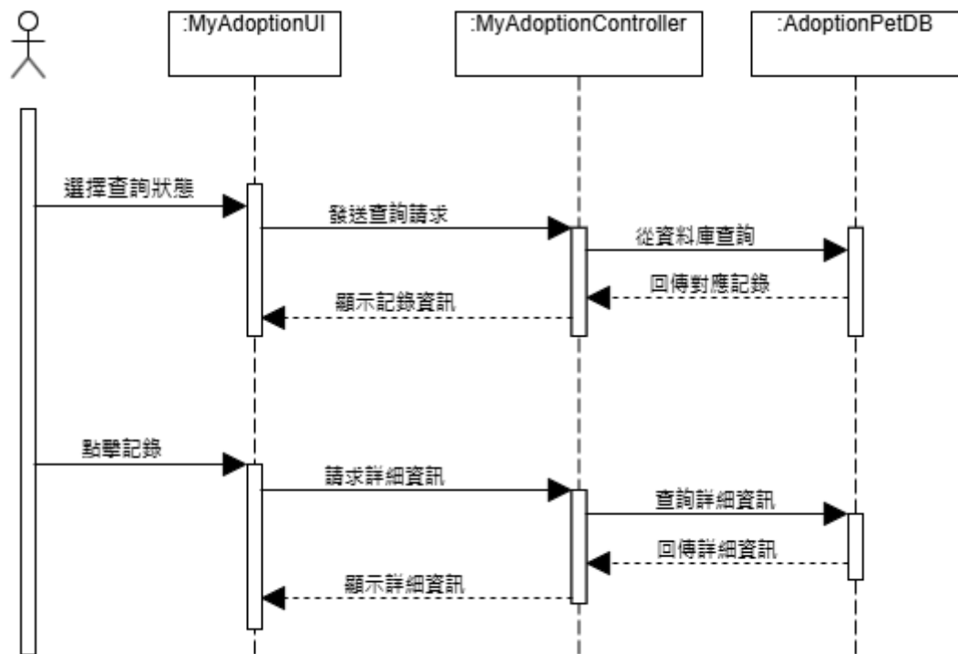
圖 6-1-15 查詢我的送養寵物循序圖
