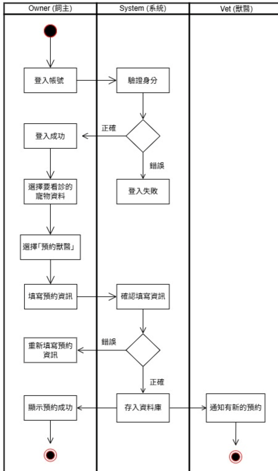
圖 5-3-7 飼主預約獸醫活動圖
