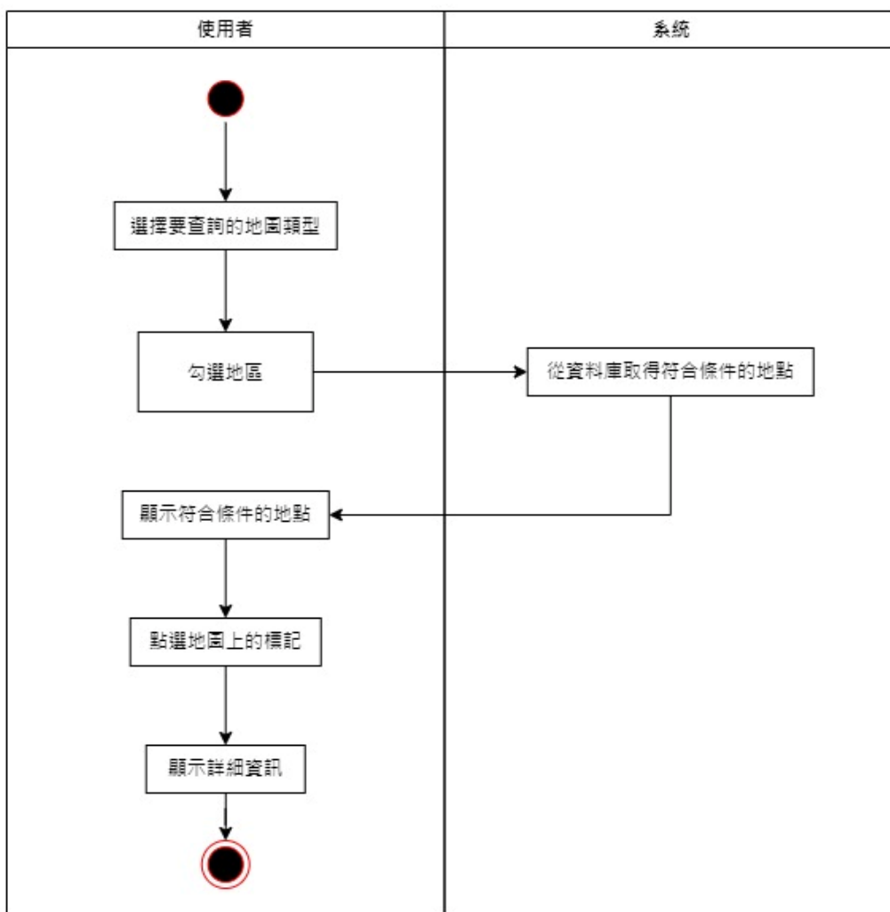
圖 5-3-6 查詢地圖活動圖
