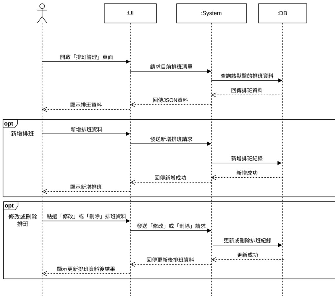
圖 6-1-8 獸醫排班管理循序圖
