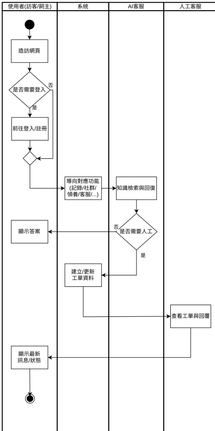
圖 5-3-11 AI 客服與人工客服接手活動圖
