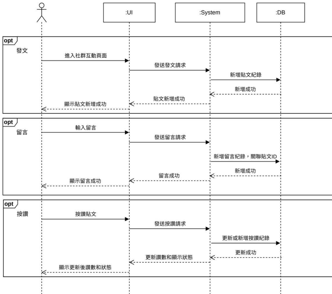
圖 6-1-11 社群互動循序圖
