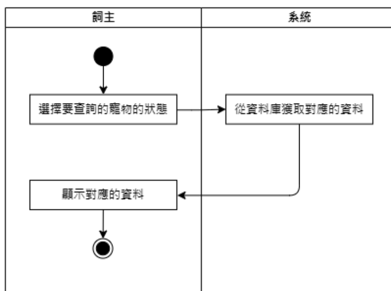
圖 5-3-17 查詢我的送養寵物活動圖
