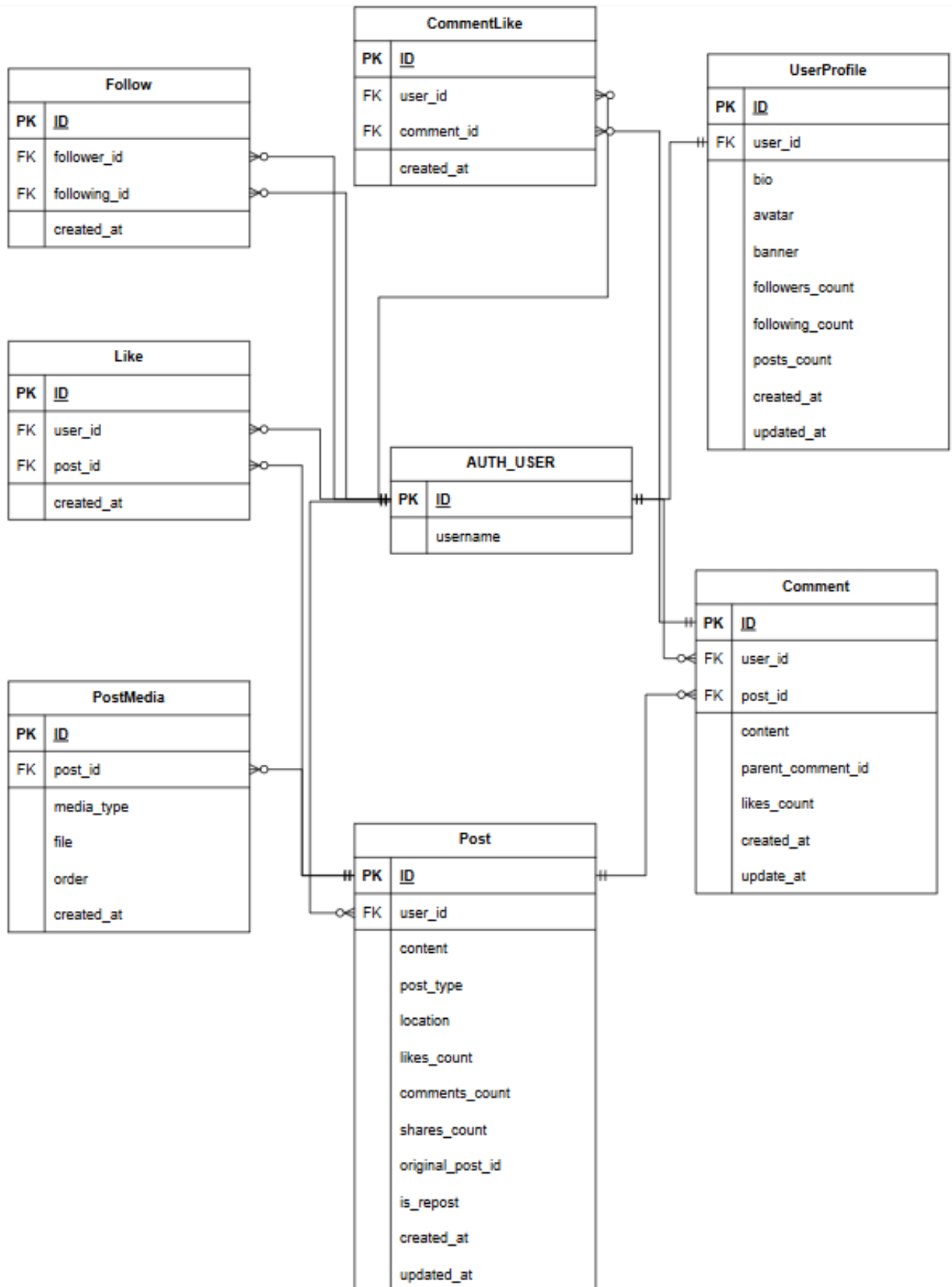
圖 8-1-6 資料庫關聯圖：社群
