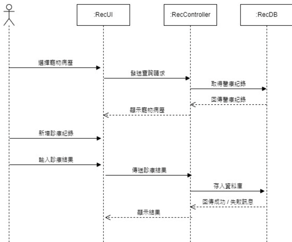
圖 6-1-7 獸醫看診循序圖
