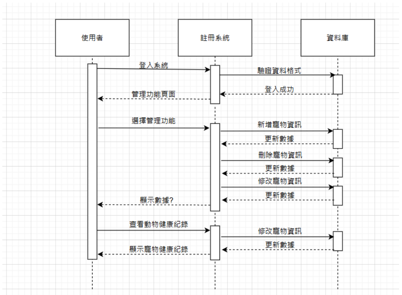
圖 6-1-9 系統管理循序圖
