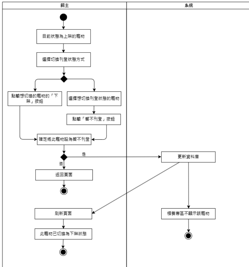
圖 5-3-19 切換為下架狀態活動圖
