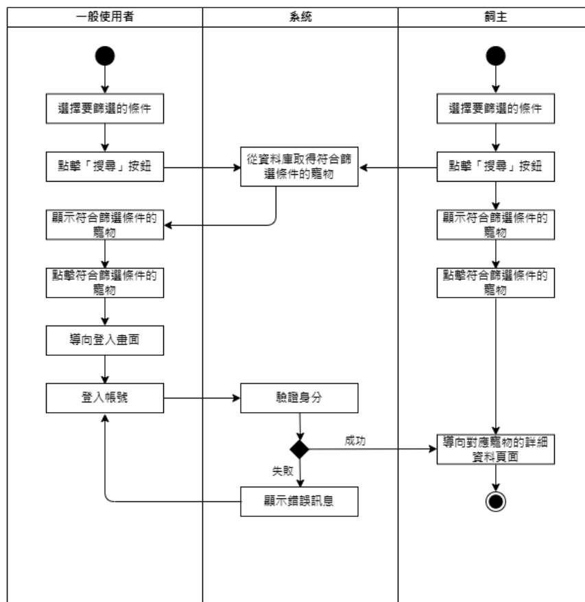
圖 5-3-16 搜尋寵物活動圖
