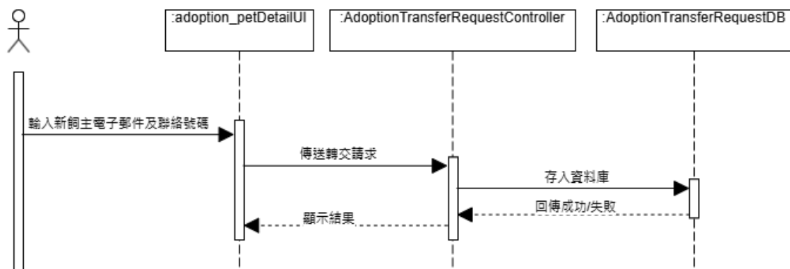
圖 6-1-16 轉交申請循序圖
