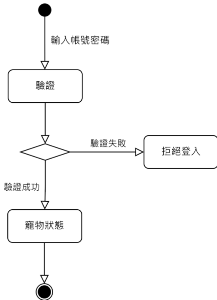
圖 7-4-1 狀態機
