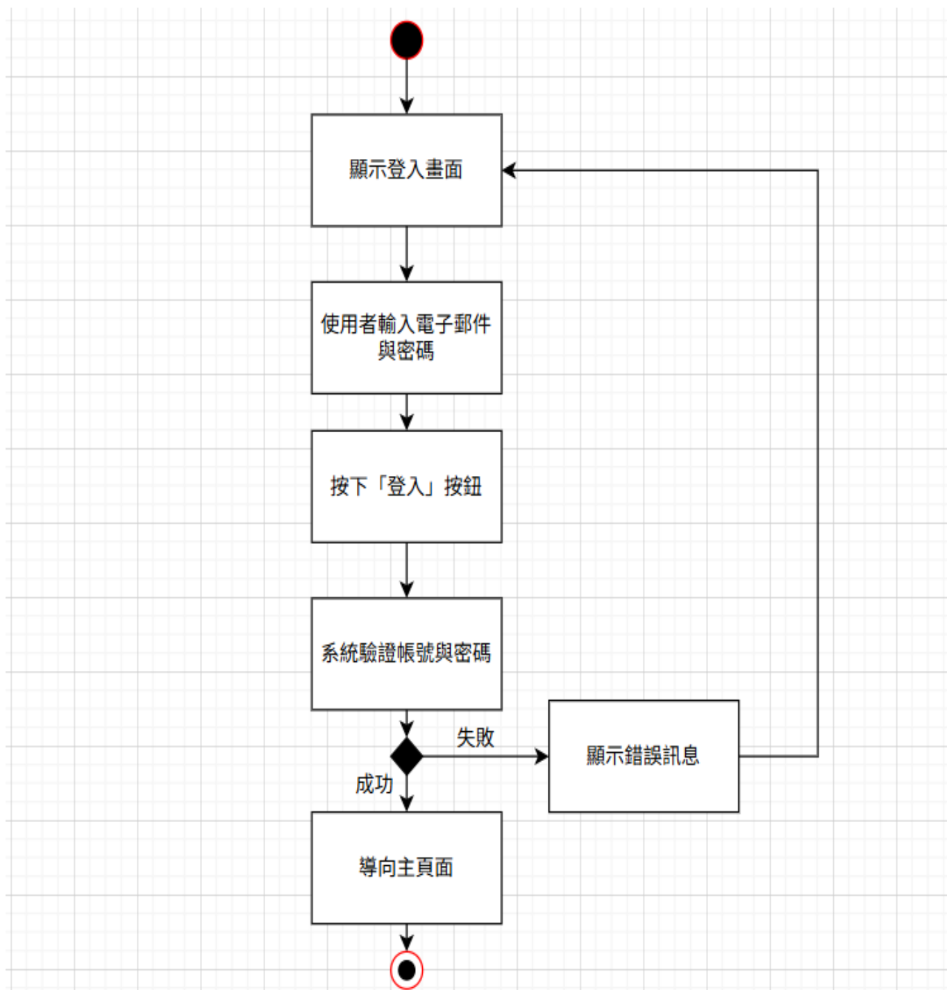
圖 5-3-3 登入活動圖
