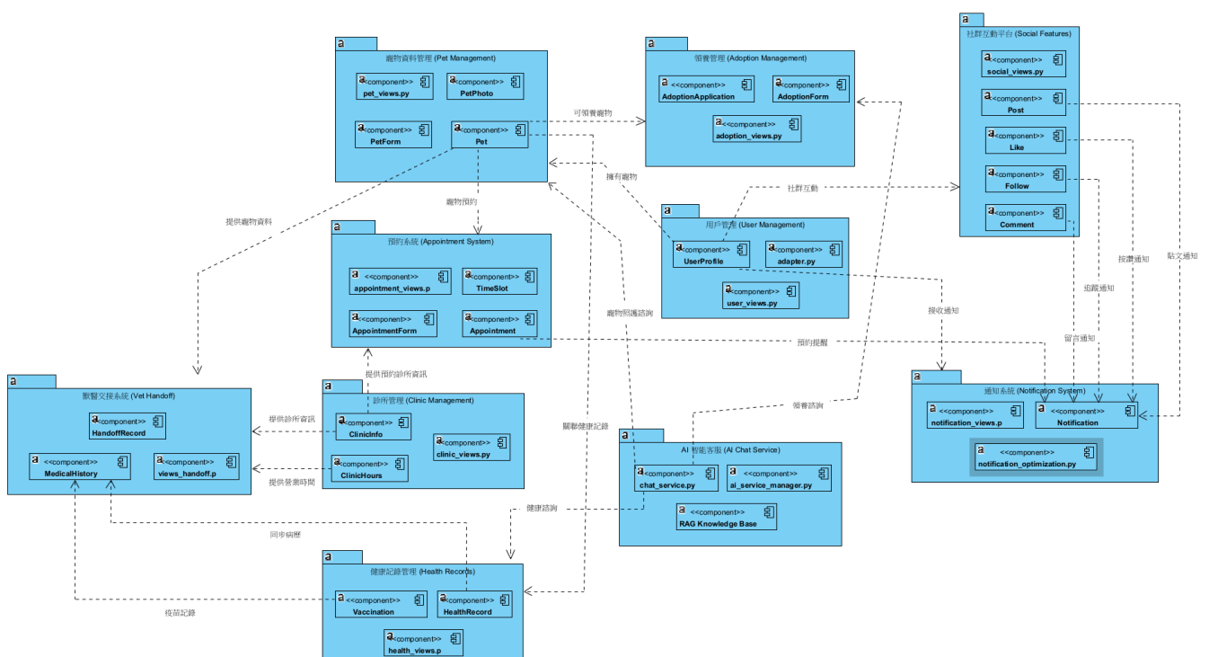
圖 7-2-1 套件圖
