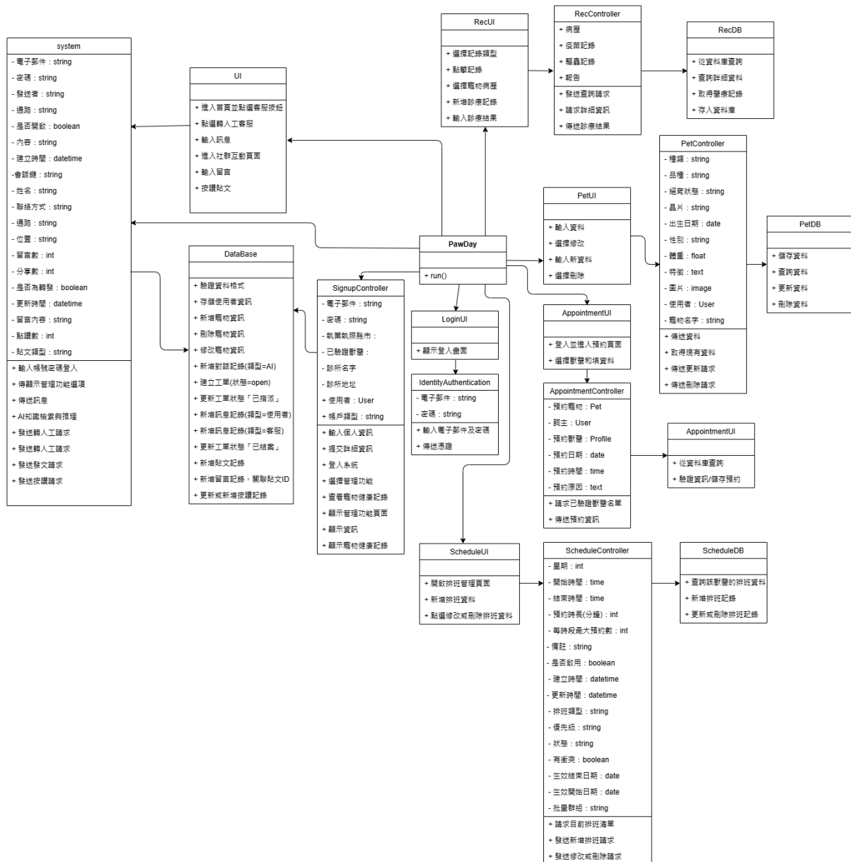
圖 6-2-1 設計類別圖-1
