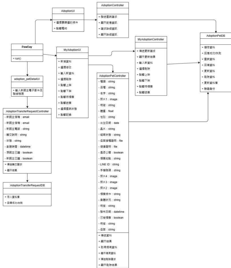
圖 6-2-2 設計類別圖-2
