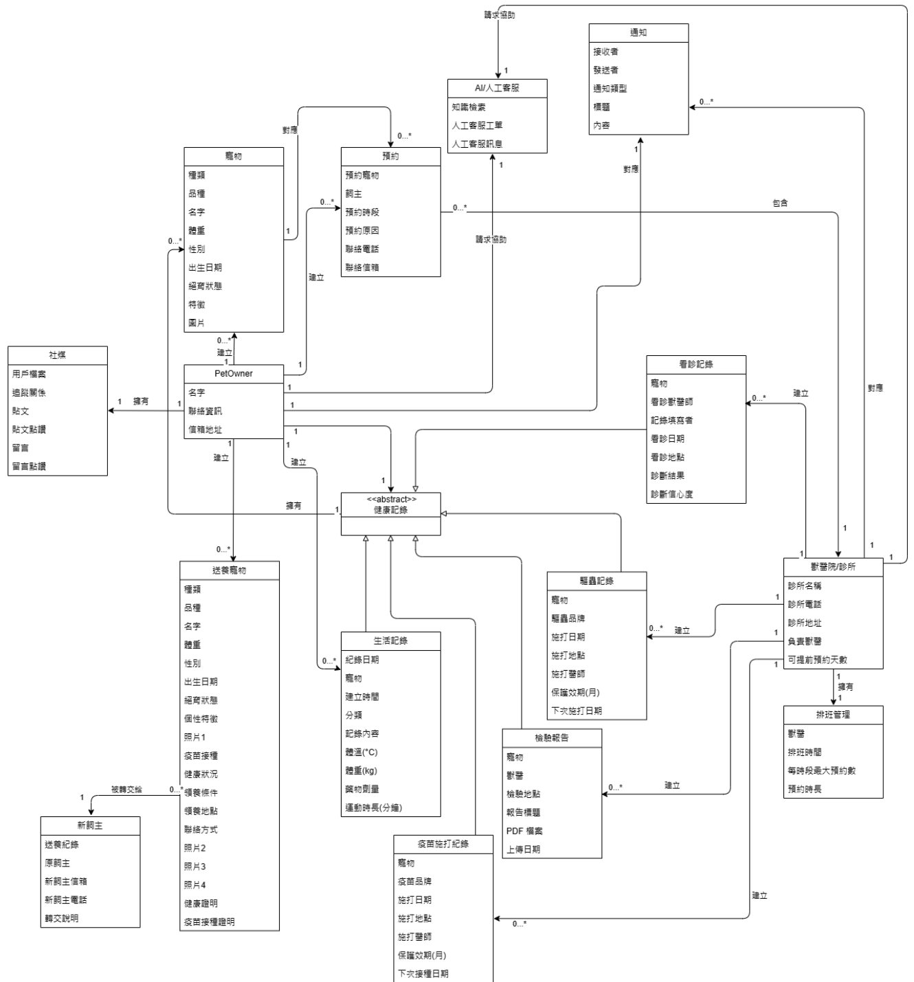
圖 5-4-1 分析類別圖
