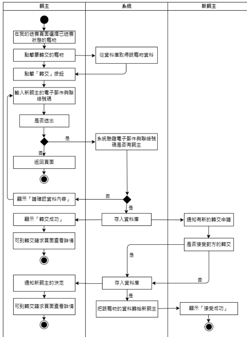
圖 5-3-22 轉交申請活動圖
