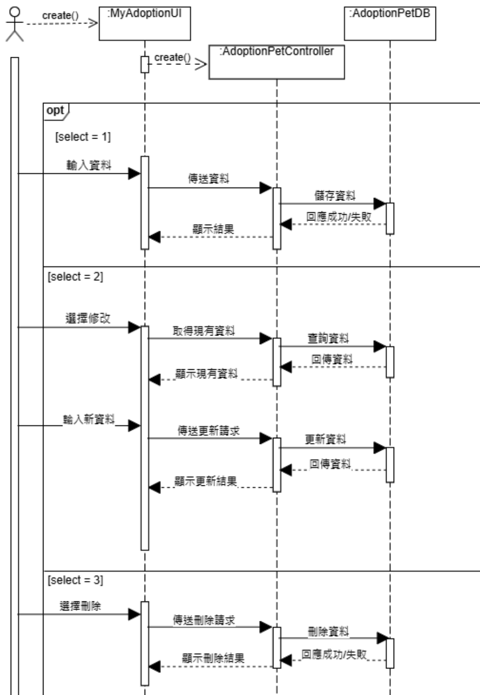
圖 6-1-12 領養專區寵物資料循序圖
