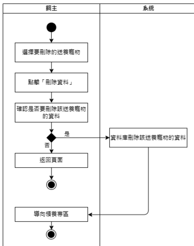
圖 5-3-15 刪除送養寵物資料活動圖
