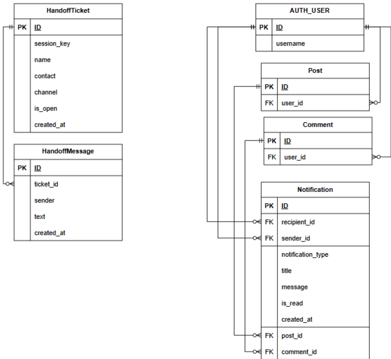
圖 8-1-7 資料庫關聯圖：客服與通知
