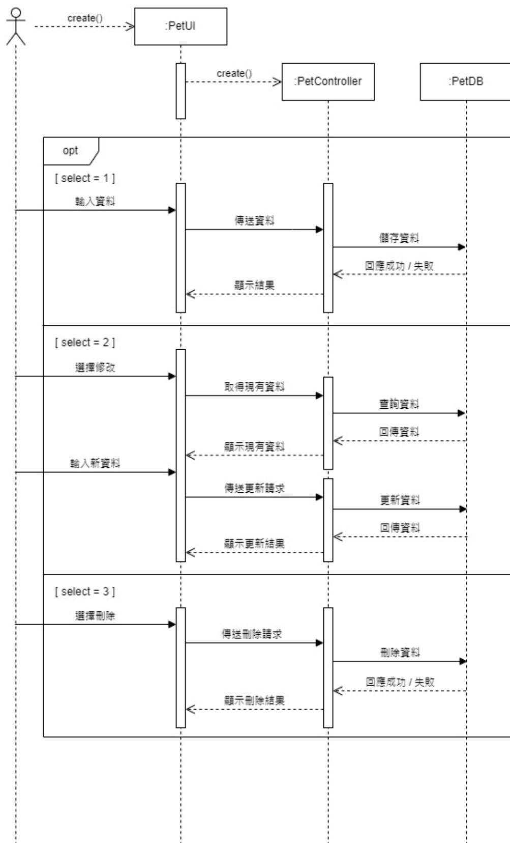
圖 6-1-3 新增寵物基本資料循序圖
