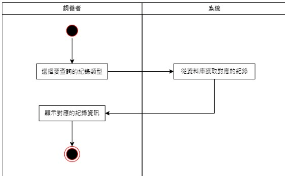
圖 5-3-5 查詢健康紀錄活動圖
