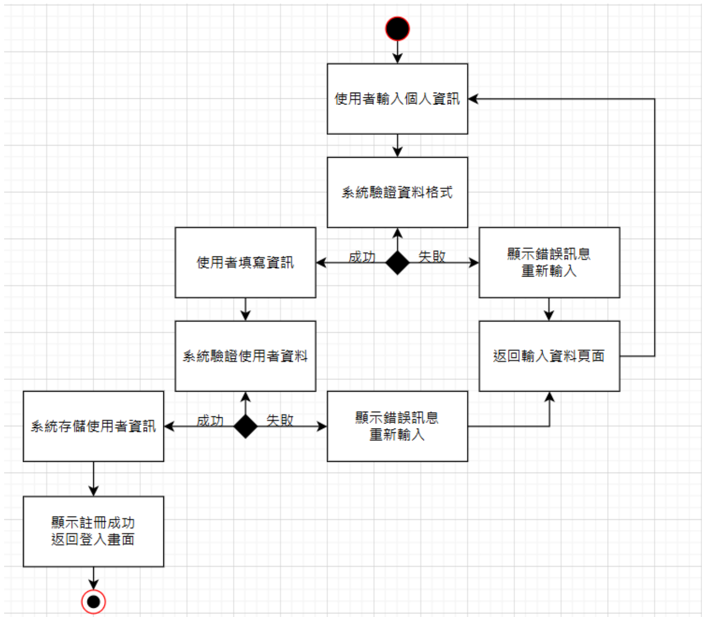
圖 5-3-2 註冊活動圖
