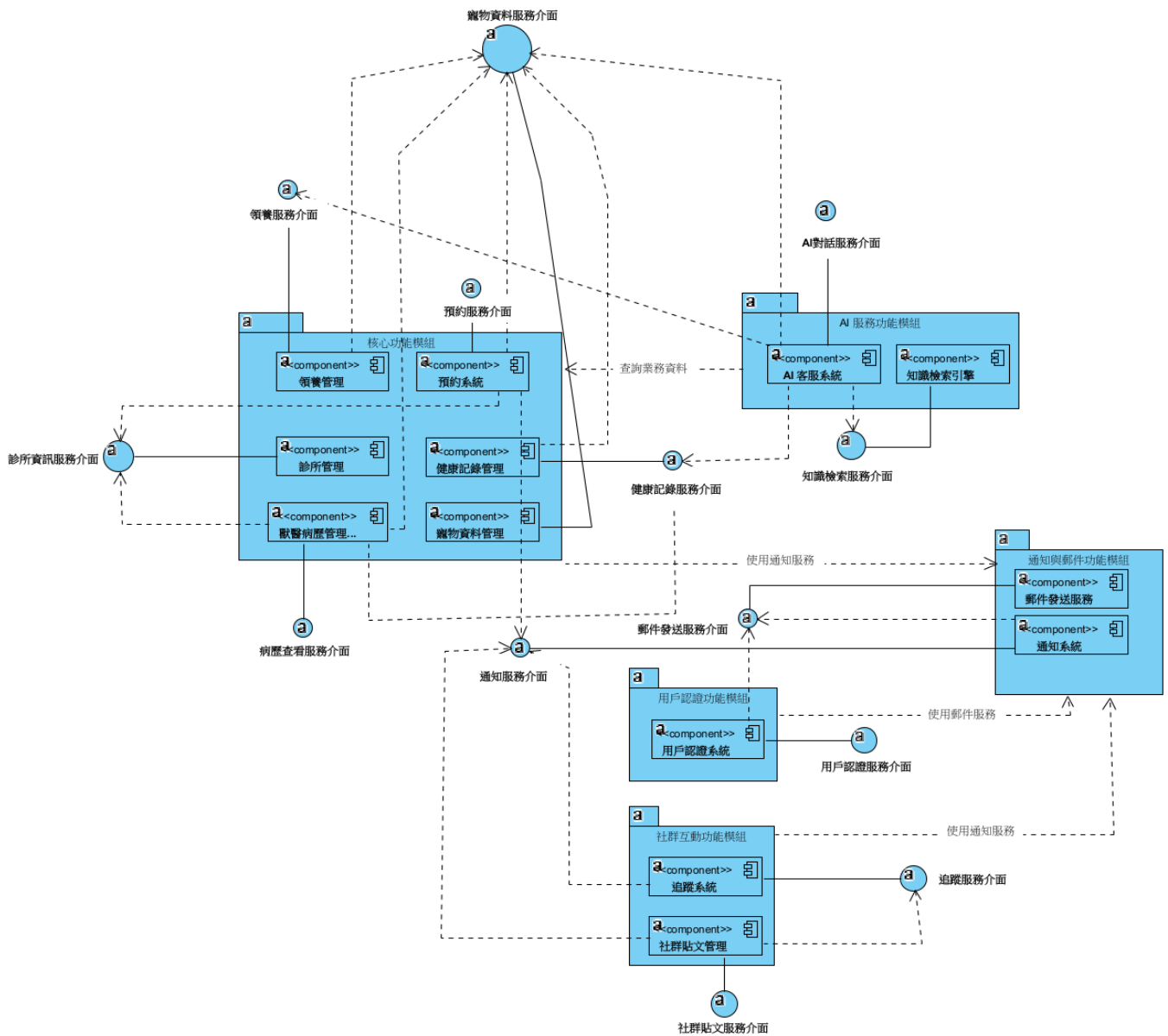
圖 7-3-1 元件圖
