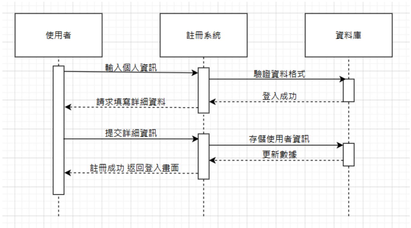
圖 6-1-1 註冊循序圖
