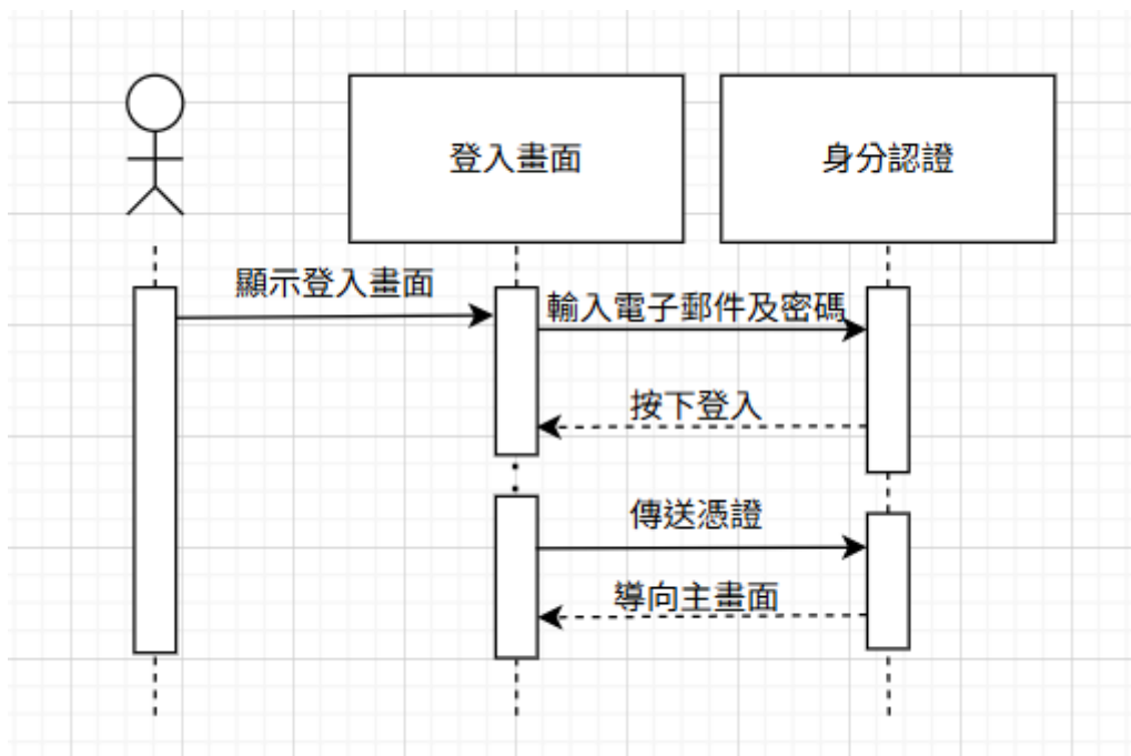
圖 6-1-2 登入循序圖
