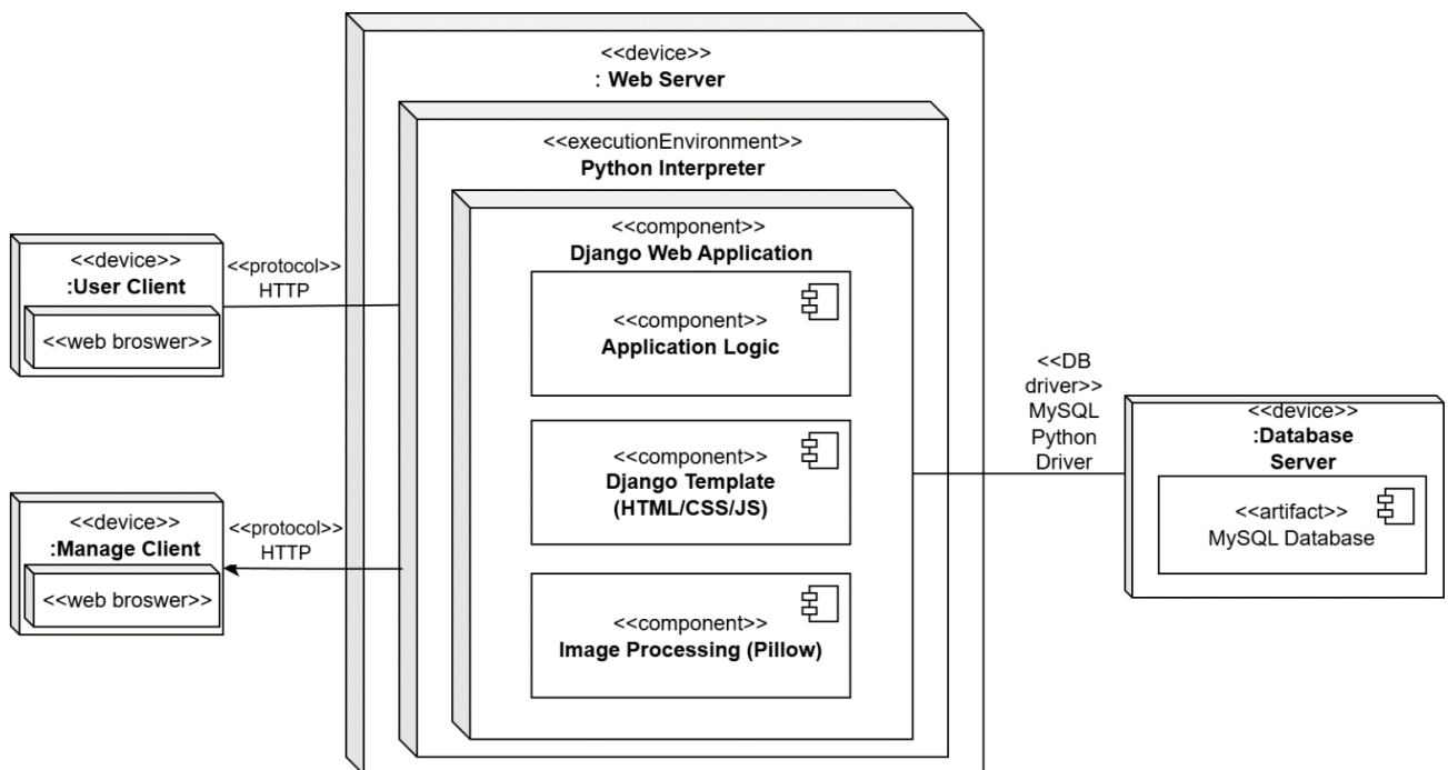
圖 7-1-1 佈署圖
