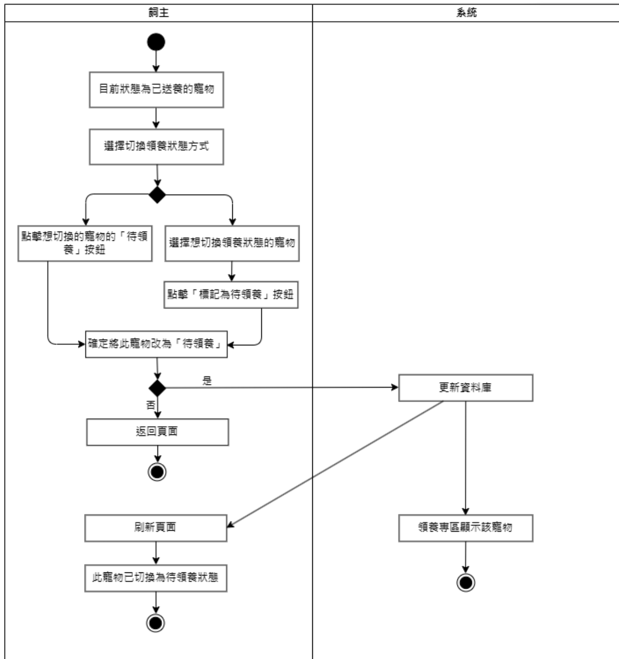
圖 5-3-21 切換為待領養狀態活動圖
