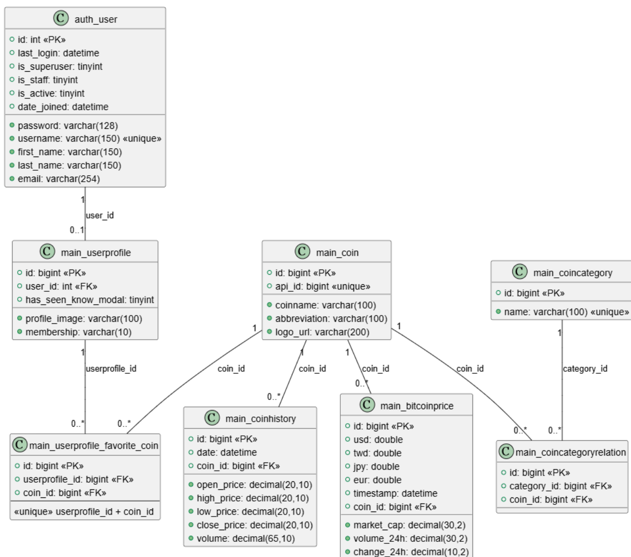
圖 5-4-1 分析類別圖(1)
