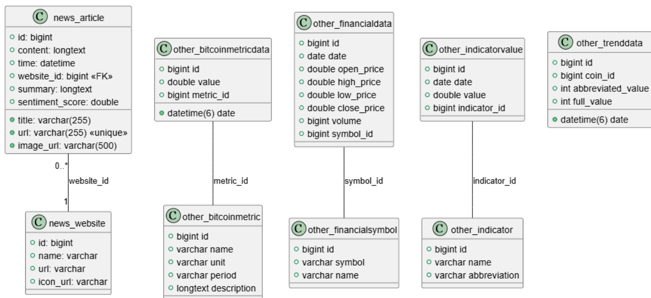
圖 5-4-2 分析類別圖(2)
