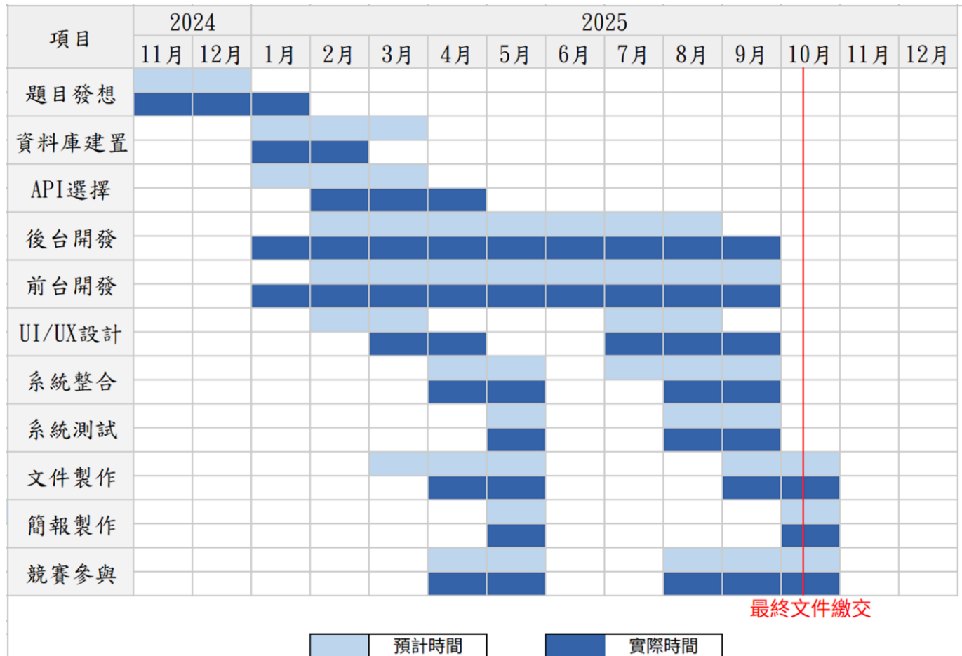
圖 4-1-1 甘特圖
