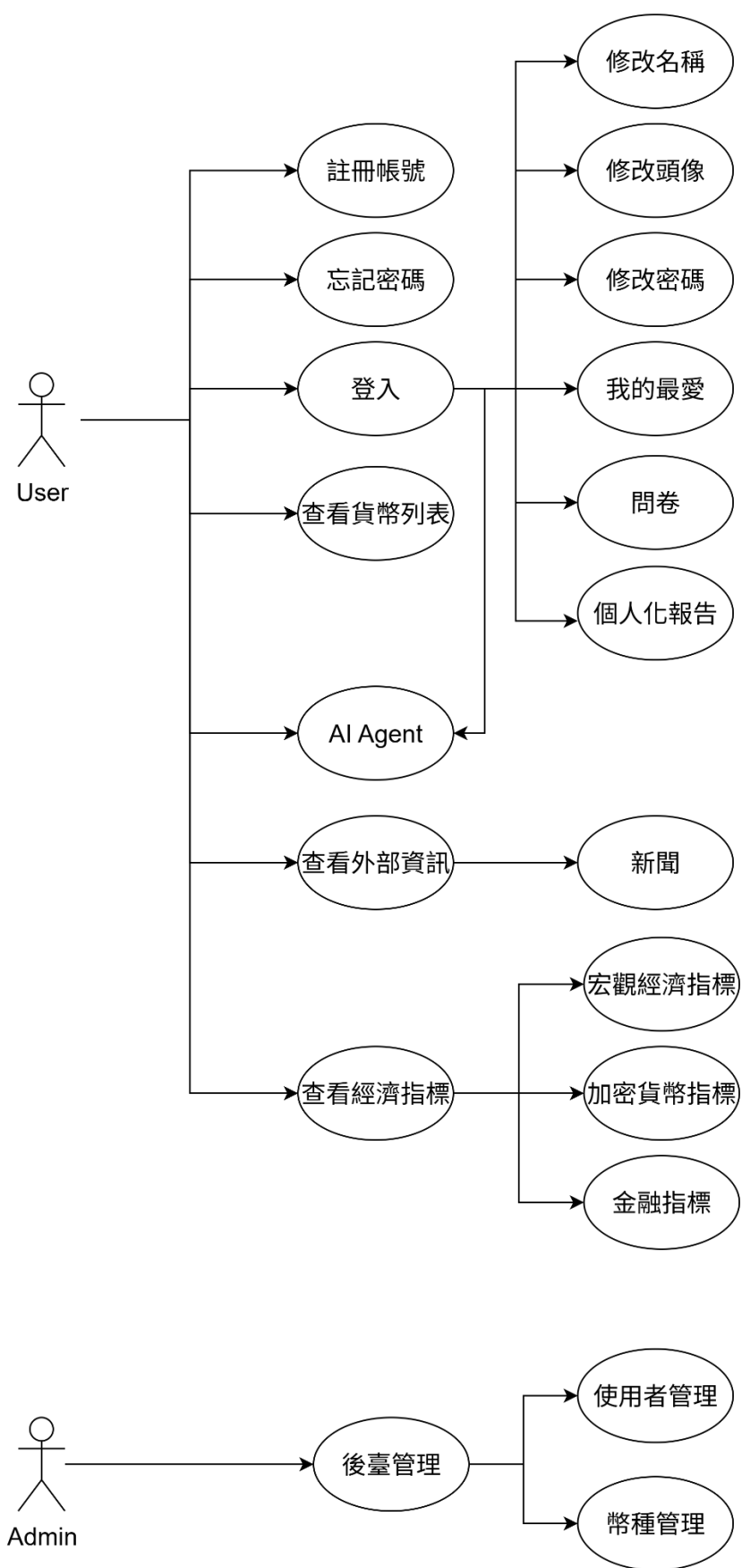
圖 5-2-1 使用個案圖
