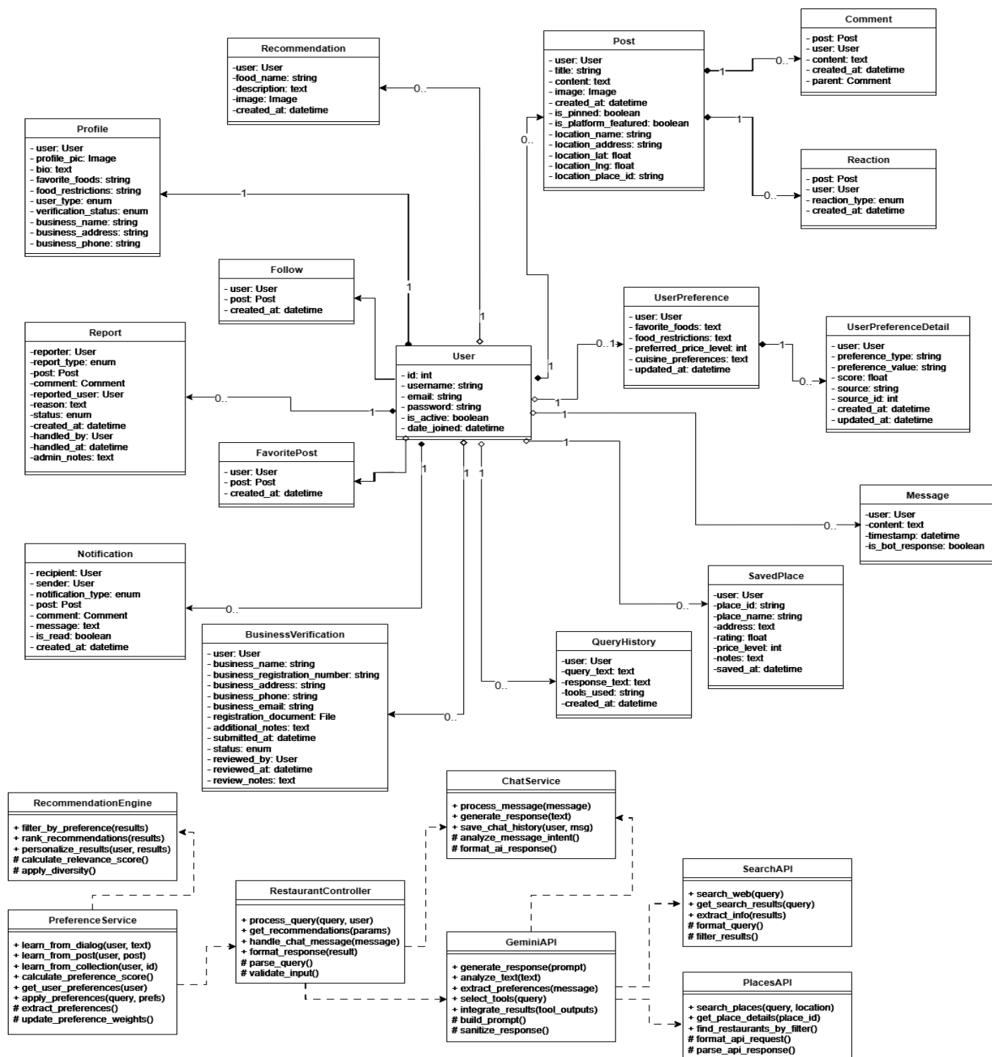
圖 5-4-1 分析類別圖
