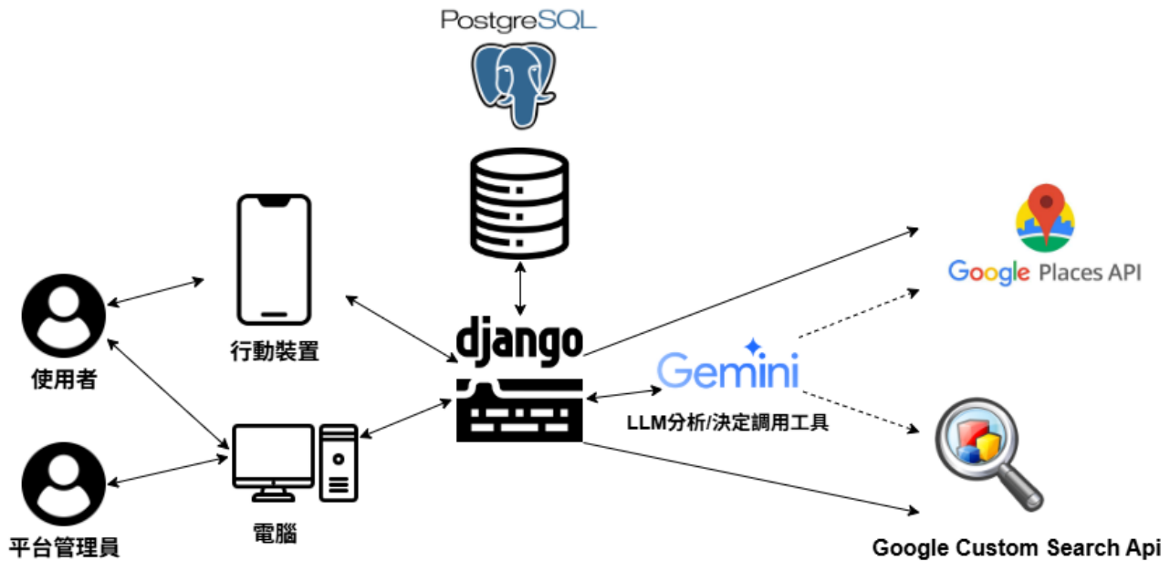
圖 3-1-1 系統架構圖
