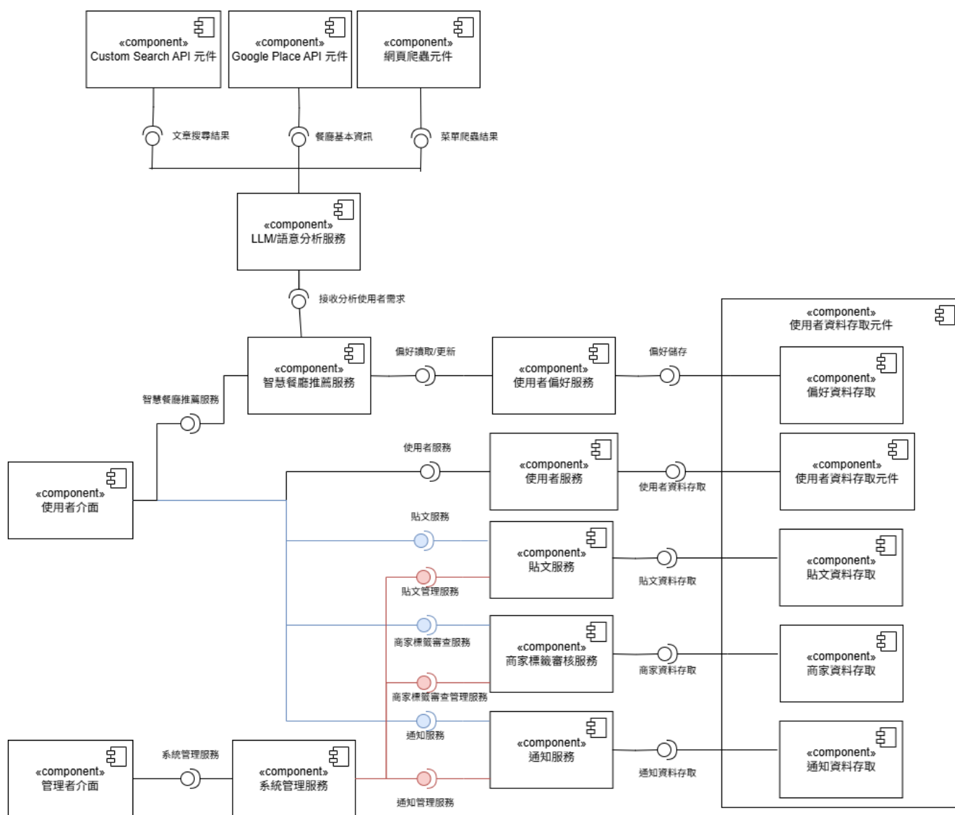
圖 7-3-1 套件圖
