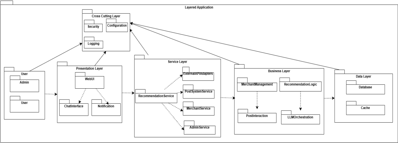
圖 7-2-1 套件圖
