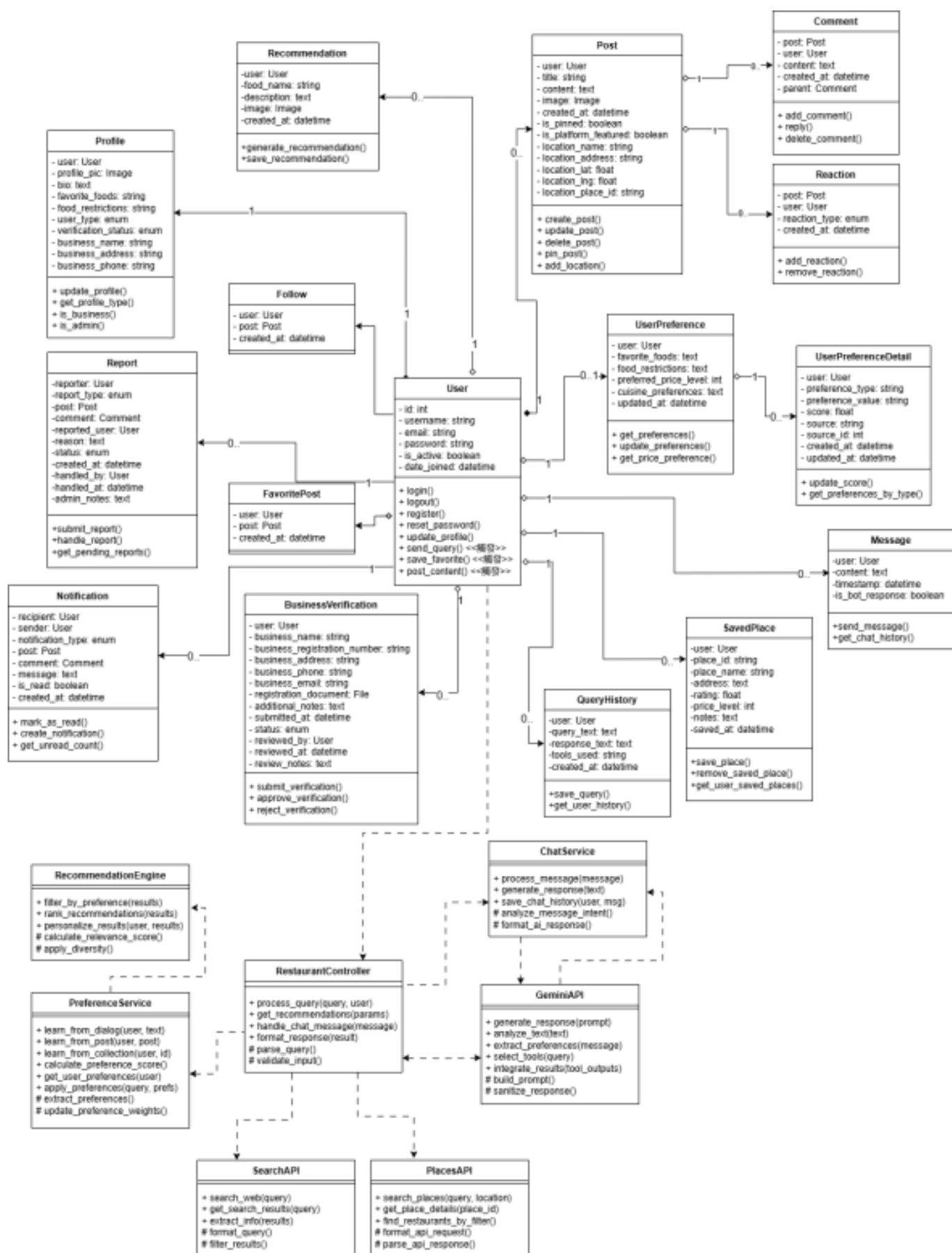
圖 6-2-1 設計類別圖
