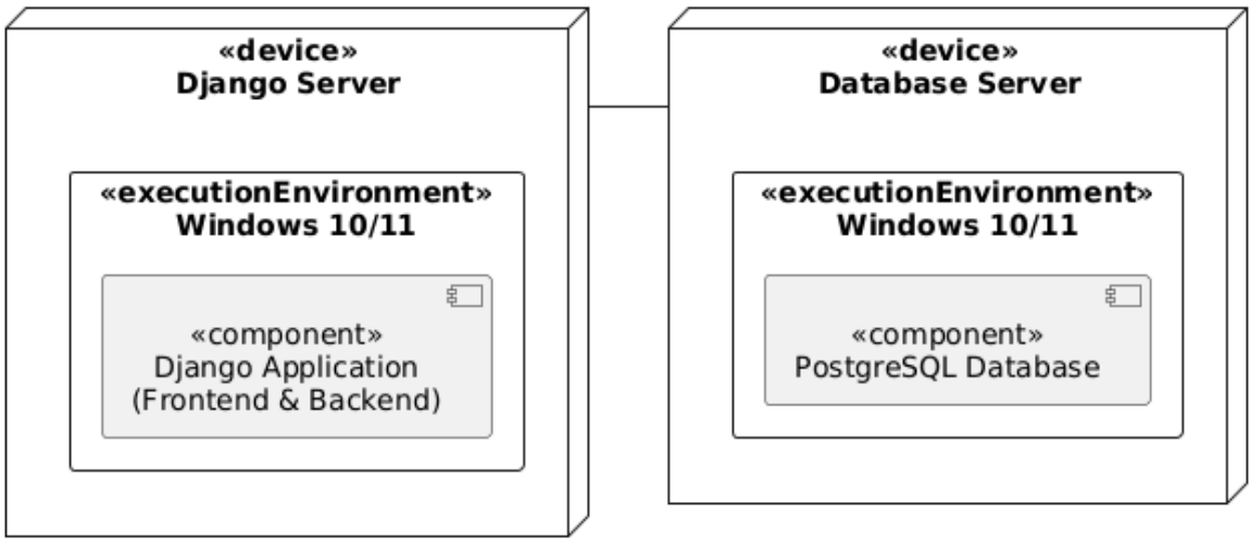
圖 7-1-1 佈署圖
