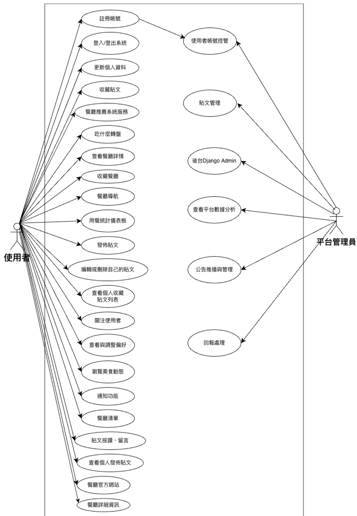
圖 5-2-1 使用個案圖
