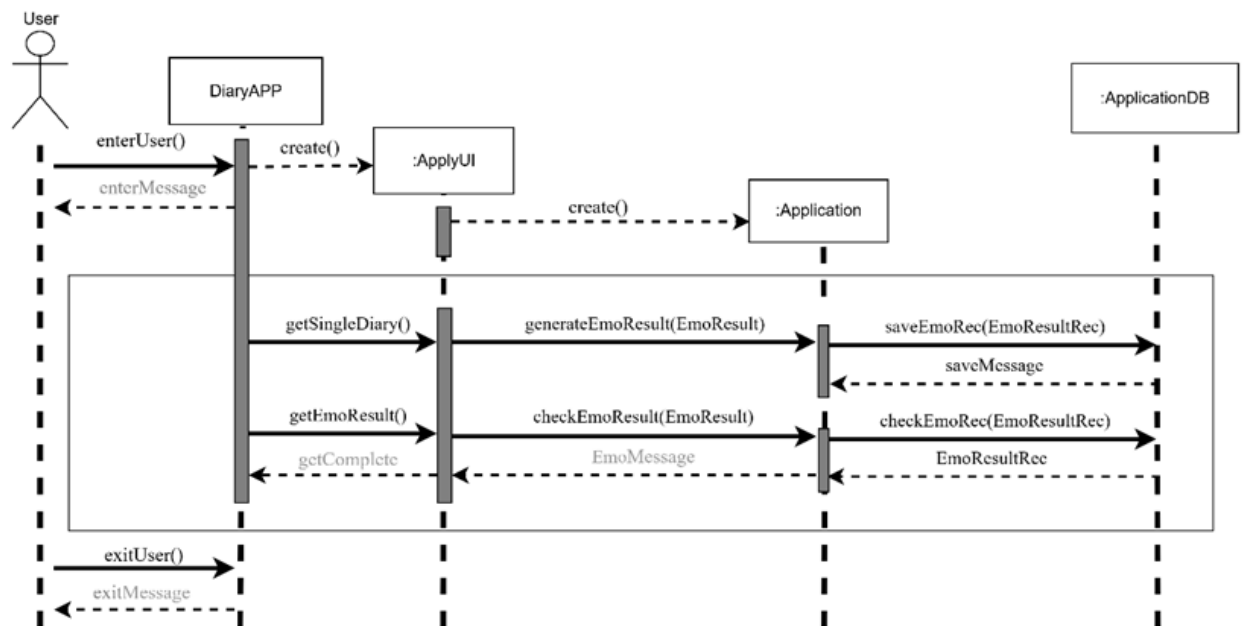
▲圖 6-1-4 「情緒分析」循序圖
