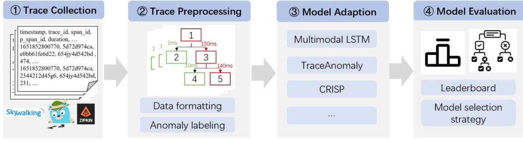
Fig. 7. Evaluation Framework.
