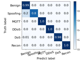
(c) CICIoMT2024
