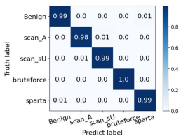
(b) MQTT-IoT-IDS2020
