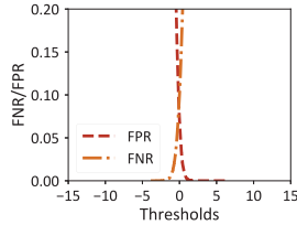
Fig. 7. FPR/FNR under NF-UNSW-NB15-v2.
