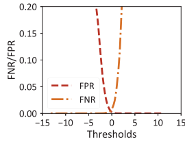
Fig. 6. FPR/FNR under NF-CSE-CIC-IDS2018-v2.
