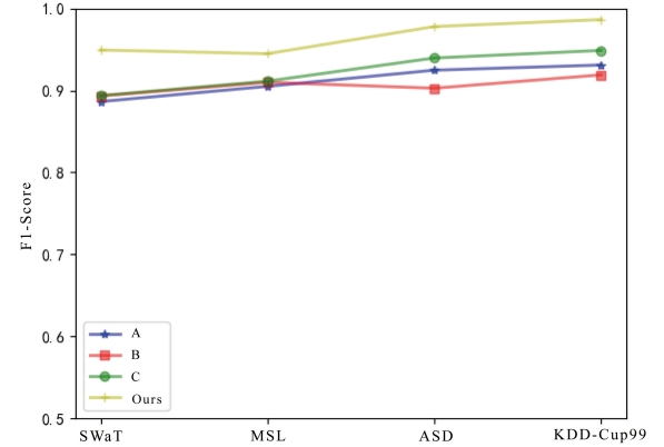
Fig. 8. F1 Score of model ablation experiment
