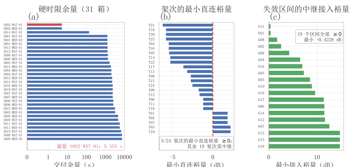
图 7.5 通信与硬时限的最小裕量
