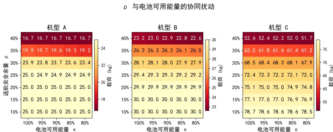
图 9.3 返航安全余量与电池可用能量的协同扰动
