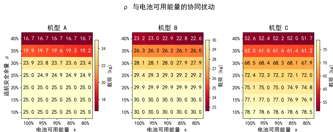
图 9.2 返航安全余量与电池可用能量的协同扰动
