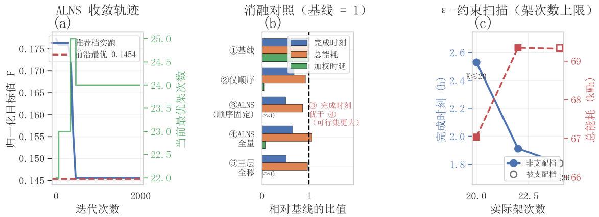
图 6.2 ALNS 收敛、消融对照与 \epsilon -约束扫描
