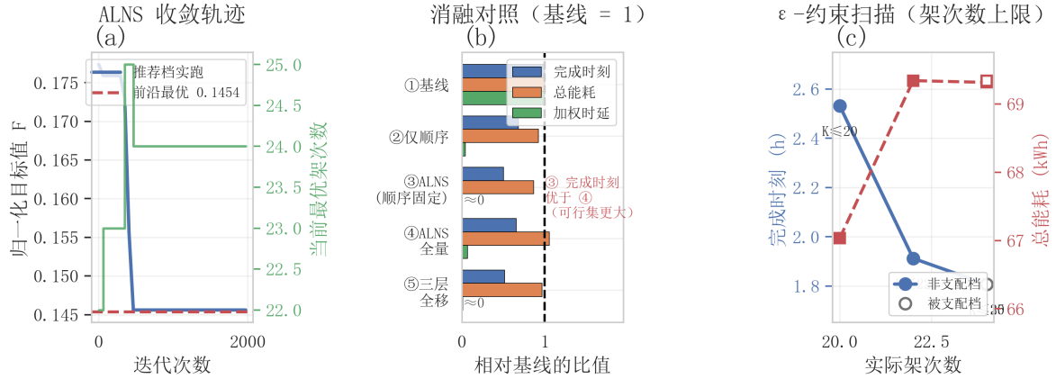
图 6.2 ALNS 收敛、消融对照与 \epsilon -约束扫描
