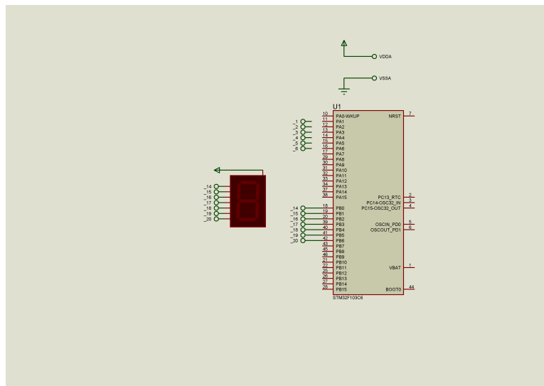
Hình 1.29: My Proteus schematic for Exercise 4
