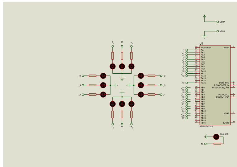
Hình 1.32: My Proteus schematic for Exercise 6
