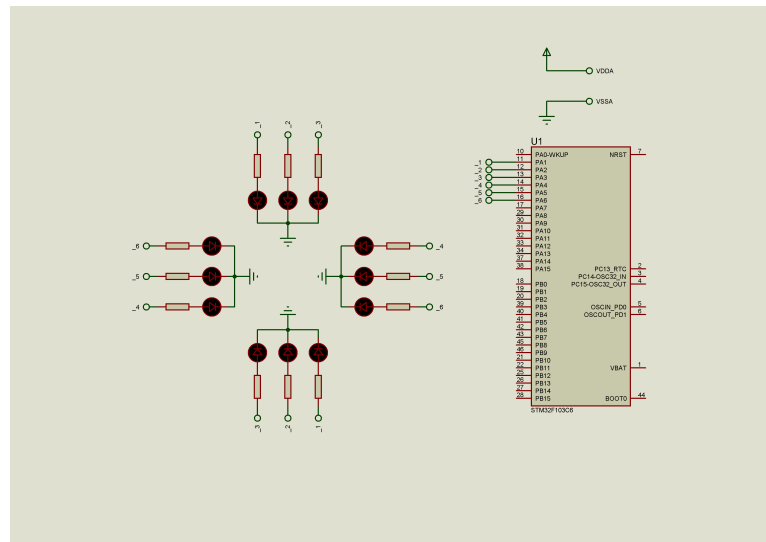
Hình 1.27: My Proteus schematic for Exercise 3
