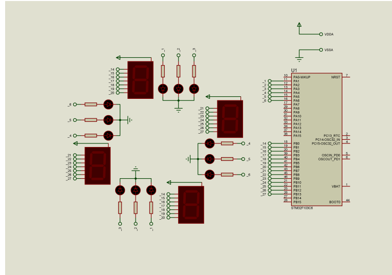
Hình 1.30: My Proteus schematic for Exercise 5
