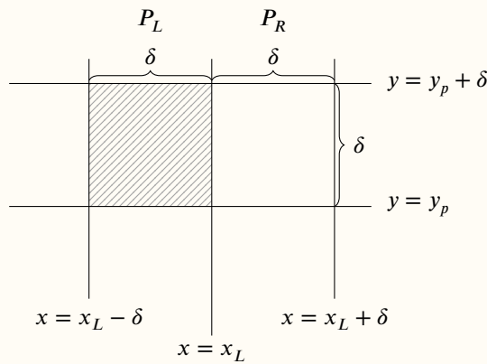
Rysunek 2: Prostokąt 2\delta \times \delta ograniczony prostymi y = y_p oraz y = y_p + \delta . Zacieniowany lewy kwadrat \delta \times \delta zawiera co najmniej 5 punktów z P .
