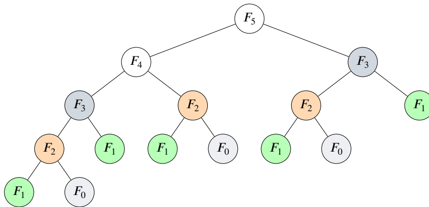
Rysunek 4: Drzewo wywołań rekurencyjnych FIB1(5). Wierzchołki o tym samym kolorze odpowiadają temu samemu podproblemowi, liczonemu wielokrotnie od zera: F_3 jest wyznaczane 2 razy, F_2 – 3 razy, a F_1 – 5 razy.
