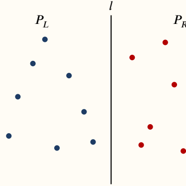
Rysunek 1: Podział zbioru P pionową prostą l na podzbiory P_L (na lewo) i P_R (na prawo) o rozmiarach |P_L| = \left\lceil \frac{|P|}{2} \right\rceil oraz |P_R| = \left\lfloor \frac{|P|}{2} \right\rfloor .
