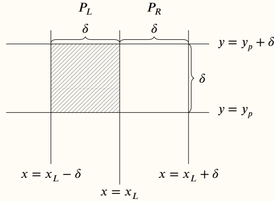
Rysunek 2: Prostokąt 2\delta \times \delta ograniczony prostymi y = y_p oraz y = y_p + \delta . Zaciemniony lewy kwadrat \delta \times \delta zawiera co najmniej 5 punktów z P .
