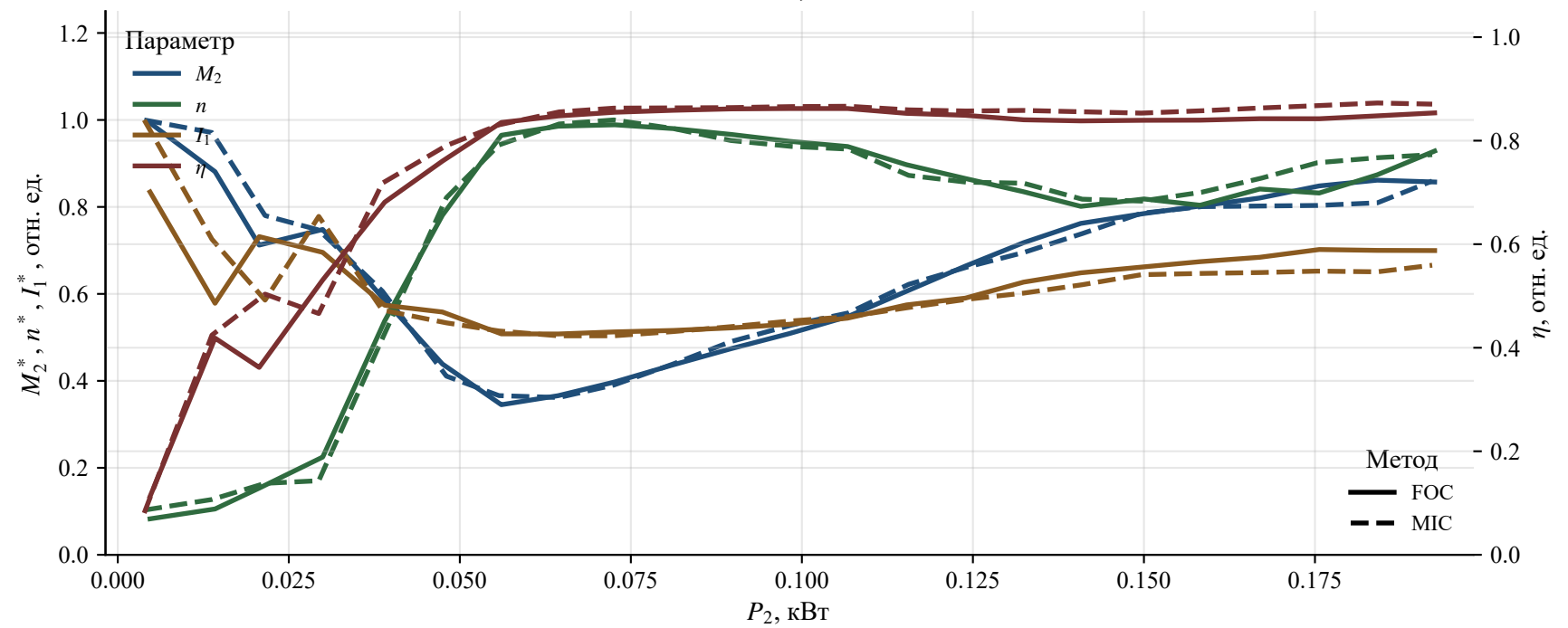
АИР56 0,25 кВт
