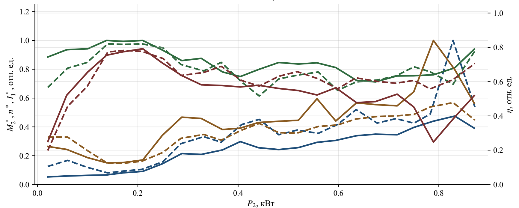
АО2-32-4 3,0 кВт
