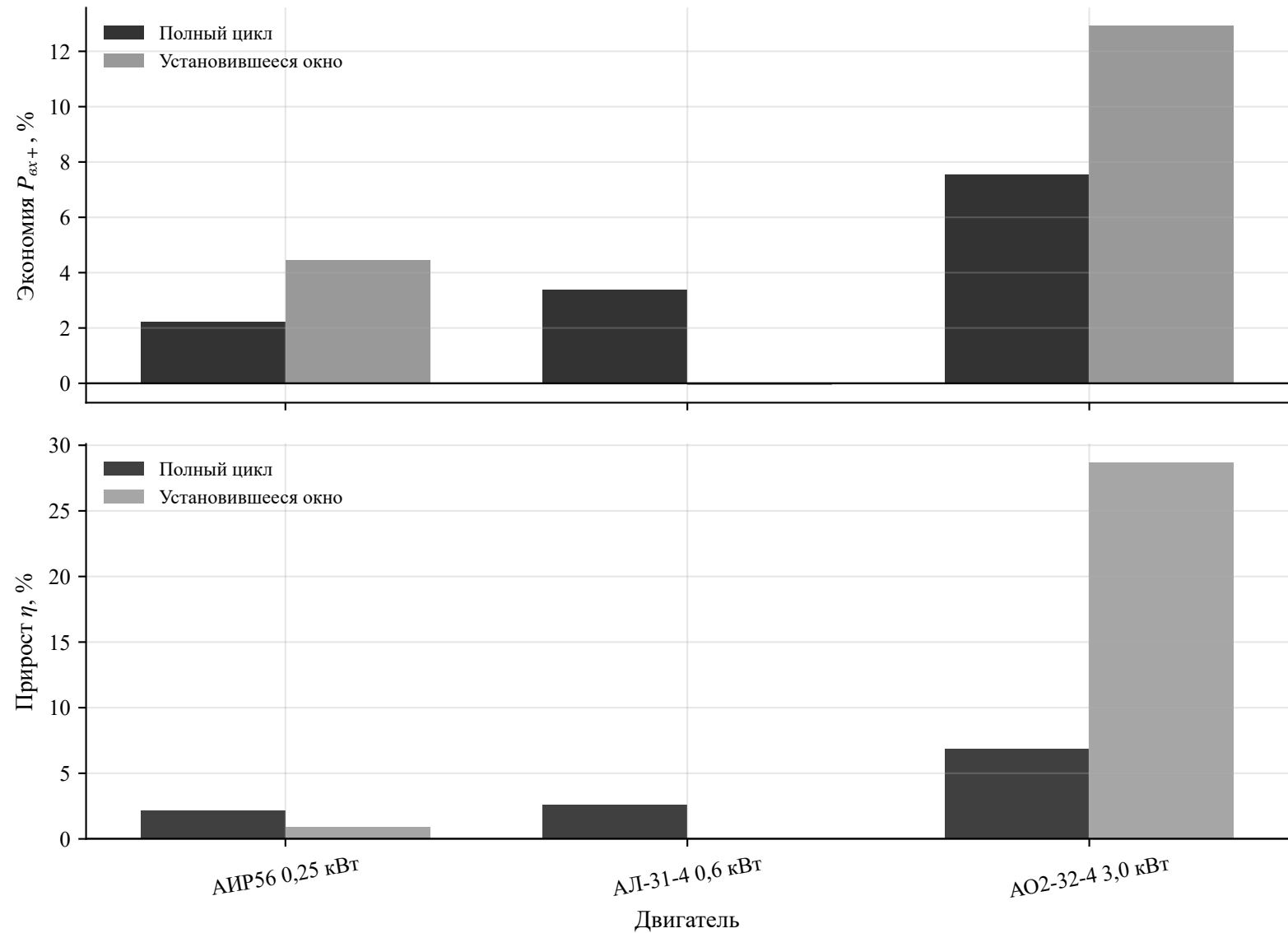
Сравнение FOC и MIC AI по экономии входной мощности
