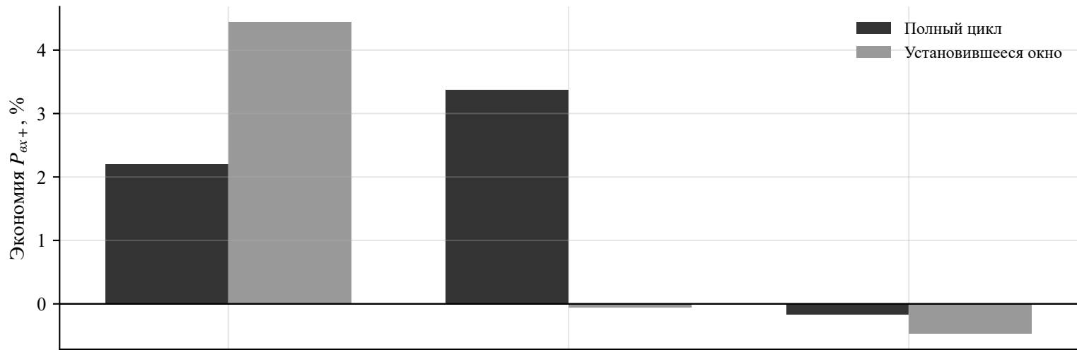
Сравнение FOC и MIC AI по экономии входной мощности
