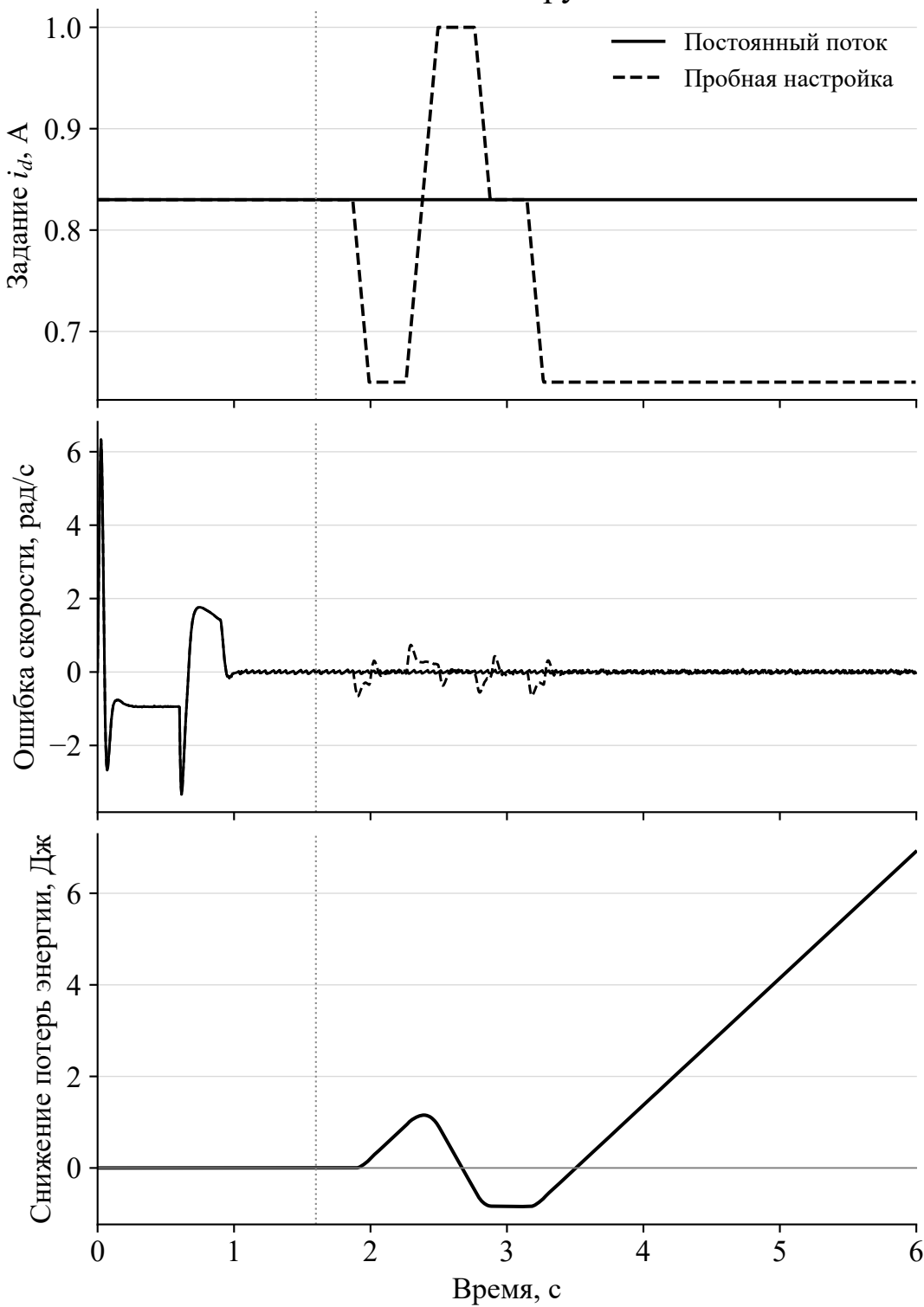
Постоянная нагрузка 25 %
