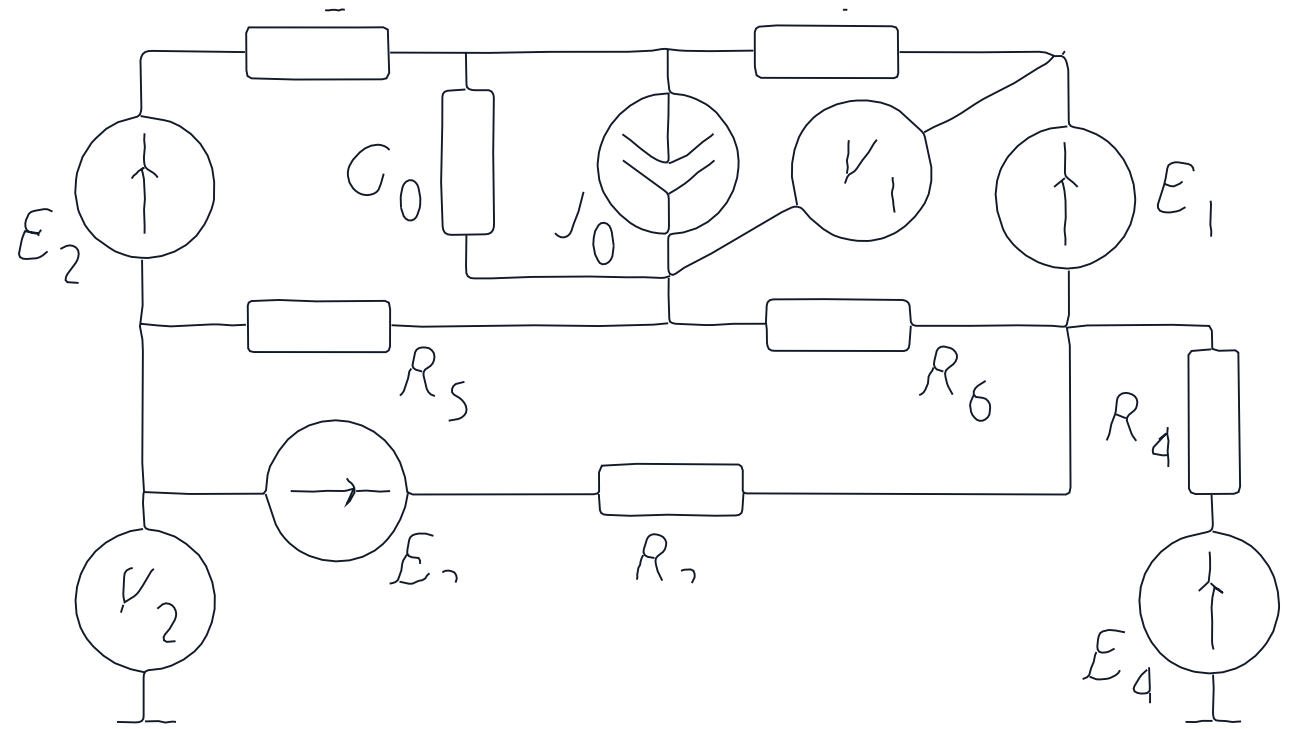
Рисунок 1.1 - Схема для определения потенциалов внешнего контура
