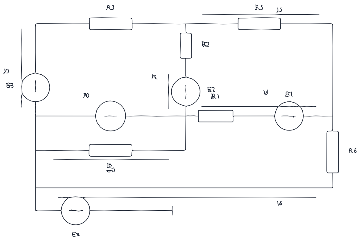
Рисунок 1.11 - Схема для определения потенциалов внешнего контура Потенциалы точек определены относительно выбранной точки заземления
