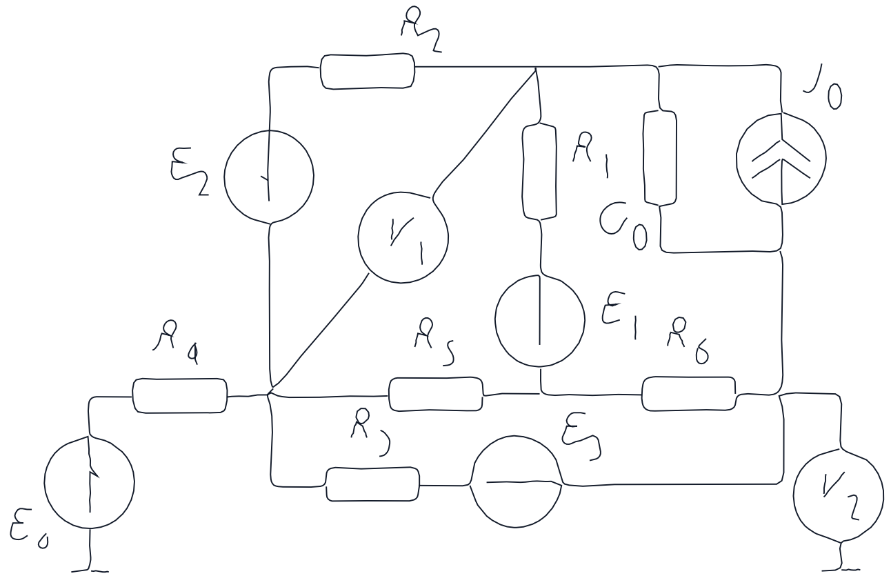
Рисунок 1.1 Схема для определения потенциалов внешнего контура Потенциалы точек определяем относительно выбранной точки заземления
