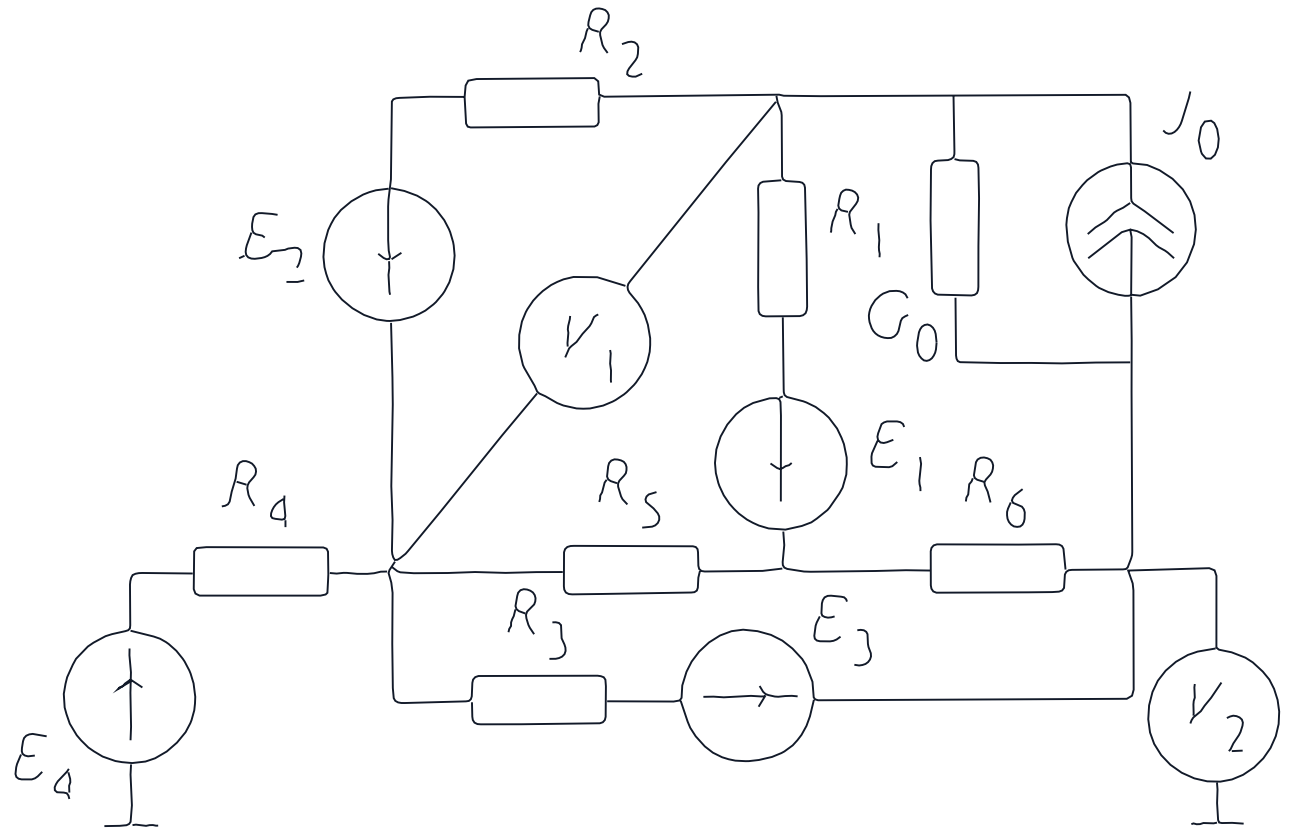
Рисунок 1.11 - Схема для определения потенциалов внешнего контура
