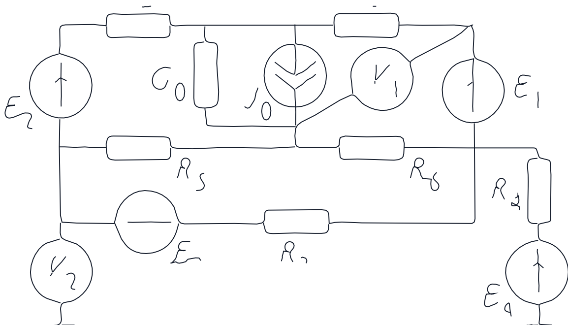
Рисунок 10а Схема для определения показаний вальстастров определен показаний по второму закону Кирхгофа
