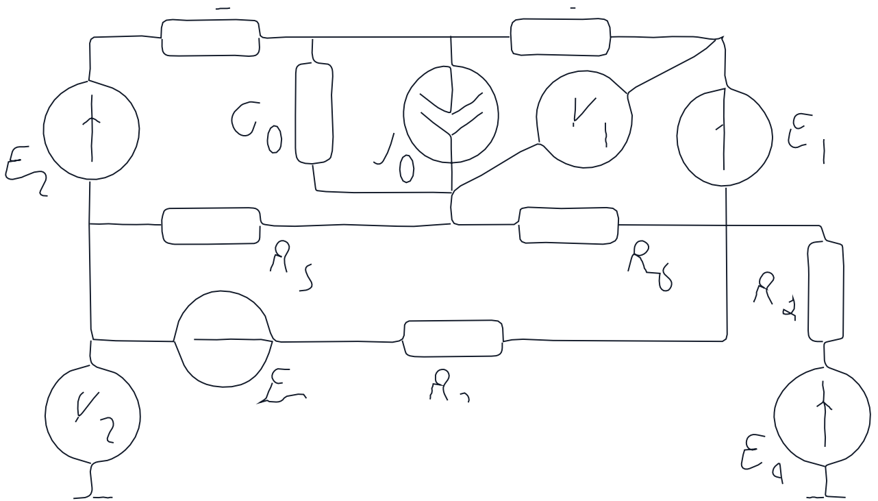
Рисунок 1 П-схема для определения потенциалов внешнего контура Потенциалы точек определяем относительно выбранной точки заземления
