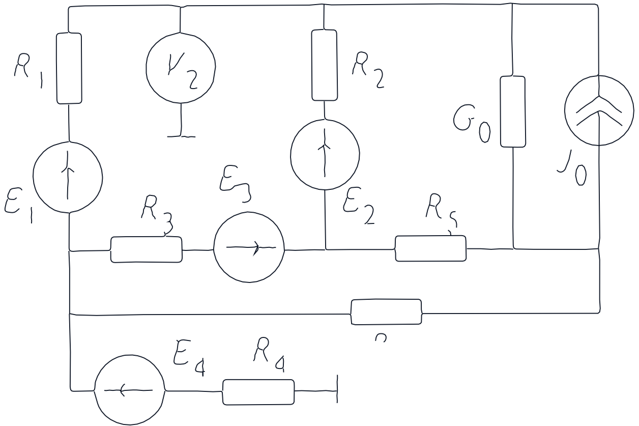
Рисунок 1.11 - Схема для определения потенциалов внешнего контура
