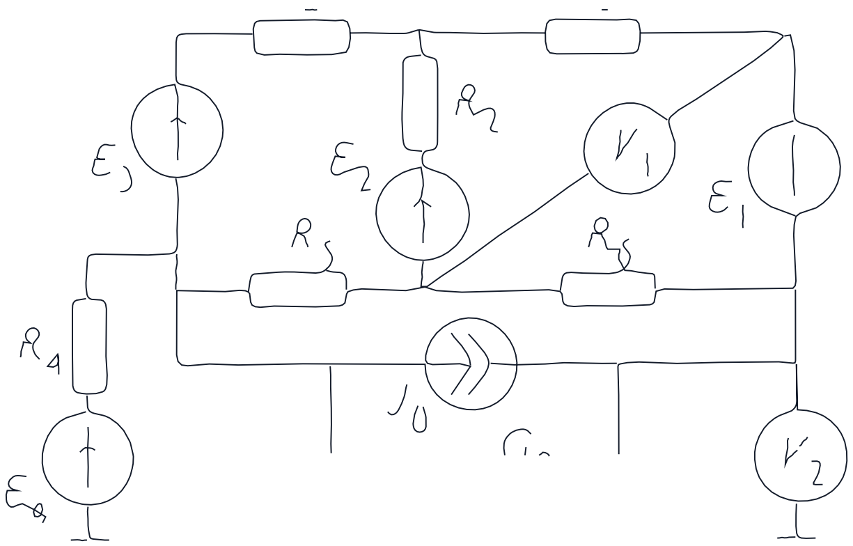
Рисунок 111 - Схема для определения потенциалов замкнутого контура Потенциалы точек определяем относительно выбранной точки заземления
