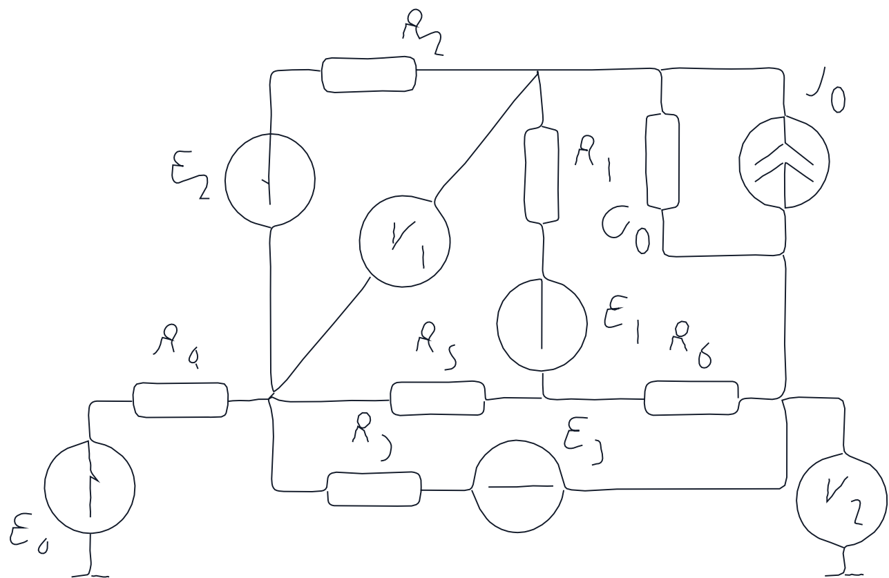
Рисунок I11 - Схема для определения потенциалов введенного контура Потенциалы точек определяем относительно выбранной точки заземления
