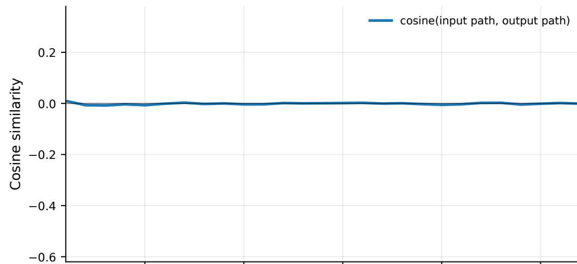
S4 input vocab LoRA
