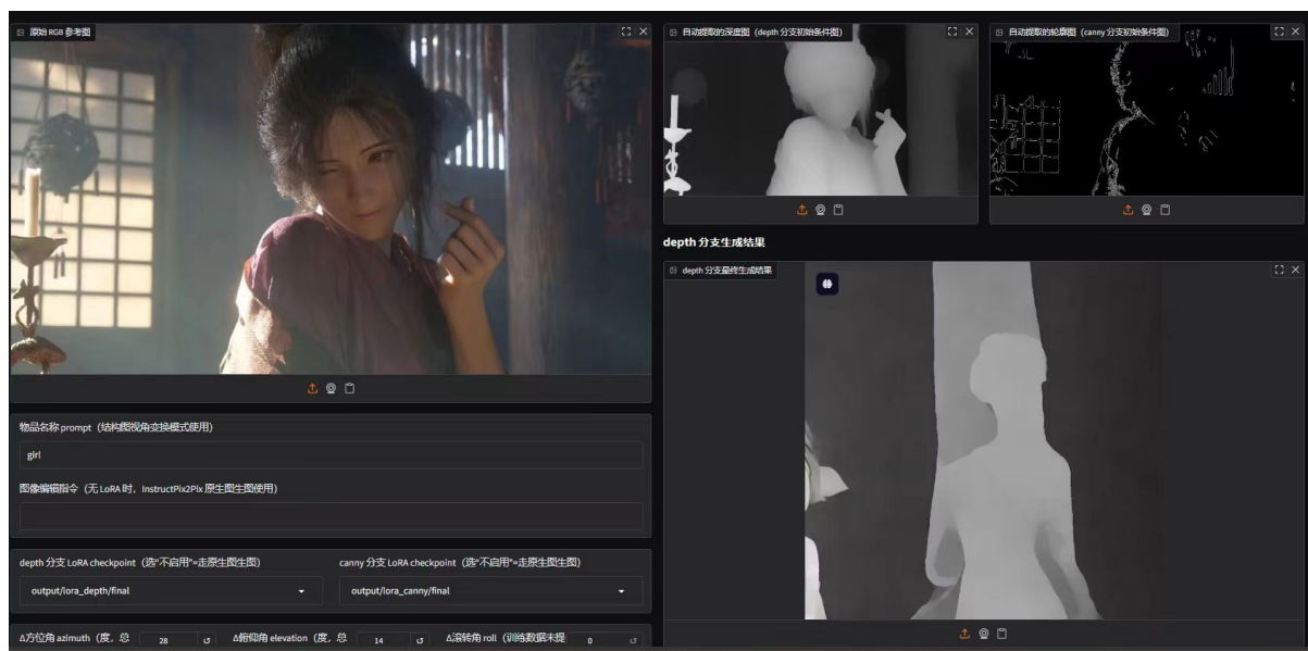
图 5.1: Gradio 推理调试界面。用户上传参考图后自动提取深度图与轮廓图, depth 与 canny 分支独立生成结果。
