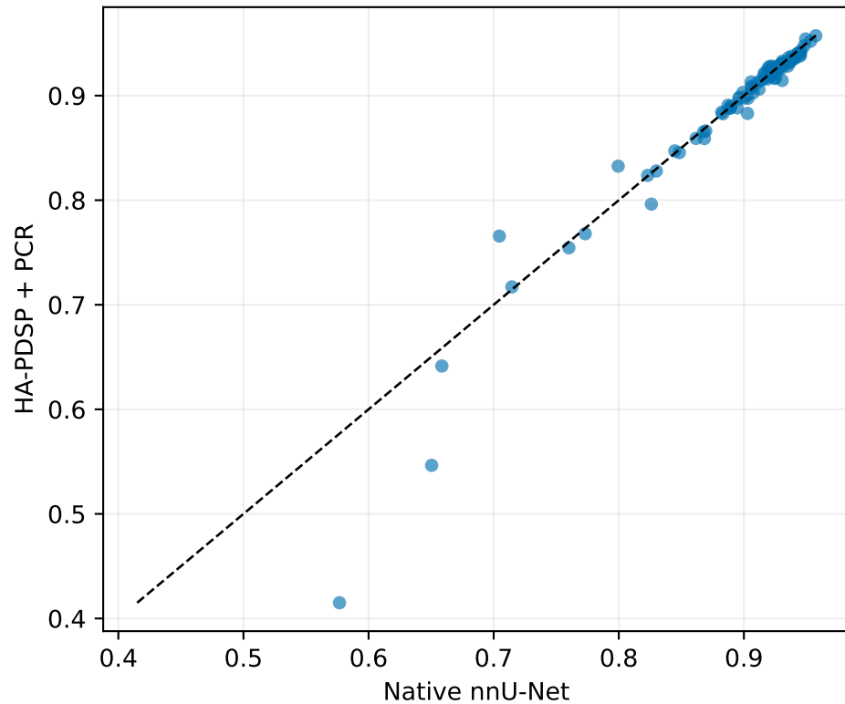
Dice
