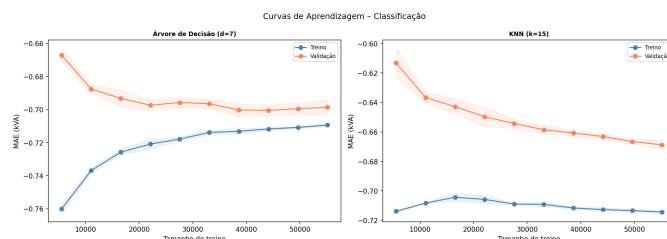
Fig. 7: Curvas de Aprendizagem dos modelos de classificação. A convergência entre as linhas de treino e validação permite diagnosticar o equilíbrio entre overfitting e underfitting .
