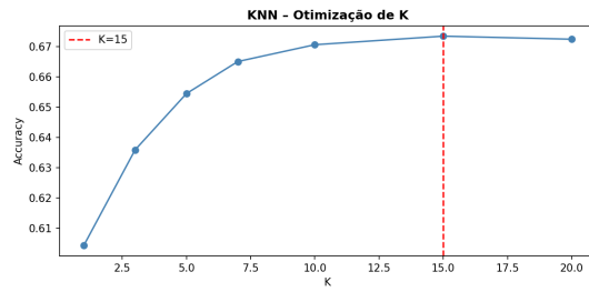
Fig. 3: Otimização do hiperparâmetro k no modelo KNN. A escolha do valor ideal é crucial para equilibrar o viés e a variância do modelo.
