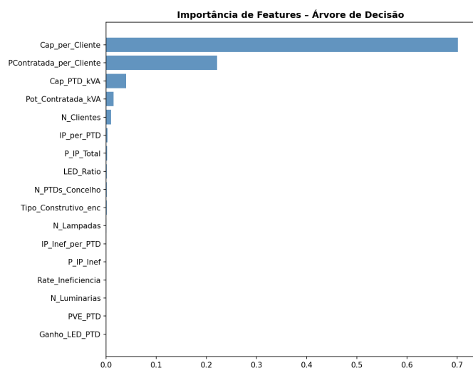
Fig. 5: Importância das características (Feature Importance) extraída do modelo de classificação baseado em árvores, destacando a relevância da capacidade instalada por cliente.
