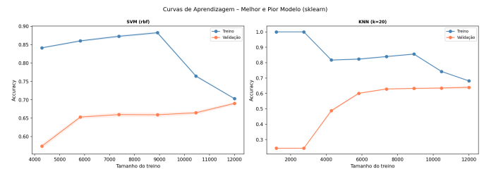
Fig. 7: Curvas de Aprendizagem dos modelos SVM (RBF) e KNN ( k = 20 ). O SVM mostra conversão eficiente sem overfitting persistente; o KNN atinge plateau prematuro e mantém gap treino/validação estável, indicando limitação estrutural do algoritmo.
