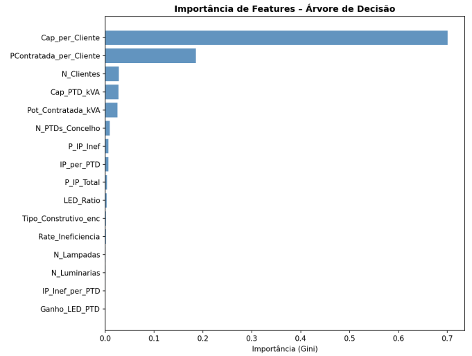
Fig. 6: Importância das variáveis na Árvore de Decisão ( Gini impurity ). Cap_per_Cliente e PContratada_per_Cliente concentram \approx 89\% da importância total; todas as variáveis de Iluminação Pública apresentam contributo residual.
