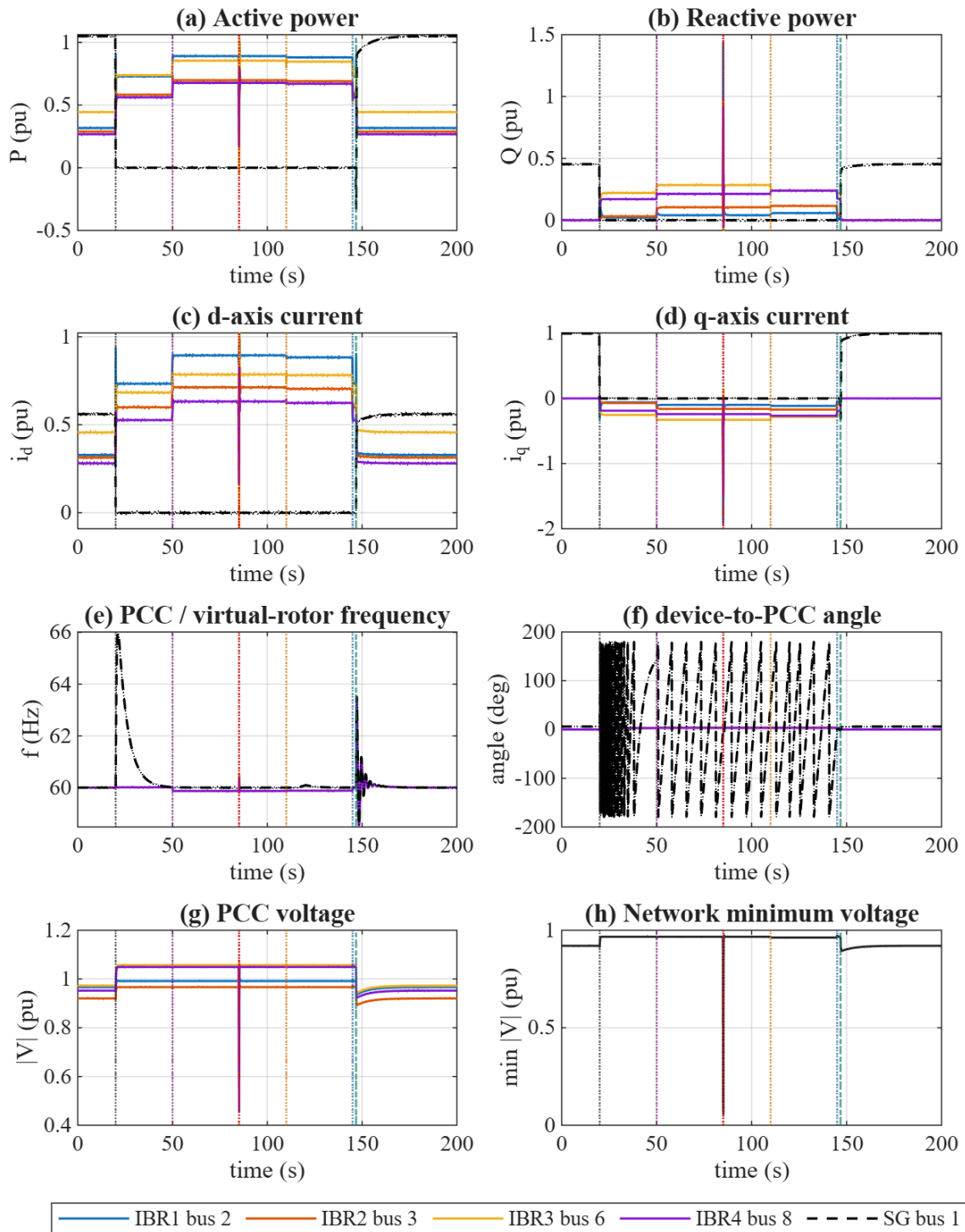
รูปที่ 6: กราฟ P , Q , i_d , i_q , f , มุมเทียบ PCC, แรงดัน PCC และแรงดันต่ำสุดของโครงข่าย เส้นประดำคือ SG เส้นสีทึบคือ raw production result ส่วนเส้นจุดสีเดียวกันคือ ripple แบบ band-limited ที่ seed คงที่เพื่อการนำเสนอเท่านั้น ripple ต่อเนื่องตามเวลาและไม่สร้าง spike ที่ event; เส้นตั้ง/ยอดแหลม ณ เวลา event ที่ยังเห็นอยู่เป็น raw switching transient จริง
