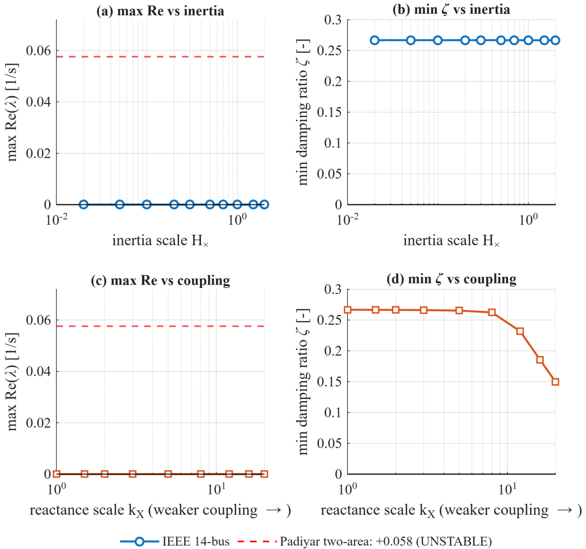
รูปที่ 3: การกวาดเสถียรภาพ SSSA ของระบบ IEEE 14 บัส 1-SG + 4-IBR: spectral abscissa \max \text{Re}(\lambda) และ \zeta ของโหมดหน่วงน้อยสุด เทียบกับการปรับความเฉื่อย (บน, H_X ) และการปรับการคู่ควบ/รีแอคแตนซ์ภายใน (ล่าง, k_X ) ระบบ IEEE 14 บัสเสถียรตลอด ( \max \text{Re} \approx 0 ); เส้นประสีแดงคือค่าอ้างอิงของ Padiyar two-area ที่ \max \text{Re} = +0.058 \text{ s}^{-1} (UNSTABLE, โทโพโลยีสายเชื่อมอ่อนที่ต่างออกไป)
