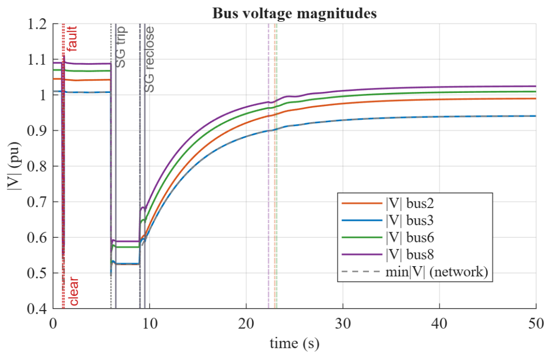
รูปที่ 6: IEEE 14 บัส: ขนาดแรงดันบัสตลอดวงจร ฟอลต์/ปลด/สับกลับ; ค่าต่ำสุดของโครงข่ายฟื้นฟู \approx 0.94 pu
