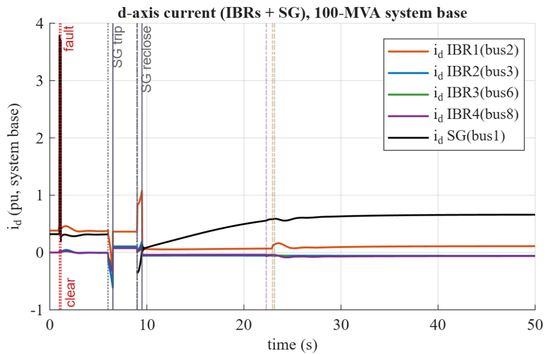
รูปที่ 10: IEEE 14 บัส: กระแสแกน d ( i_d ) ของ IBR; ต่อเนื่องข้ามการสลับ (bumpless)
