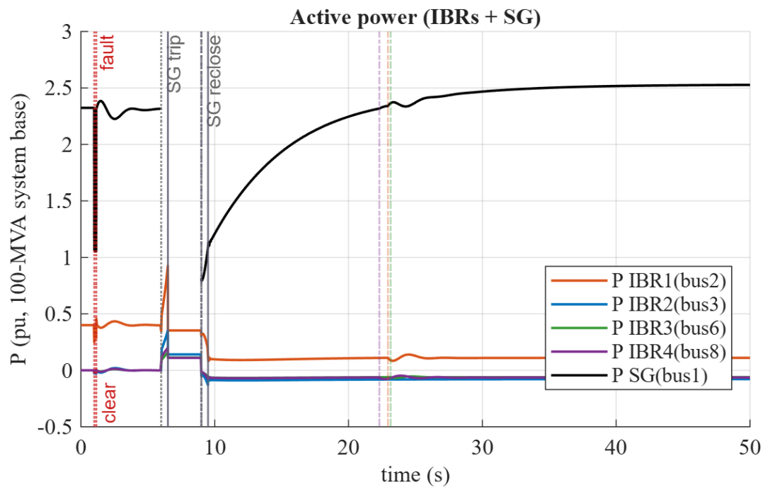
รูปที่ 8: IEEE 14 บัส: กำลังจริงที่ฉีดเข้าระบบ ก่อนเหตุการณ์ SG คง \approx 2.32 pu และ IBR1 (บัส 2) คง \approx 0.40 pu; หลังสับกลับ SG รับกำลังคืน \approx 2.5 pu
