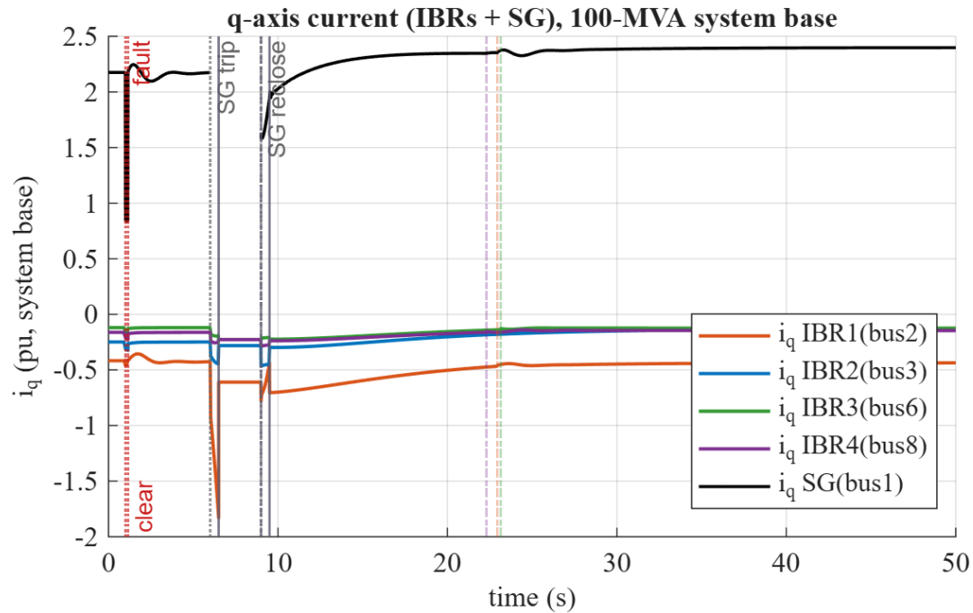
รูปที่ 11: IEEE 14 บัส: กระแสแกน q ( i_q ) ของ IBR; ต่อเนื่องข้ามการสลับ (bumpless)
