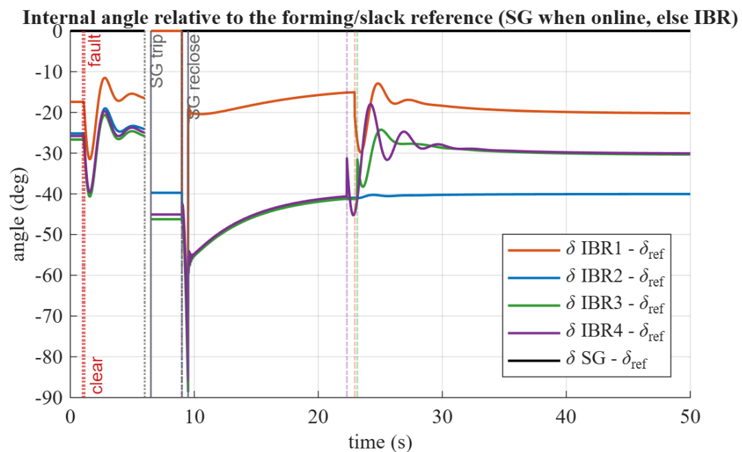
รูปที่ 12: IEEE 14 บัส: มุมของอุปกรณ์ ( \delta ของ SG และ IBR) ตลอดวงจร ปลด/สับกลับ
