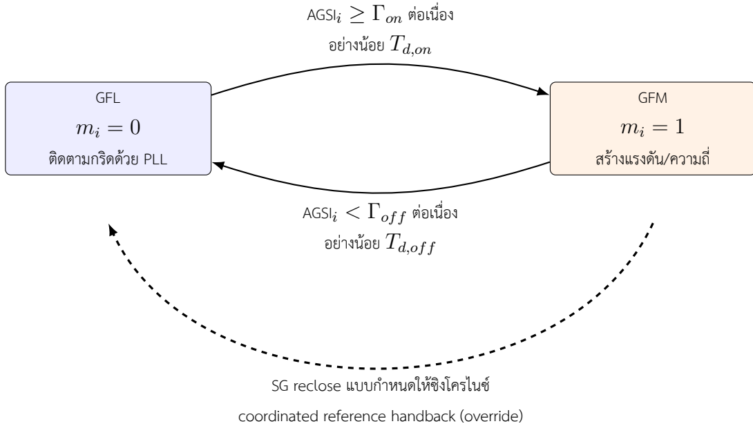
รูปที่ 1: กลไก hybrid state machine ต่อ IBR เส้นทึบคือการสลับอัตโนมัติจาก AGSI++/hysteresis/dwell ส่วนเส้นประคือ coordinated SG-reference handback ซึ่งเป็น event override และไม่ได้อ้างว่าเกิดจากดัชนี
