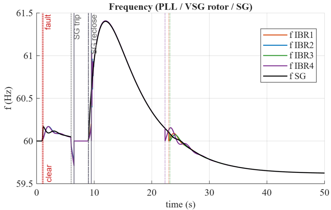
รูปที่ 7: IEEE 14 บัส: ความถี่ของ SG และ IBR (PLL / VSG); การแกว่งหลังปลดขึ้นสูงสุดใกล้ 61.4 Hz แล้วนิ่ง
