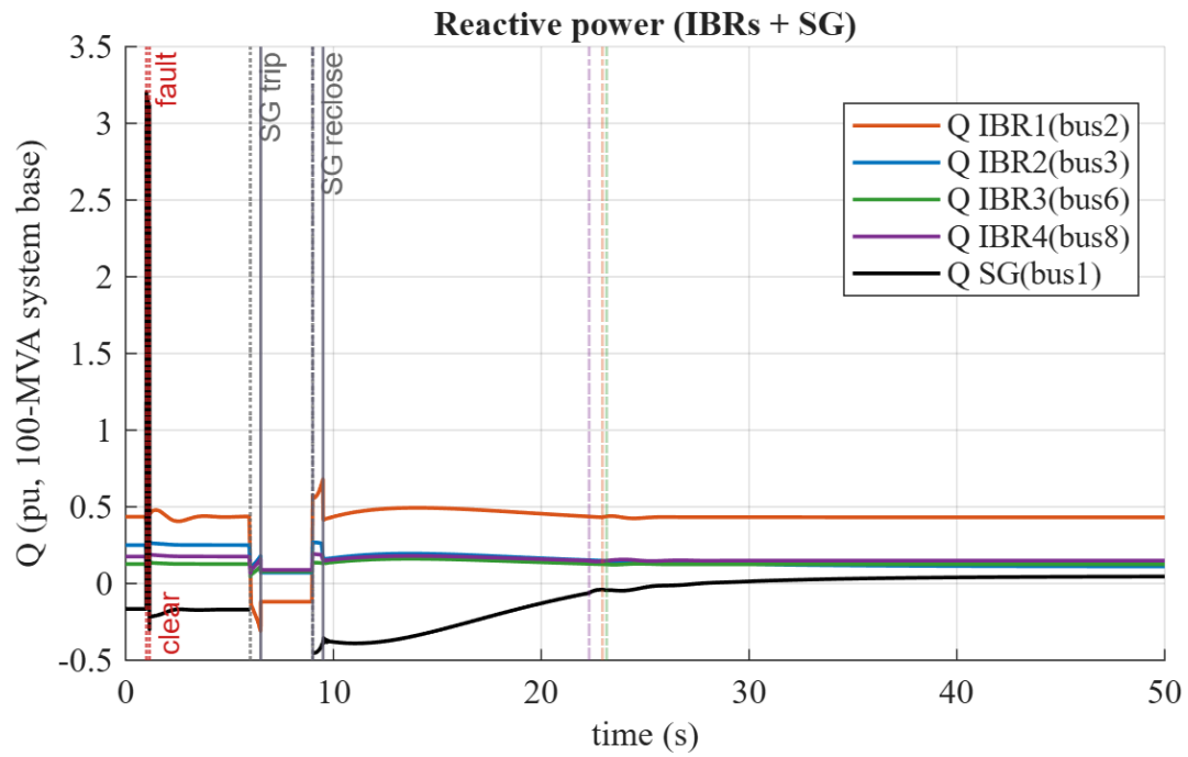
รูปที่ 9: IEEE 14 บัส: กำลังรีแอกทีฟที่ฟีดเข้าระบบตลอดวงจร ปลด/สับกลับ
