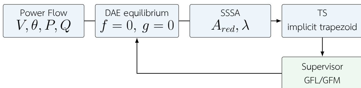
รูปที่ 2: สายงานคำนวณหลักของโครงการ ตั้งแต่ PF ถึงการสลับโหมดใน TS
