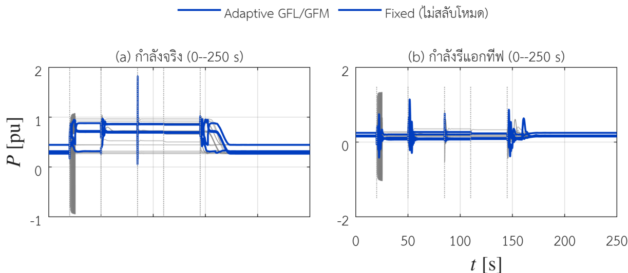
รูปที่ 7: กำลังจริงและกำลังรีแอกทีฟรายคอนเวอร์เตอร์: นโยบายสลับแบบทยอย (น้ำเงิน) เทียบกับแขนงที่ตรงจำนวน GFM คงที่ระหว่างไว้ SG ทุกแขนง (เทา)
