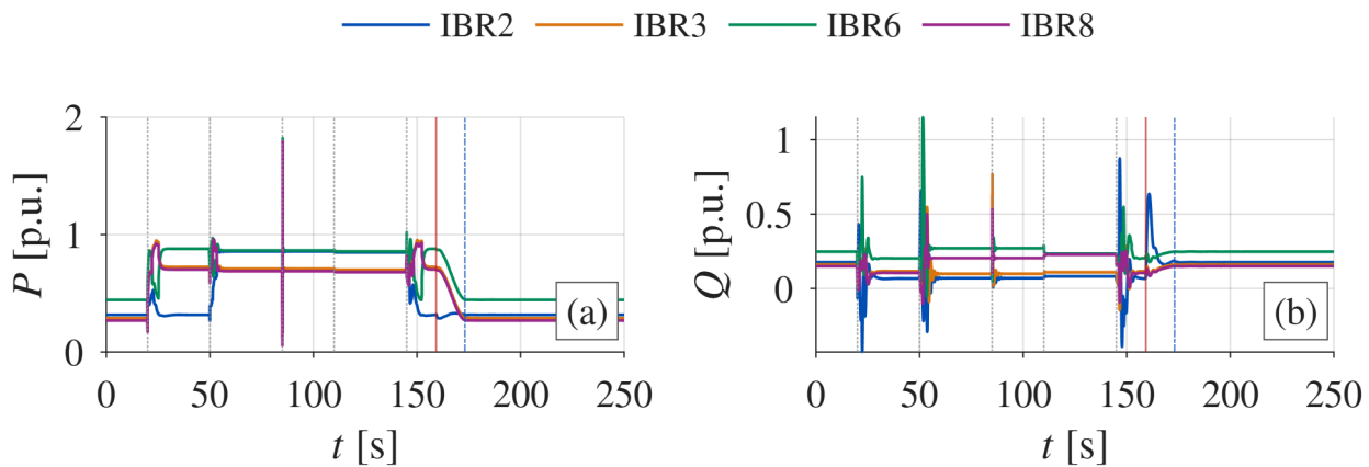
รูปที่ 6: กำลังไฟฟ้าของคอนเวอร์เตอร์ของการสลับโหมด: (a) กำลังไฟฟ้าจริง P (b) กำลังไฟฟ้ารีแอกทีฟ Q เส้นประแนวตั้งคือเวลาเหตุการณ์ที่กรณีศึกษากำหนดไว้ล่วงหน้า เส้นทึบแดงคือเวลาปิดเบรกเกอร์ SG และเส้นประน้ำเงินคือเวลาที่ IBR ตัวสุดท้ายคืนสู่ GFL
