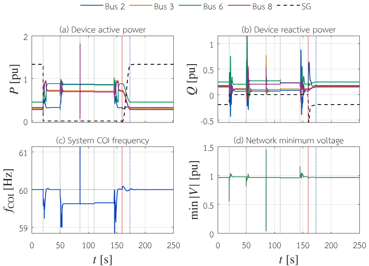
รูปที่ 5: ผลตอบสนองทางไฟฟ้าของแขนงสลับโหมดตลอดลำดับเหตุการณ์ 250 วินาที: กำลังจริงและกำลังรีแอกทีฟรายอุปกรณ์ ความถี่เฉลี่ยระบบ และแรงดันต่ำสุดของเครือข่าย
