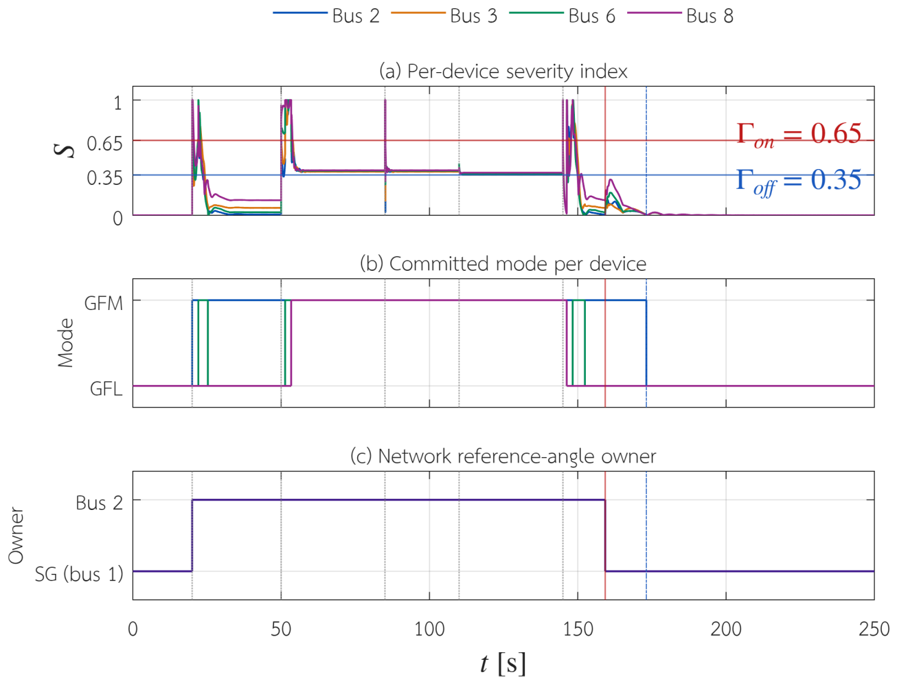
รูปที่ 4: Severity index, สถานะ GFL/GFM และผู้ถือ reference angle ของ adaptive trajectory
