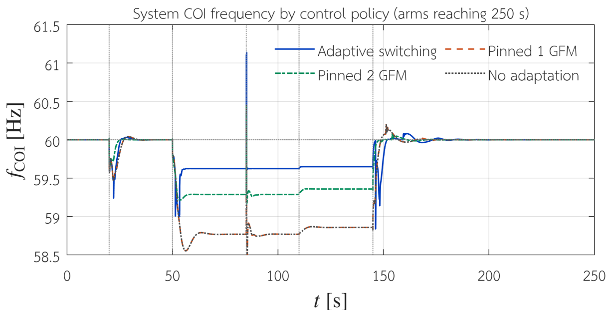
รูปที่ 6: ผลเปรียบเทียบความถี่เฉลี่ยระบบระหว่างนโยบายควบคุมที่ถึงขอบเขตเวลา 250 วินาที
