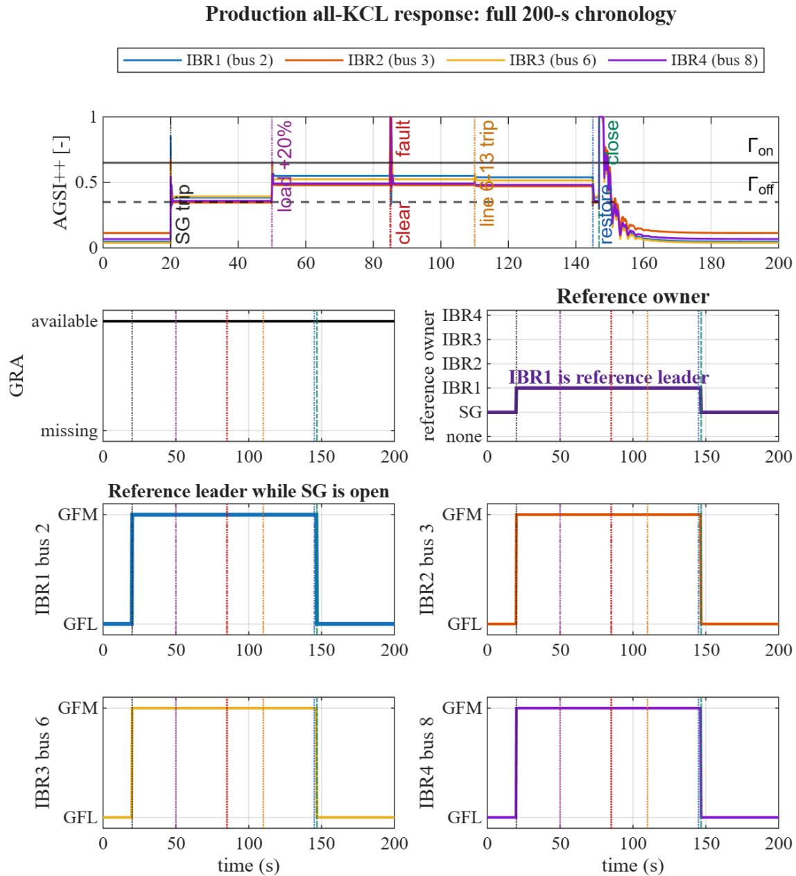
รูปที่ 5: AGSI++ ที่ถูกจำกัดใน [0, 1] , GRA, reference owner และ mode timeline แยก IBR1–IBR4 โหมดเป็น GFL ก่อน 20 s, GFM ช่วง 20–146.825 s และกลับ GFL หลัง 146.825 s
