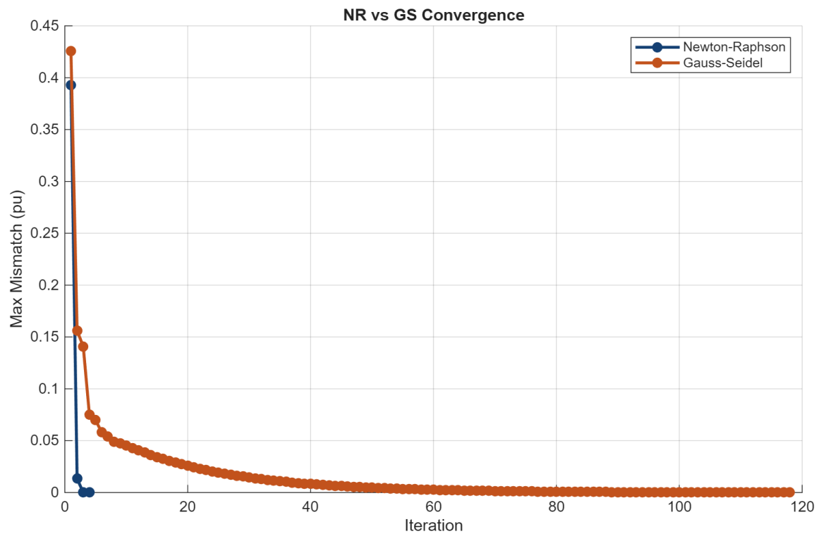
Figure 5: NR vs GS Convergence เปรียบเทียบ – IEEE 30-Bus
