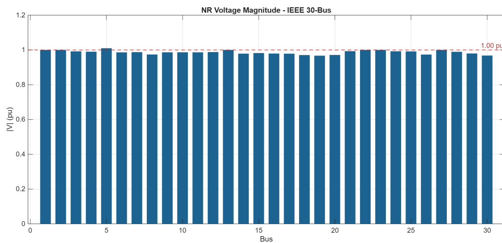
Figure 2: NR Voltage Magnitude ทั่ว Bus – IEEE 30-Bus
