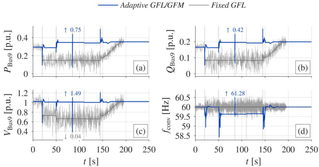
รูปที่ 7 สมรรถนะที่บัส 9 ระหว่างการสลับโหมด Adaptive GFL/GFM (น้ำเงิน) และไม่สลับ Fixed GFL (เทา):
