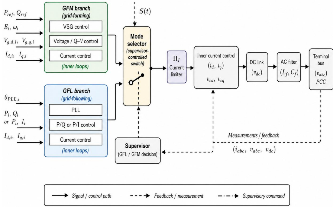
รูปที่ 3 บล็อกไดอะแกรมของ IBR แบบ dual-mode สาขา GFM (VSG, Q-V , วงกระแสชั้นใน) และสาขา GFL (PLL, P/Q , วงกระแสชั้นใน) สร้างกระแสอ้างอิงคนละชุด ตัวเลือกโหมดที่ตัวกำกับสั่งด้วยดัชนีความรุนแรง S(t) ปลอยให้ผ่านได้เพียงสาขาเดียว จากนั้นกระแสอ้างอิงผ่านตัวจำกัด \Pi_I เข้าสู่วงกระแสชั้นใน แล้วต่อไปยัง DC link, ตัวกรอง AC และบัสปลายทางซึ่งทั้งสองโหมดใช้ร่วมกัน เส้นทึบคือทางเดินสัญญาณควบคุม เส้นประคือทางป้อนกลับจากการวัด และเส้นประ-จุดคือคำสั่งจากตัวกำกับ
