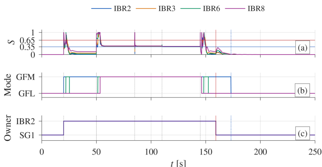
รูปที่ 4 ดัชนีความรุนแรงรายอุปกรณ์ โหมดที่ commit และผู้ถือ reference angle ของแขนงสลัปโหมด: (a)
