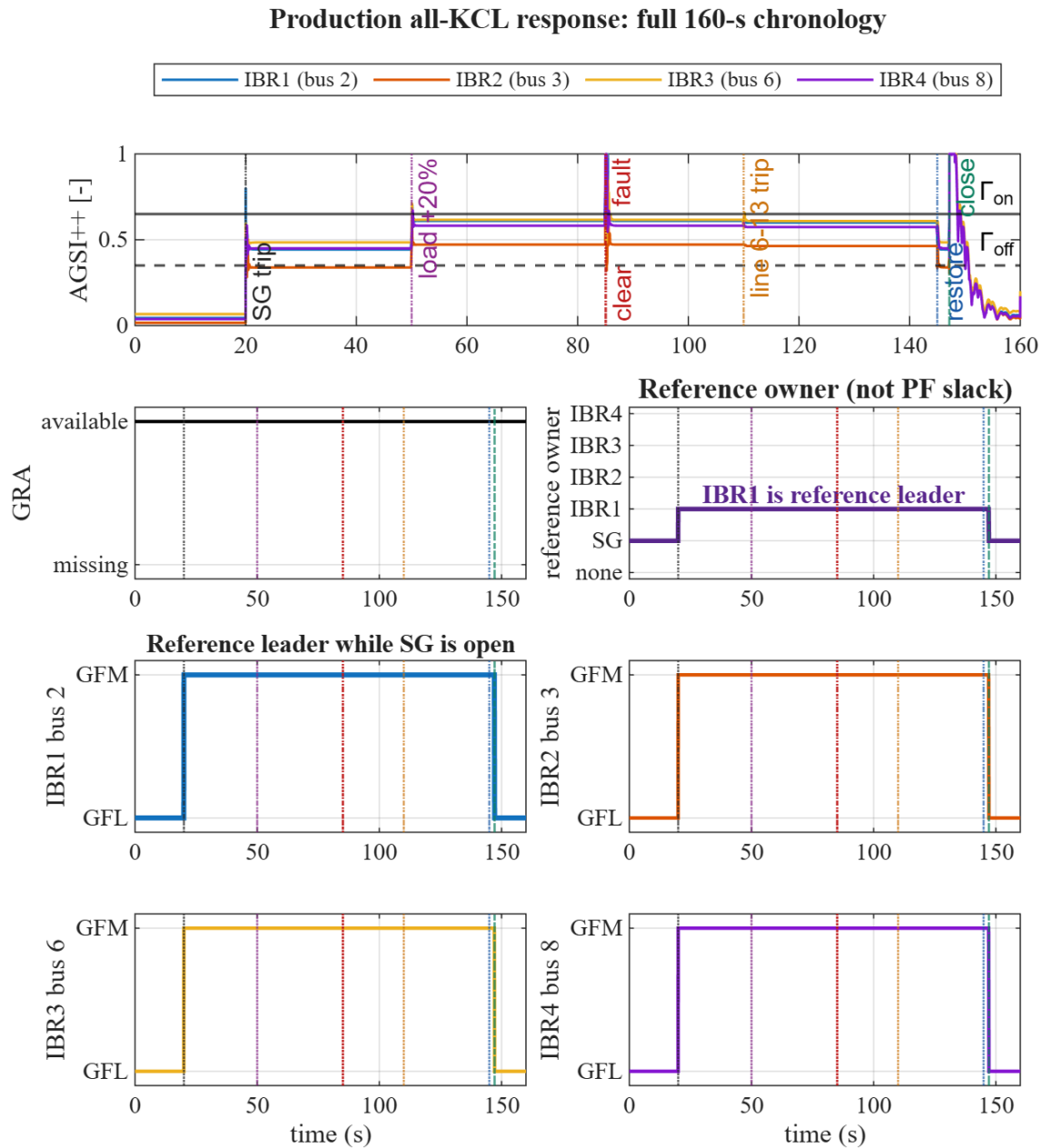
รูปที่ 3: AGSI++ ที่ถูกจำกัดใน [0, 1] , GRA, reference owner และ mode timeline แยก IBR1–IBR4 โหมดเป็น GFL ก่อน 20 s, GFM ช่วง 20–147.175 s และกลับ GFL หลัง 147.175 s
