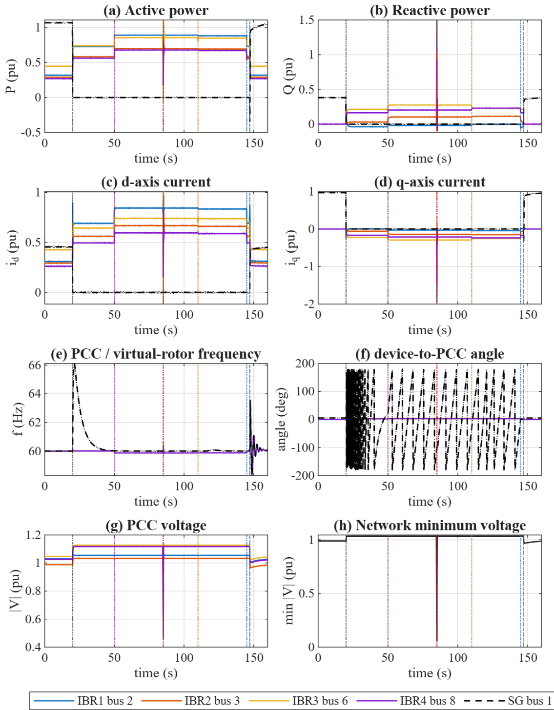
รูปที่ 4: กราฟ P , Q , i_d , i_q , f , มุมเทียบ PCC, แรงดัน PCC และแรงดันต่ำสุดของโครงข่าย เส้นประดำคือ SG เส้นสีทึบคือ raw production result ส่วนเส้นจุดสีเดียวกันคือ ripple แบบ band-limited ที่ seed คงที่เพื่อการนำเสนอเท่านั้น ripple ต่อเนื่องตามเวลาและไม่สร้าง spike ที่ event; เส้นตั้ง/ยอดแหลม ณ เวลา event ที่ยังเห็นอยู่เป็น raw switching transient จริง
