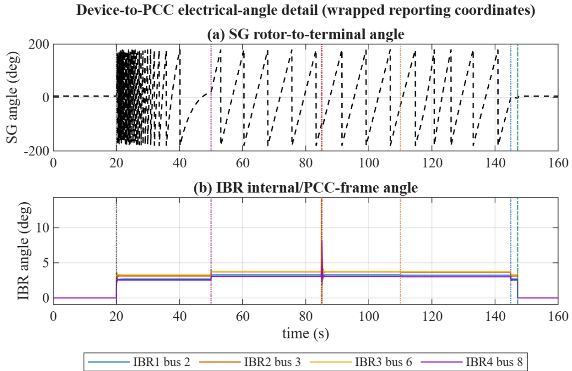
รูปที่ 5: รายละเอียดมุม SG และ IBR เทียบ PCC มุม SG ขณะ offline มี slip จึงแสดงแบบ wrap ในช่วง [-180, 180) องศาไม่ได้ clip state จริง
