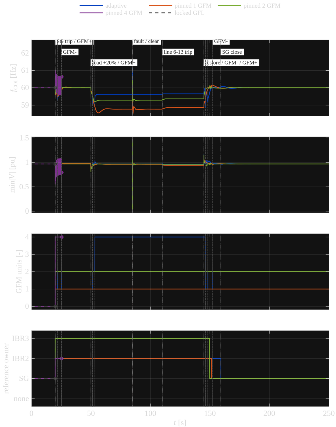
รูปที่ 9: ทำแผนวางทับกันบนขอบฟ้าเต็ม แถวจากบนลงล่าง: ความถี่จุดศูนย์กลางความเฉื่อย แรงดันต่ำสุดของเครือข่าย จำนวนหน่วยที่สร้างแรงดัน และเจ้าของโหมดอ้างอิง ลำดับเหตุการณ์ ถูกระบุเพียงครั้งเดียวบนแถบบนสุดในแถบที่กันไว้เหนือข้อมูล หน้านี้อ่านพฤติกรรม ที่เข้าที่แล้ว: สามแผนที่ รอดแยกออกเป็นสามระดับความถี่ที่ชัดเจน และการเลื่อน ขึ้นเป็นชั้น 1 \rightarrow 2 \rightarrow 4 ของแผนสลับเห็นได้ในแถวที่สาม แผนที่จบก่อนขอบฟ้าหยุด ที่จุดตัวอย่างสุดท้ายของตัวเอง (จุดทึบ) และไม่ถูกต่อเติม ตรึงค่า หรือประมาณค่า นอกช่วงให้ยาวเท่าแผนอื่น ช่วงแกนตั้งทุกแผนมาจากข้อมูลที่อยู่ใน หน้าต่างเวลาที่เราจริง และตัวสร้างรูปจะหยุดถ้ามีจุดใดหลุดออกนอกช่วงนั้น
