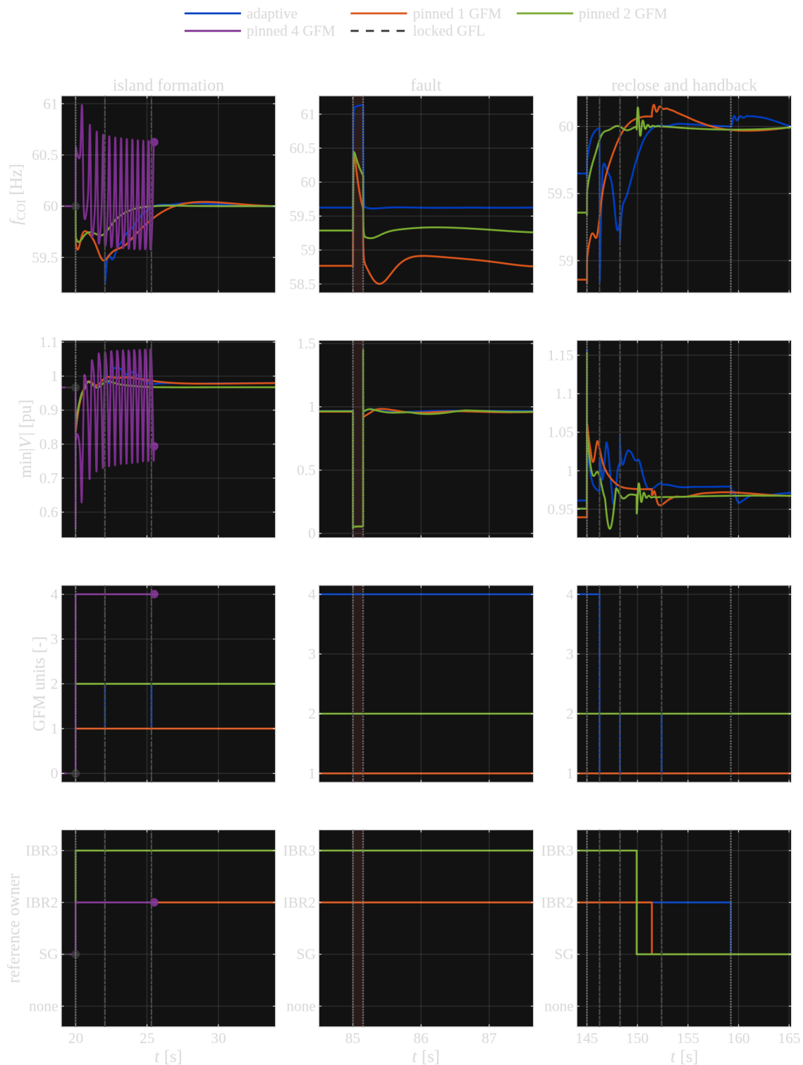
รูปที่ 10: สีแถวเดียวกันบนสามหน้าต่างที่ค่าชั่วคราวแยกแยะได้ ขอบเขตทุกหน้าต่างมาจาก ตารางเหตุการณ์ ช้าย: การสร้างเกาะ ซึ่งแผนที่จริงสี่ตัว แต่เป็นการแกว่งที่โตขึ้นแล้ว ยุติลง กลาง: ฟอลต์ โดยแรงจูงช่วงสั้น 0.150 s แสดงแรงดันต่ำสุดของเครือข่ายที่ทรุด ลงแล้วฟื้นขึ้น ขวา: การต่อกลับและการส่งคืนหน้าที่ แต่ละคอลัมน์ปรับสเกลตามหน้าต่าง ของตัวเอง ซึ่งเป็นสิ่งที่รูปภาพเดียวฉบับก่อนทำไม่ได้
