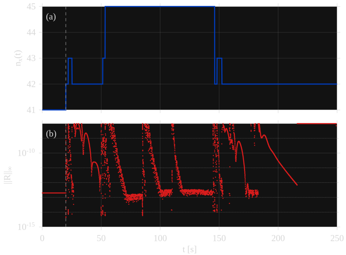
รูปที่ 4: (a) จำนวนสเตตเชิงอนุพันธ์ที่ระบบรวมอินทิเกรตจริง n_x(t) วาดเป็นเส้นขั้นบันได อ่านจากแผนที่สเตตของอุปกรณ์เองที่ทุกจุดตัวอย่างที่ยอมรับ (b) เชวิตลของแต่ละ ขั้นตอนเวลาที่ยอมรับ \|R\|_\infty บนสเกลลอการิทึม เส้นประแนวตั้งสีเทาคือเวลา ที่ SG ถูกตัดออก ทุกจุดเป็นค่าดิบที่ตัวแก้ยอมรับจากวิธี 250 วินาทีของแกนสลับอัตโนมัติ
