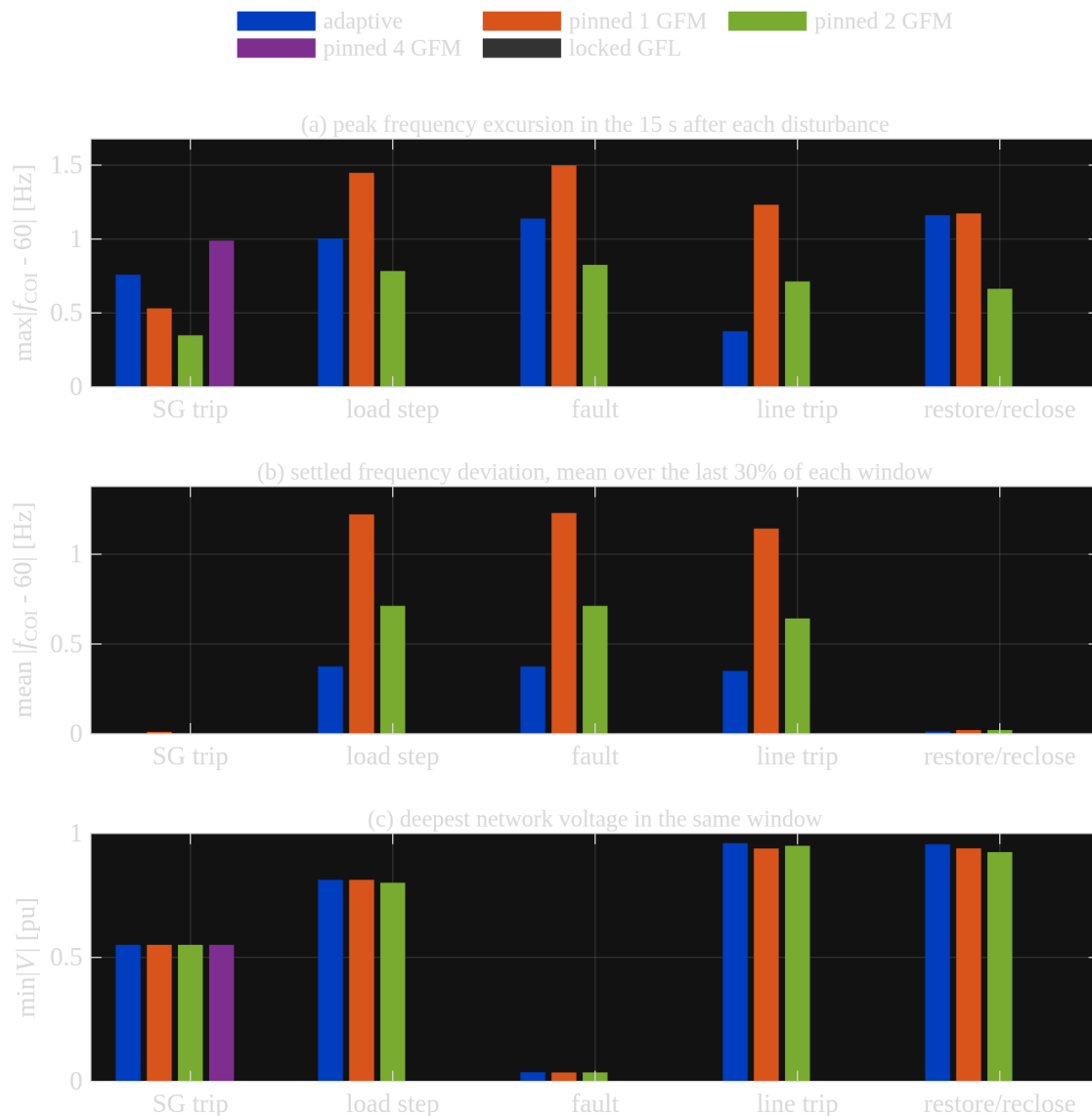
รูปที่ 11: (a) ค่ายอดของการเบี่ยงเบนความถี่ในหน้าต่าง 15 วินาทีหลังแต่ละเหตุการณ์ (b) ค่าที่นิ่งแล้วในหน้าต่างเดียวกัน (c) แรงดันต่ำสุดของเครือข่าย แท่งที่หายไปหมายถึงแกนนั้นไม่ได้เดินเข้าไปในหน้าต่างนั้น ไม่ใช่ค่าศูนย์
