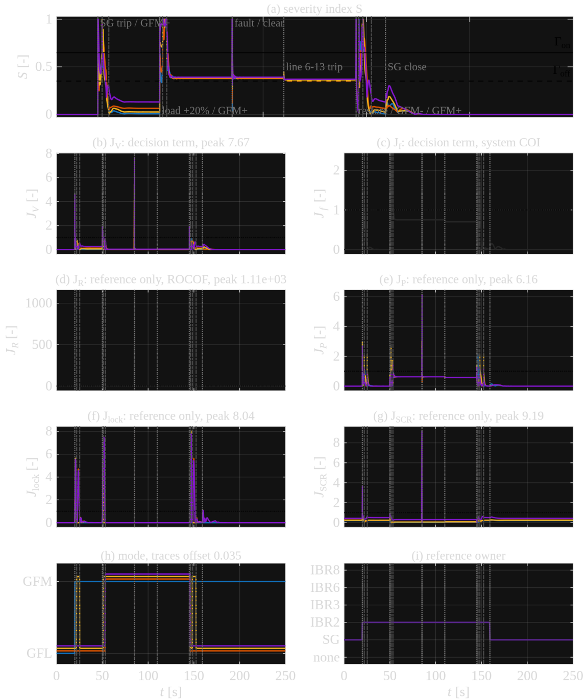
รูปที่ 1: หลักฐาน การตัดสินใจ สลับ โหมด ทุก แผลง ใช้ แกน เวลา เดียวกัน และ เส้น เหตุการณ์ ชุด เดียวกัน (a) ดัชนี ความ รุนแรง S = \text{sat}_{[0,1]}(0.5J_V + 0.5J_f) พร้อมเส้นเกณฑ์ \Gamma_{\text{on}} = 0.65 และ \Gamma_{\text{off}} = 0.35 (b) J_V (c) J_f ของระบบ (d) J_R ของระบบ (e) J_P (f) J_{\text{lock}} (g) J_{\text{SCR}} (h) โหมด GFL/GFM รายตัว (i) เจ้าของมมอ้างอิง เส้นจุด: เหตุการณ์รบกวน เส้นจุด-ขีด: คำสั่งของตัวกำกับ แผลง (a)–(c) เป็นตัวตัดสินใจ แผลง (d)–(g) เป็นดัชนีอ้างอิงที่ไม่เข้าเกณฑ์
