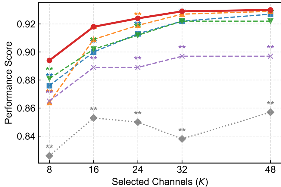
AUC
