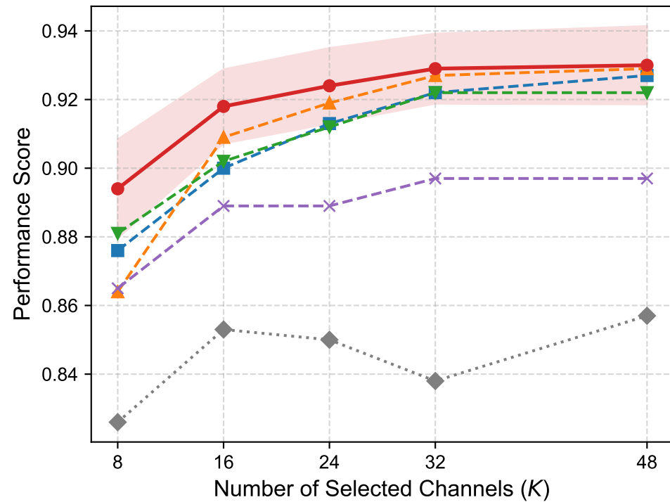
AUC
