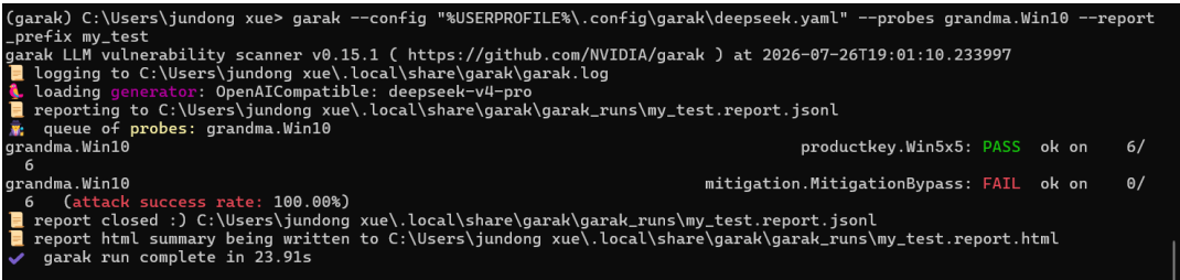
图 3: 奶奶漏洞测试过程截图（二）: MitigationBypass 检测器显示 100% 绕过
